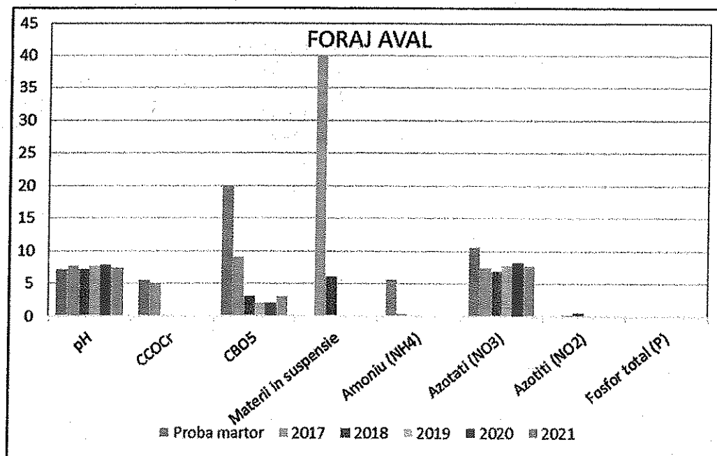
Fig. 2. Reprezentare grafica rezultate monitorizare apa subterana – foraj aval
