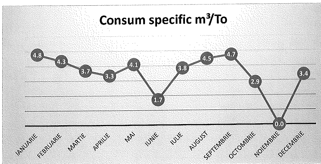
EVOLUTIA CONSUMULUI SPECIFIC DE APA INDUSTRIALA m 3 /t 2021
