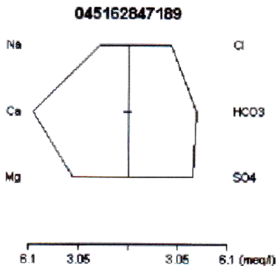
Fig.4.1.3 Diagrama Stiff executate pe baza analizelor chimice ale forajului Poiana F1
