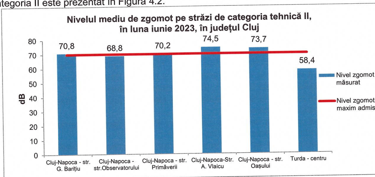
Figura 4.2. Nivelul de zgomot urban pe străzi de categoria II, în județul Cluj, în luna iunie 2023
