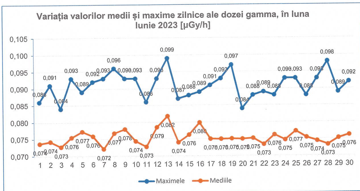
Figura nr. 3.1.1 Variația valorilor medii și maxime zilnice ale debitului dozei gamma în luna iunie 2023
