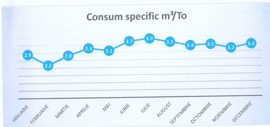
EVOLUTIA CONSUMULUI SPECIFIC DE APA INDUSTRIALA m 3 /t 2023
