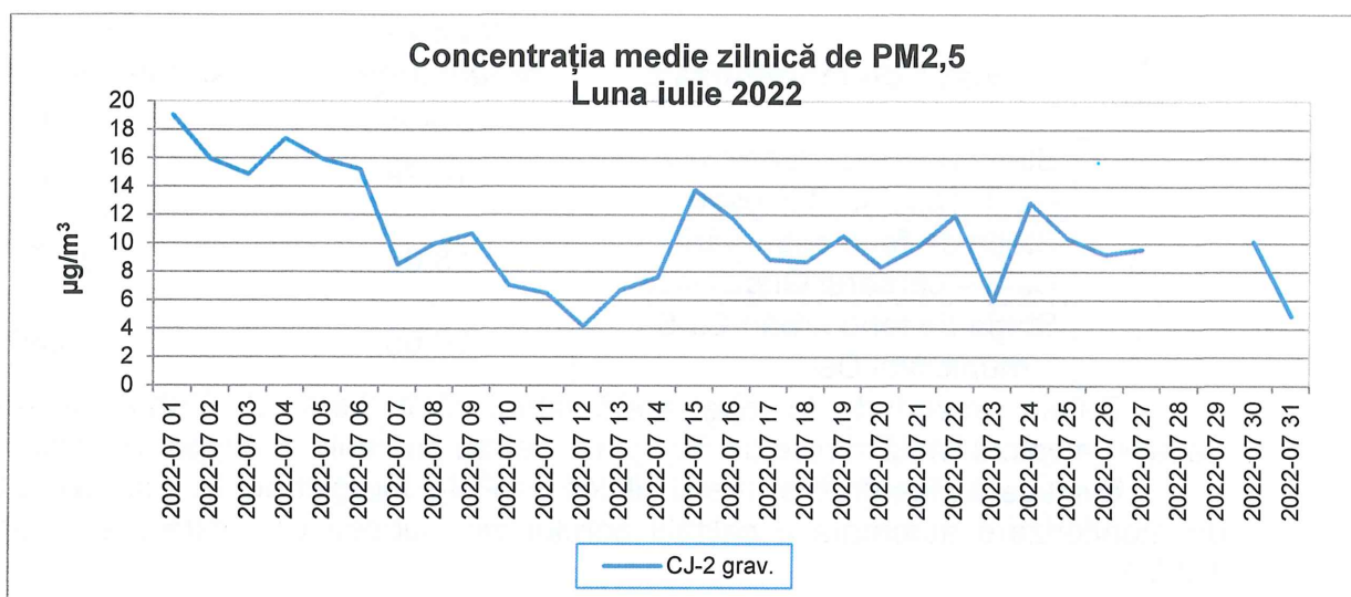
Figura 1.2.5.2. Evoluția concentrației medii zilnice de PM 2,5 , în județul Cluj, în luna Iulie 2022
