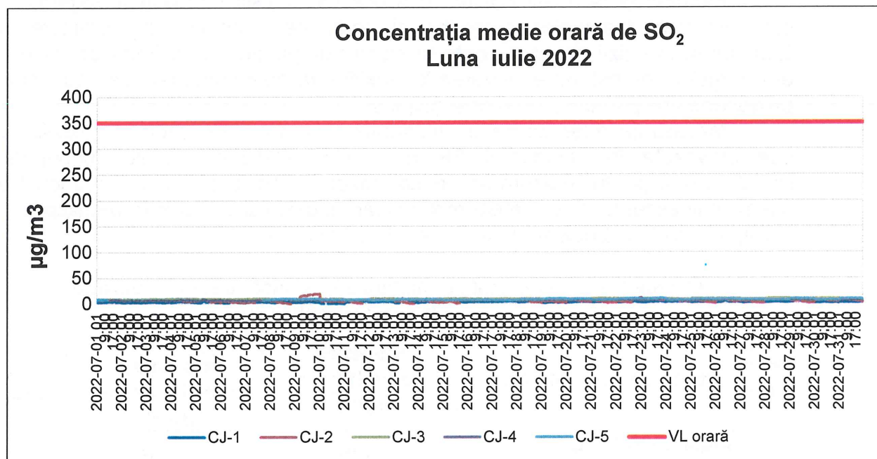
Figura 1.2.1.2. Evoluția concentrației medii orare de SO 2 în județul Cluj în luna Iulie 2022
