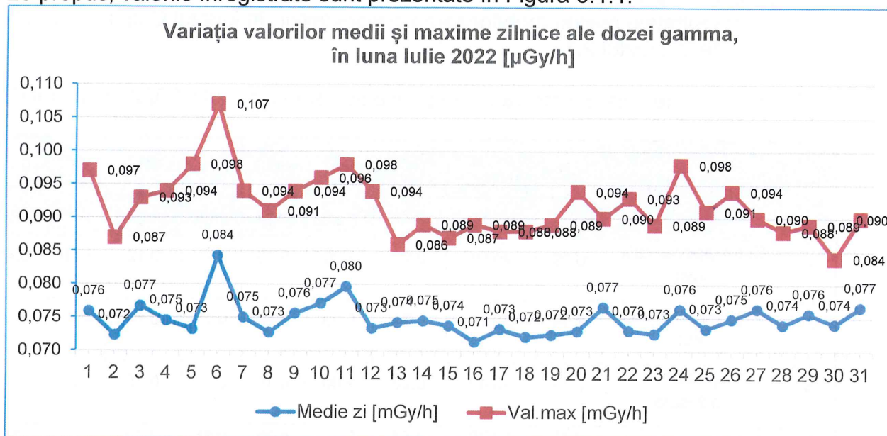
Figura nr. 3.1.1 Variația valorilor medii și maxime zilnice ale debitului dozei gamma în luna Iulie 2022
