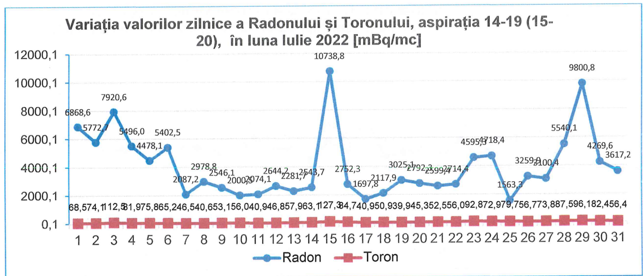
Figura nr. 3.2.2.3 aspirația 14-19
