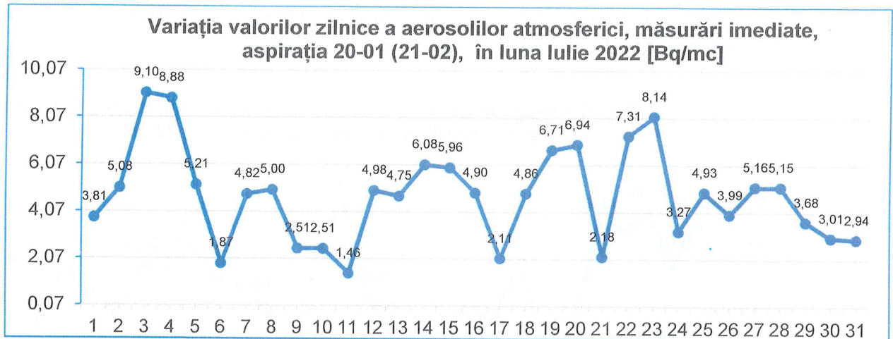
Figura nr. 3.2.1.4 aspirația 21-02
