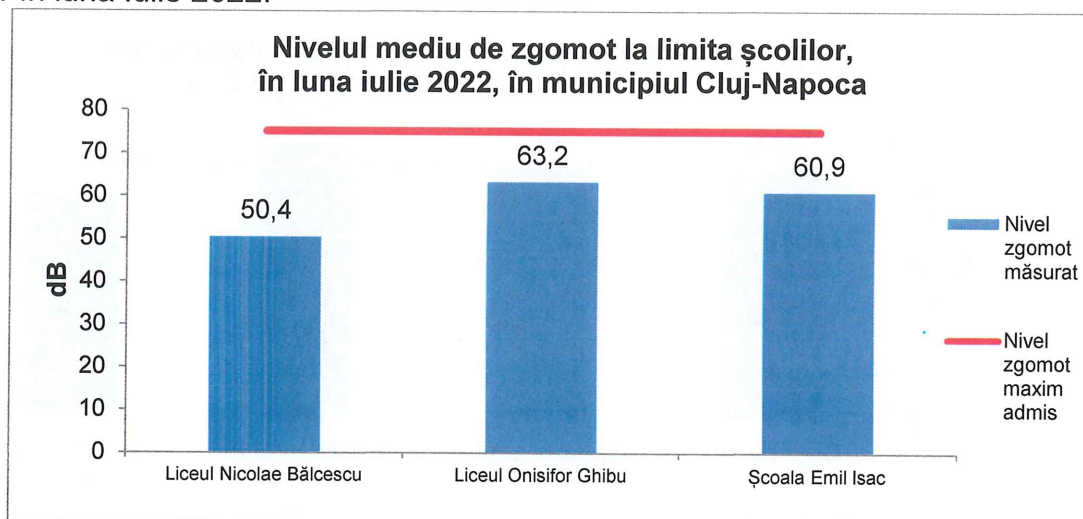
Figura 4.3. Nivelul de zgomot la limita școlilor, în luna Iulie 2022
