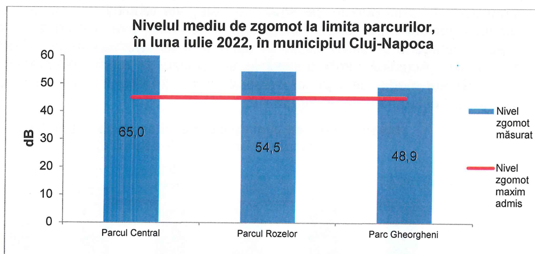
Figura 4.4. Nivelul de zgomot la limita parcurilor, în luna Iulie 2022
