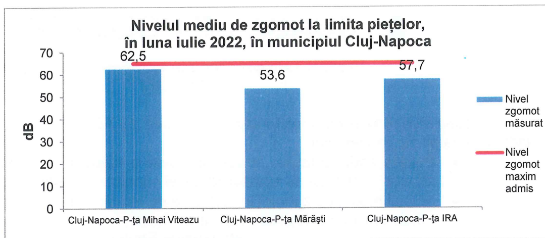
Figura 4.5. Nivelul de zgomot la limita piețelor, în luna Iulie 2022
