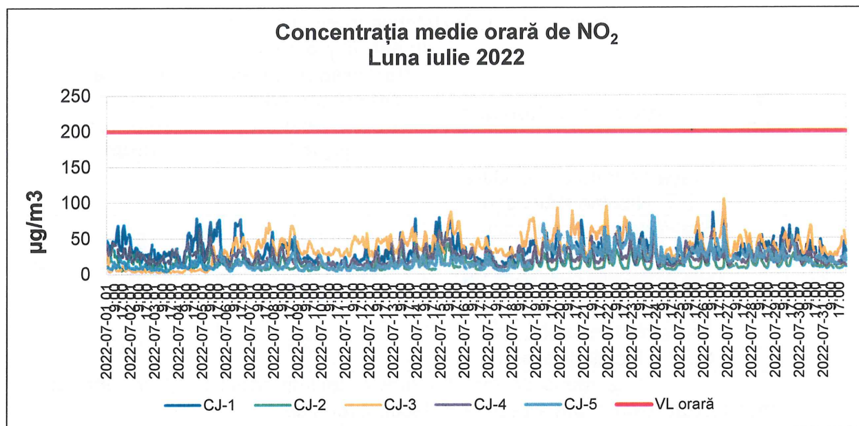
Figura 1.2.2.1. Evoluția concentrațiilor medii orare de \text{NO}_2 în județul Cluj în luna Iulie 2022
