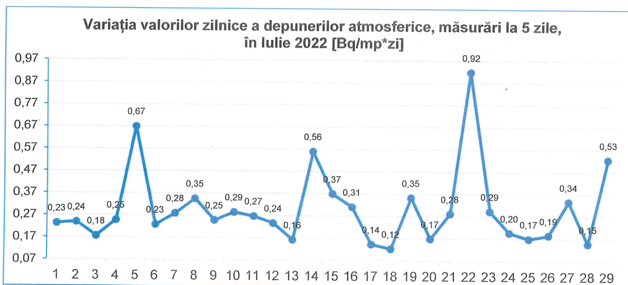
Figura nr. 3.3.2.1 Variația valorilor zilnice a depunerilor atmosferice, măsurări la 5 zile, luna Iulie 2022 [Bq/mp*zi]
