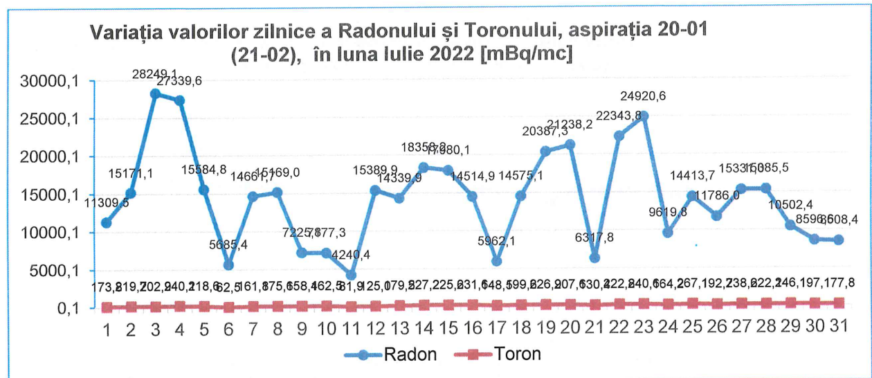
Figura nr. 3.2.2.4 aspirația 20-01
