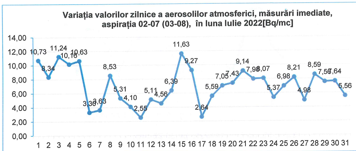
Figura nr. 3.2.1.1 aspirația 3-8
