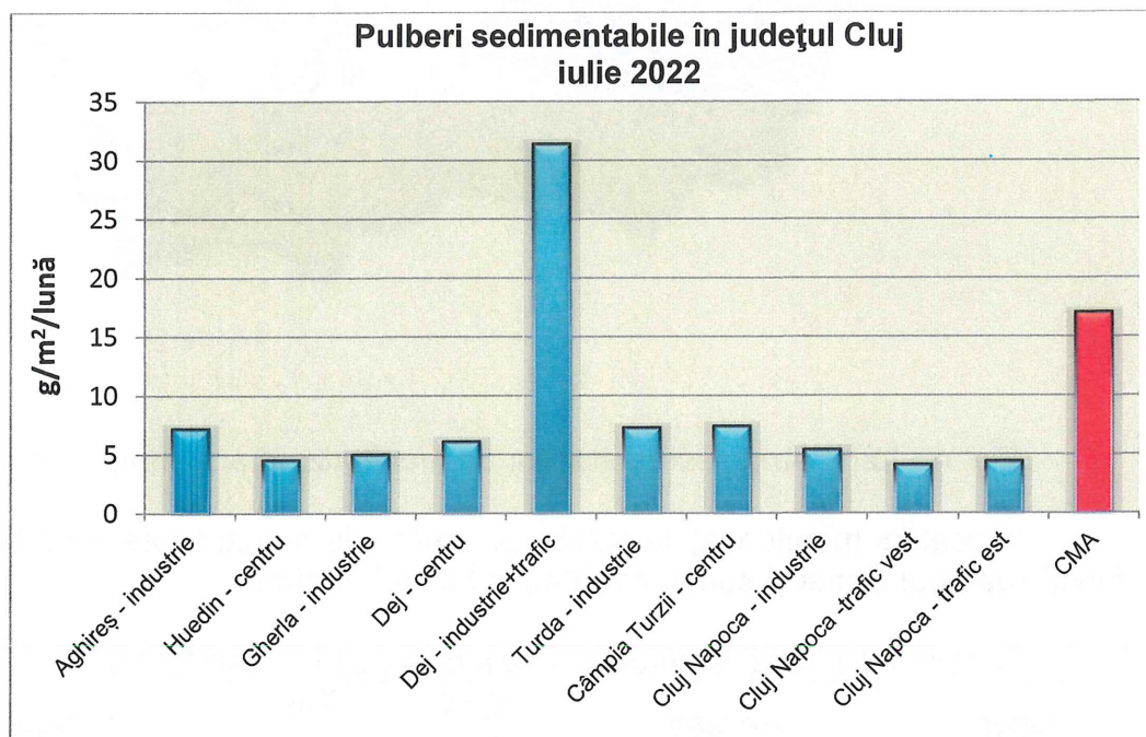
Figura 1.1.4. Evoluția concentrației de pulberi sedimentabile în județul Cluj în luna Iulie 2022
