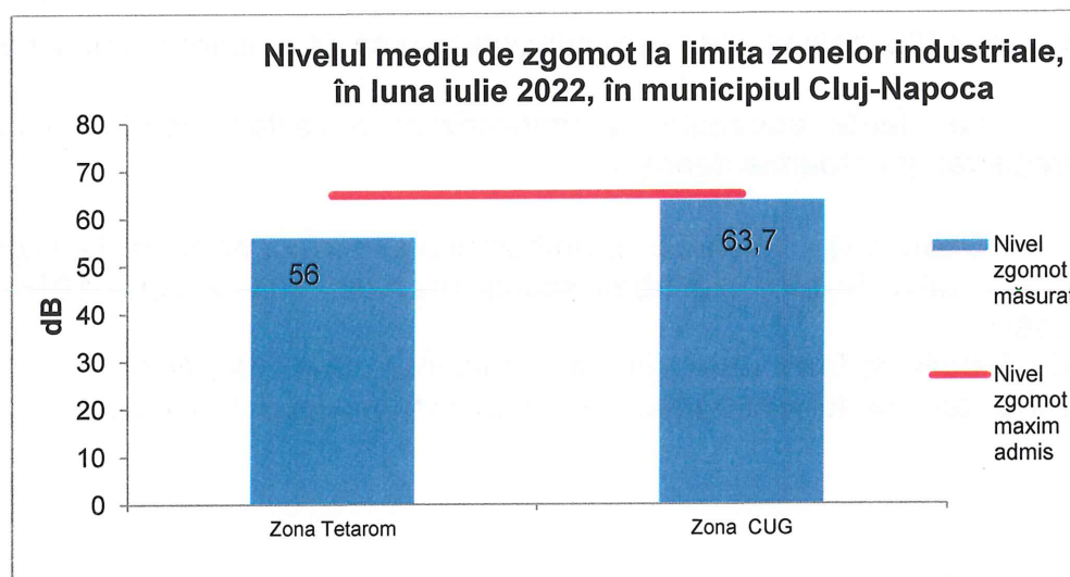
Figura 4.6. Nivelul de zgomot la limita zonelor industriale, în luna Iulie 2022
