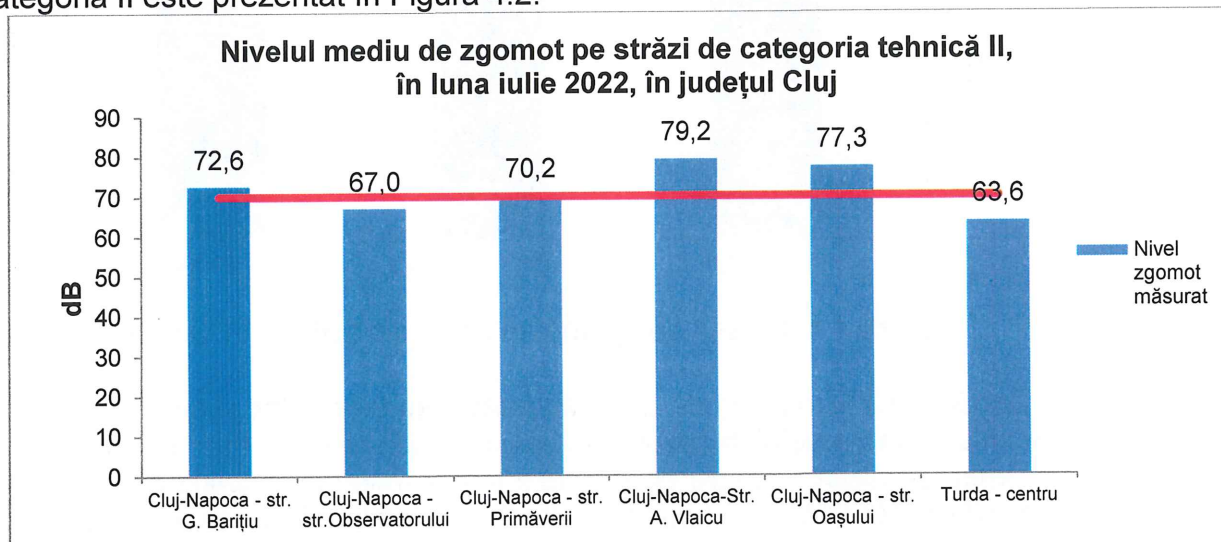
Figura 4.2. Nivelul de zgomot urban pe străzi de categoria II, în județul Cluj, în luna Iulie 2022
