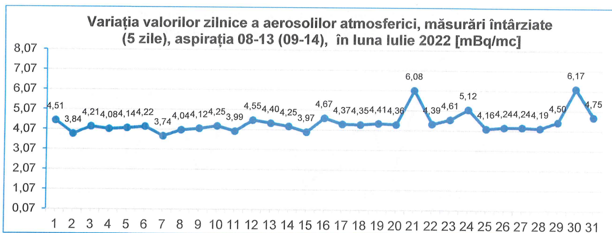
Figura nr. 3.2.3.2 Variația valorilor zilnice a aerosolilor atmosferici, măsurări la 5 zile, aspirația 08-13, în luna Iulie 2022.
