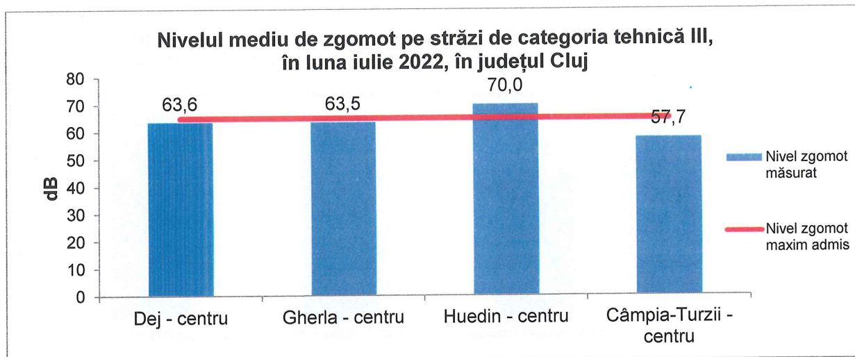
Figura 4.1. Nivelul de zgomot urban pe strazi de categoria III, în județul Cluj, în luna Iulie 2022
