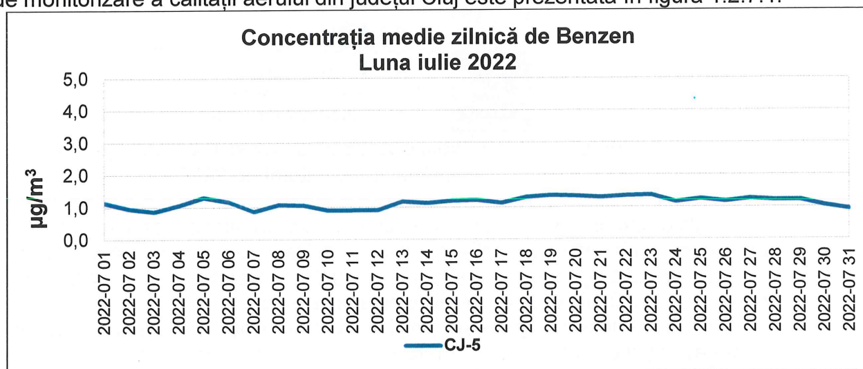
Figura 1.2.7.1. Evoluția concentrației medii de zilnice de benzene în județul Cluj, în luna Iulie 2022
