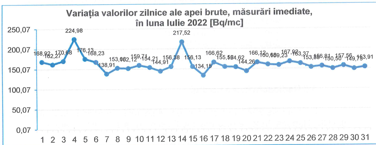
Figura nr. 3.4.1.1.1 Variația valorilor zilnice ale apei brute, măsurări imediate, luna Iulie 2022
