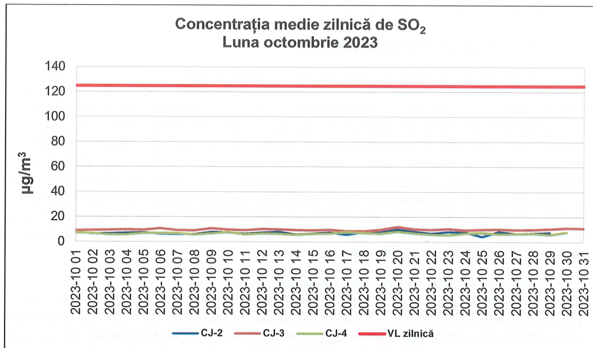
Figura 1.2.1.1. Evoluția concentrației medii zilnice de SO 2 în județul Cluj, în luna octombrie 2023
