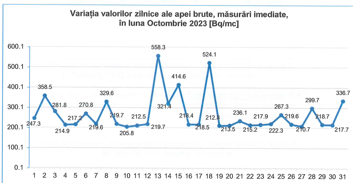
Figura nr. 3.4.1.1.1 Variația valorilor zilnice ale apei brute, măsurări imediate, luna octombrie 2023
