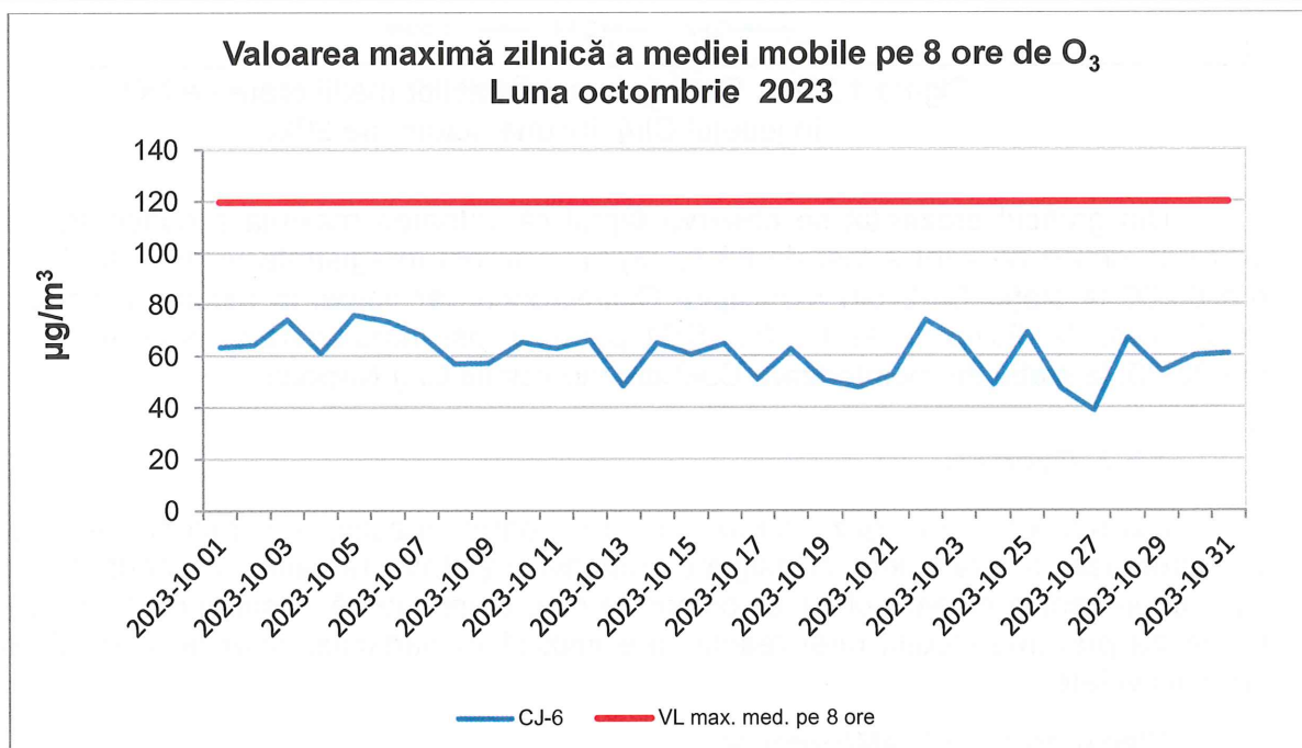
Figura 1.2.3.1. Evoluția maximelor zilnice ale mediilor mobile pe 8 ore de \text{O}_3 , în județul Cluj, în luna octombrie 2023
