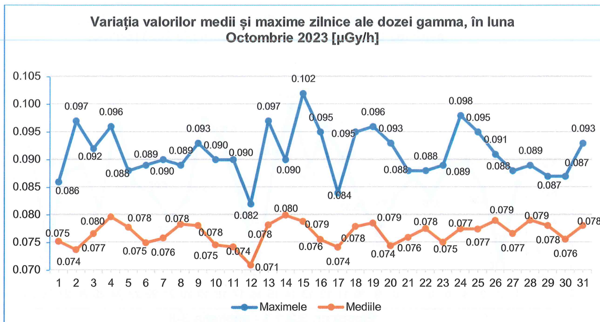
Figura nr. 3.1.1 Variația valorilor medii și maxime zilnice ale debitului dozei gamma, în luna octombrie 2023
