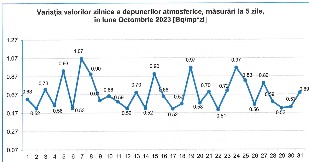
Figura nr. 3.3.2.1 Variația valorilor zilnice a depunerilor atmosferice, măsurări la 5 zile, luna octombrie 2023 [Bq/mp*zi]
