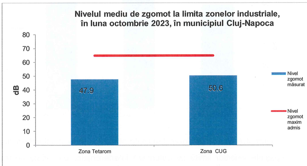
Figura 4.6. Nivelul de zgomot la limita zonelor industriale, în luna octombrie 2023
