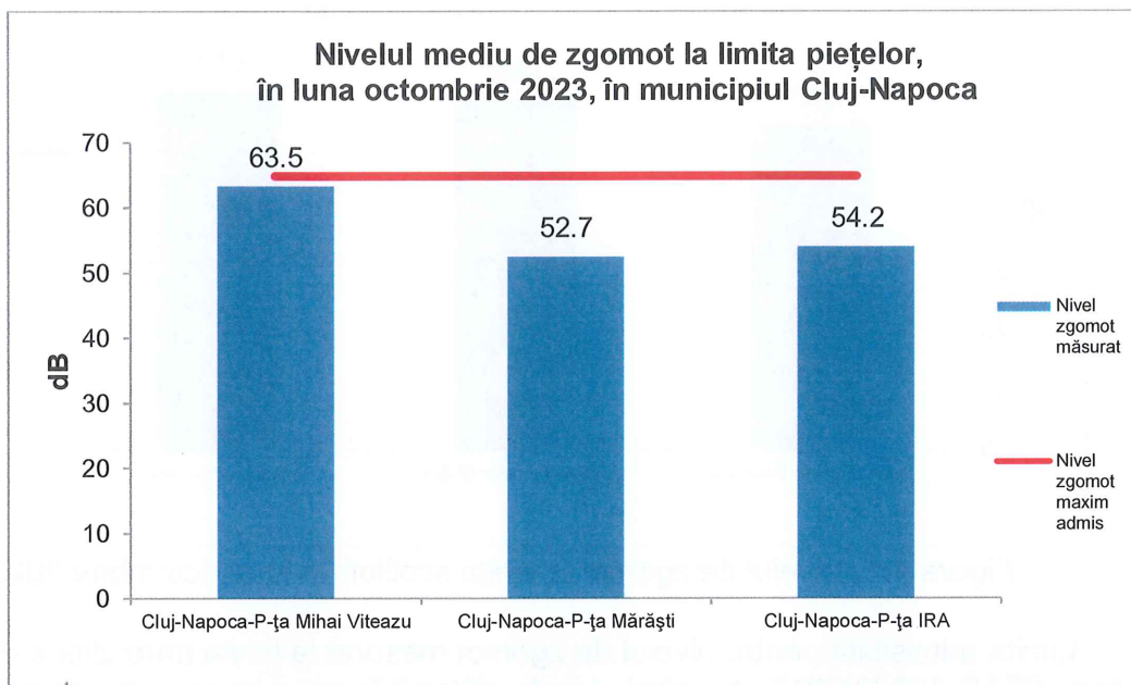
Figura 4.5. Nivelul de zgomot la limita piețelor, în luna octombrie 2023
