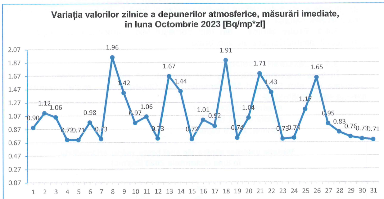
Figura nr. 3.3.1.1 Variația valorilor zilnice a depunerilor atmosferice, măsurări imediate, luna octombrie 2023 [Bq/mp*zi]
