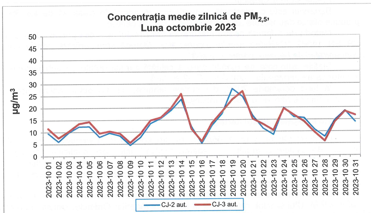
Figura 1.2.5.2. Evoluția concentrației medii zilnice de PM 2,5 , în județul Cluj, în luna octombrie 2023
