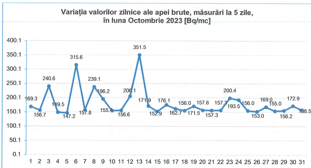
Figura nr. 3.4.1.2.1 Variația valorilor zilnice ale apei brute, măsurări la 5 zile, luna octombrie 2023
