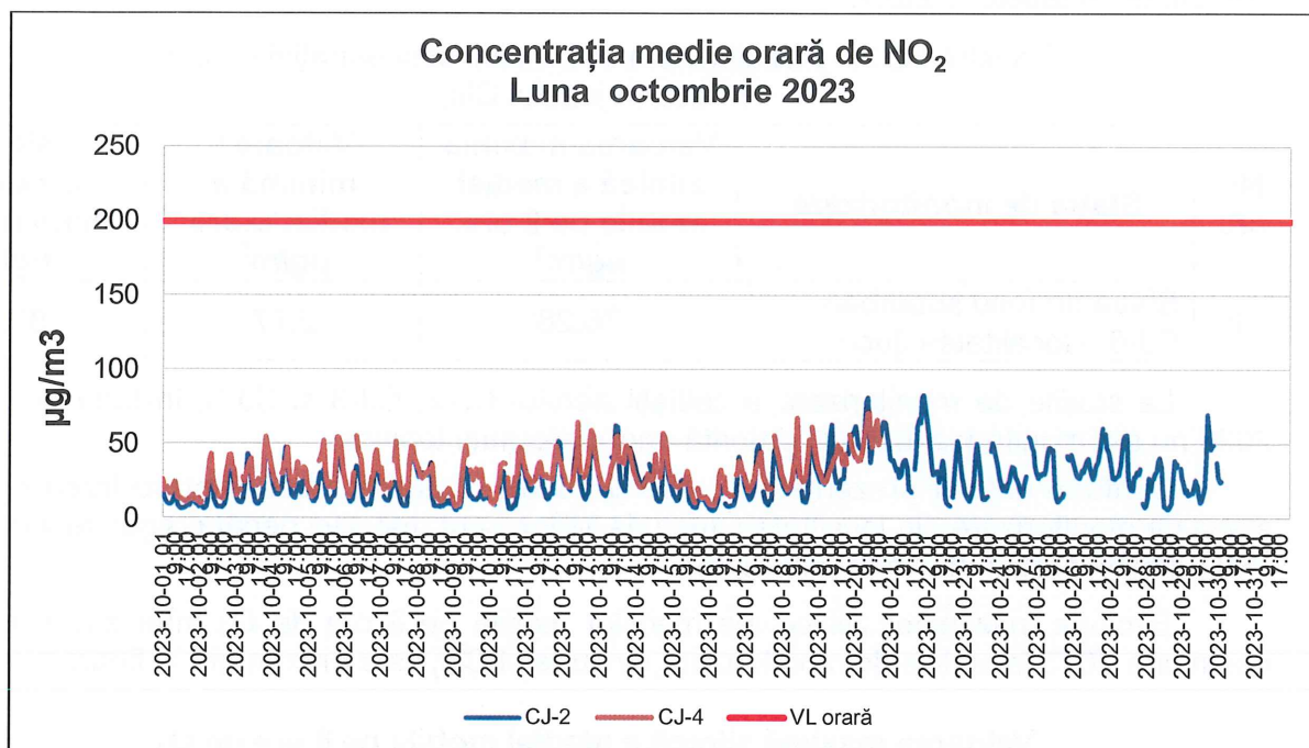
Figura 1.2.2.1. Evoluția concentrațiilor medii orare de \text{NO}_2 în județul Cluj, în luna octombrie 2023
