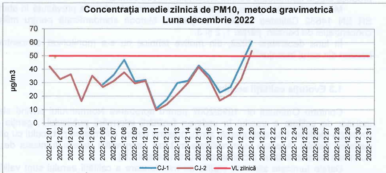
Figura 1.2.5.1. Evoluția concentrației medii zilnice de \text{PM}_{10} , în județul Cluj, în luna Decembrie 2022
