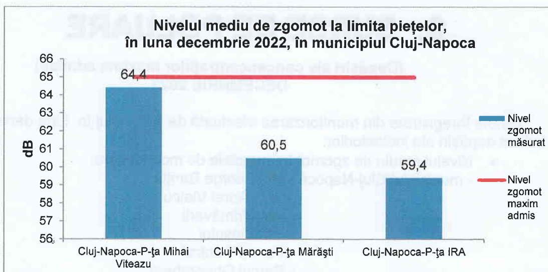
Figura 4.5. Nivelul de zgomot la limita piețelor, în luna decembrie 2022
