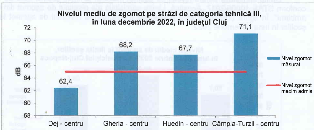
Figura 4.1. Nivelul de zgomot urban pe străzi de categoria III, în județul Cluj, în luna decembrie 2022
