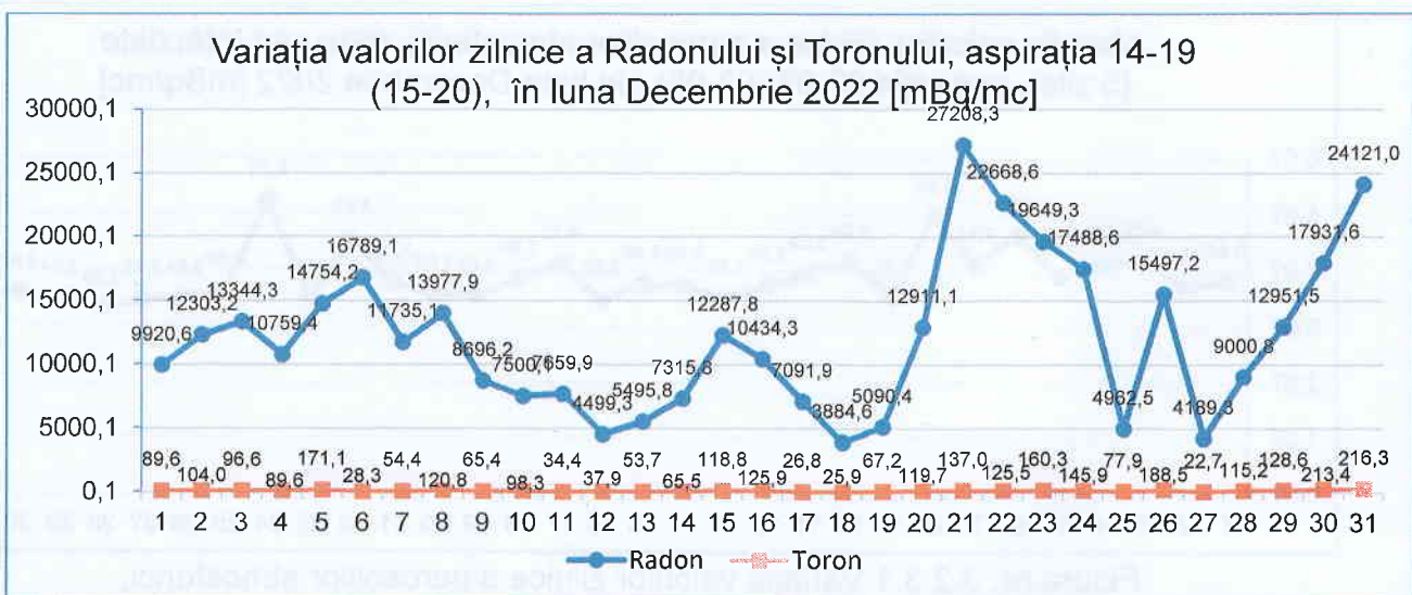
Figura nr. 3.2.2.3 aspirația 14-19
