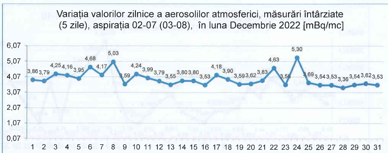
Figura nr. 3.2.3.1 Variația valorilor zilnice a aerosolilor atmosferici, măsurări la 5 zile, aspirația 02-07, în luna Decembrie 2022
