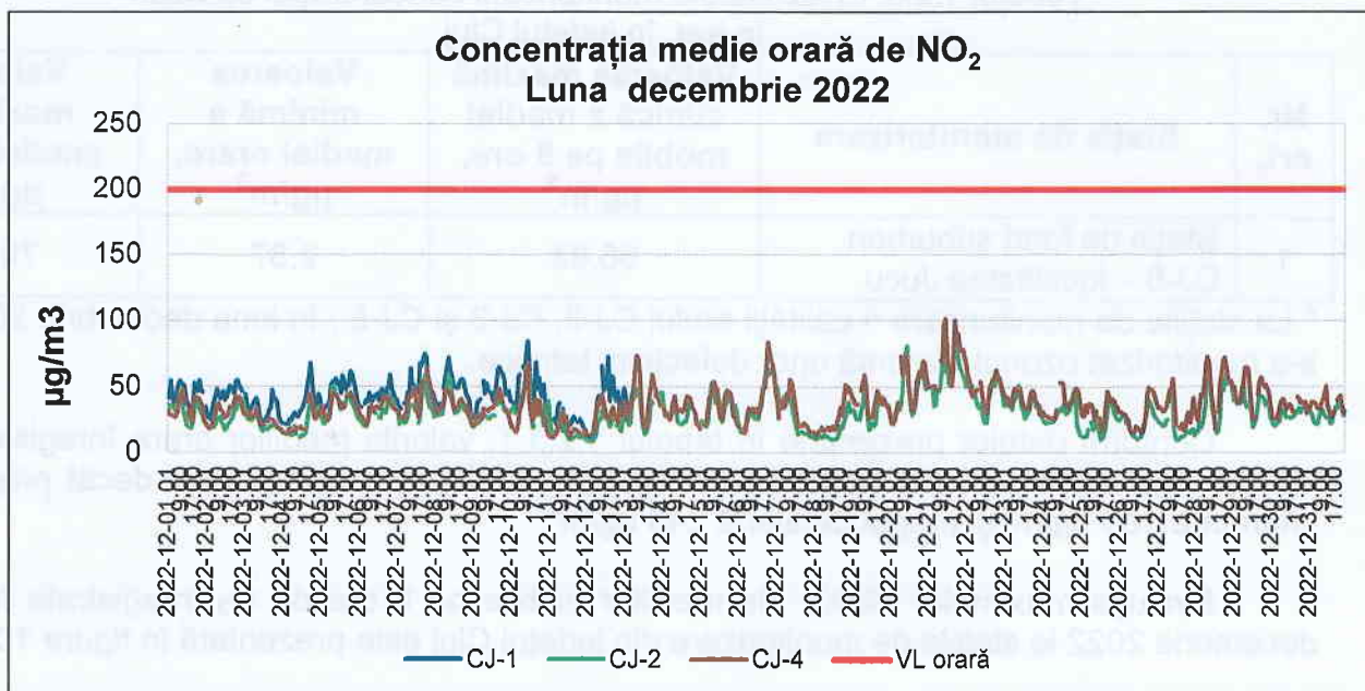
Figura 1.2.2.1. Evoluția concentrațiilor medii orare de \text{NO}_2 în județul Cluj în luna decembrie 2022
