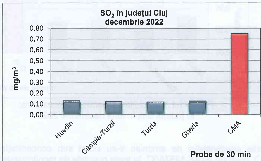
Figura 1.1.3. Evoluția concentrației de dioxid de sulf în județul Cluj în luna decembrie 2022
