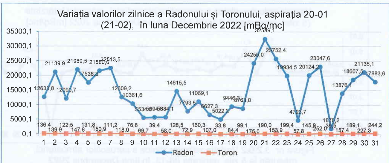
Figura nr. 3.2.2.4 aspirația 20-01
