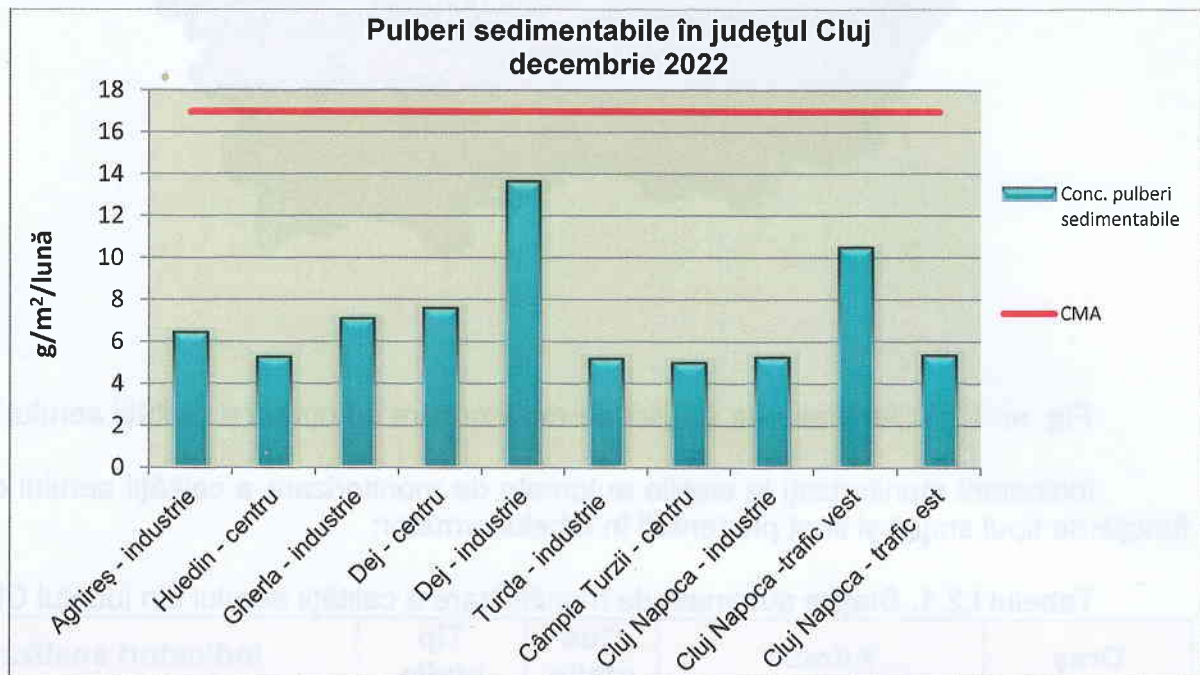
Figura 1.1.4. Evoluția concentrației de pulberi sedimentabile în județul Cluj în luna decembrie 2022
