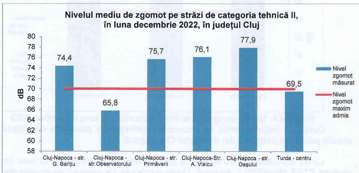
Figura 4.2. Nivelul de zgomot urban pe străzi de categoria II, în județul Cluj, în luna decembrie 2022
