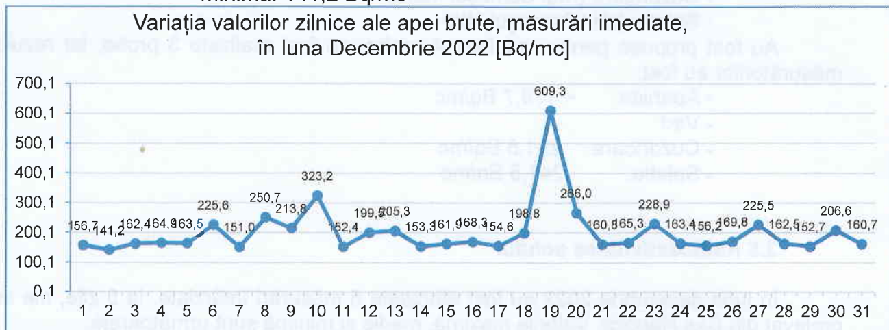
Figura nr. 3.4.1.1.1 Variația valorilor zilnice ale apei brute, măsurări imediate, luna Decembrie 2022
