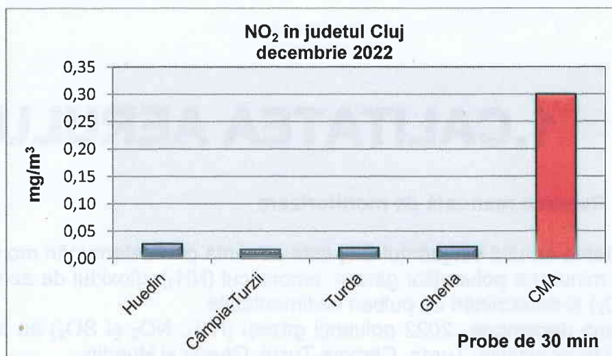
Figura 1.1.2. Evoluția concentrației de dioxid de azot în județul Cluj în luna decembrie 2022
