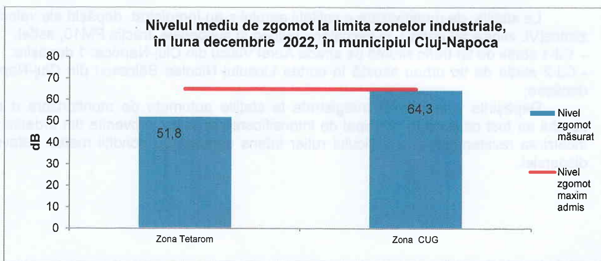
Figura 4.6. Nivelul de zgomot la limita zonelor industriale, în luna decembrie 2022
