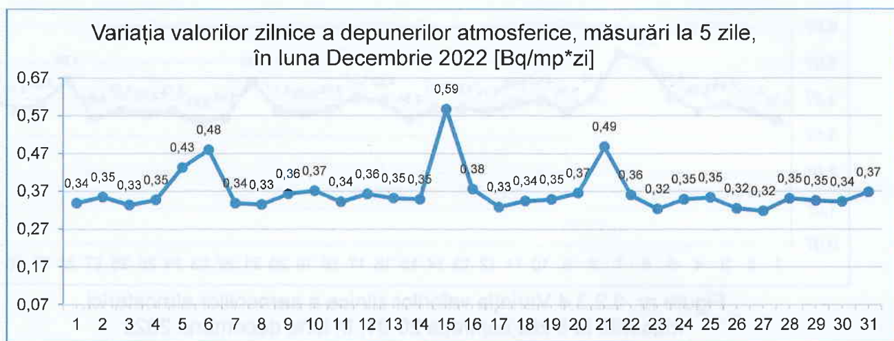
Figura nr. 3.3.2.1 Variația valorilor zilnice a depunerilor atmosferice, măsurări la 5 zile, luna decembrie 2022 [Bq/mp*zi]
