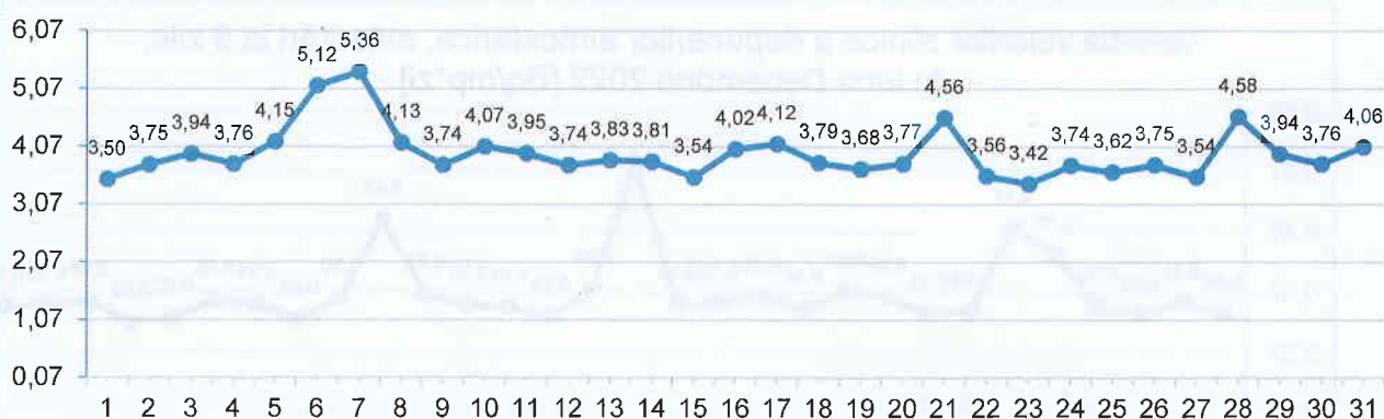
Figura nr. 3.2.3.4 Variația valorilor zilnice a aerosolilor atmosferici, măsurări la 5 zile, aspirația 20-01, în luna decembrie 2022
