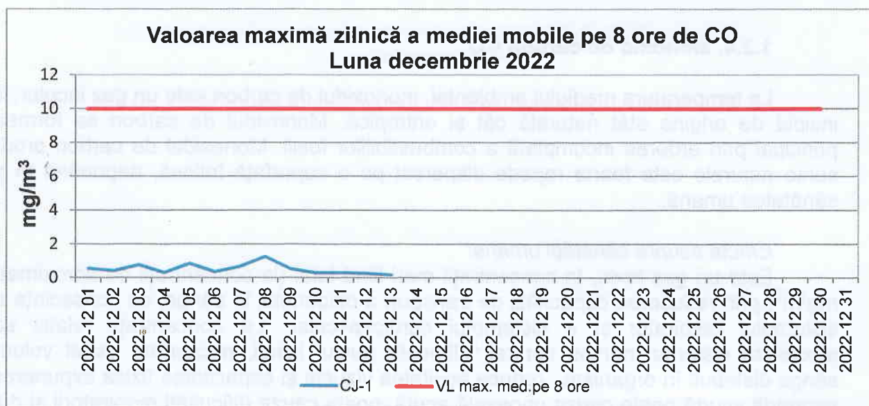
Figura 1.2.4.1. Evoluția concentrațiilor maxime zilnice a mediilor mobile pe 8 ore de CO, în județul Cluj, în luna decembrie 2022
