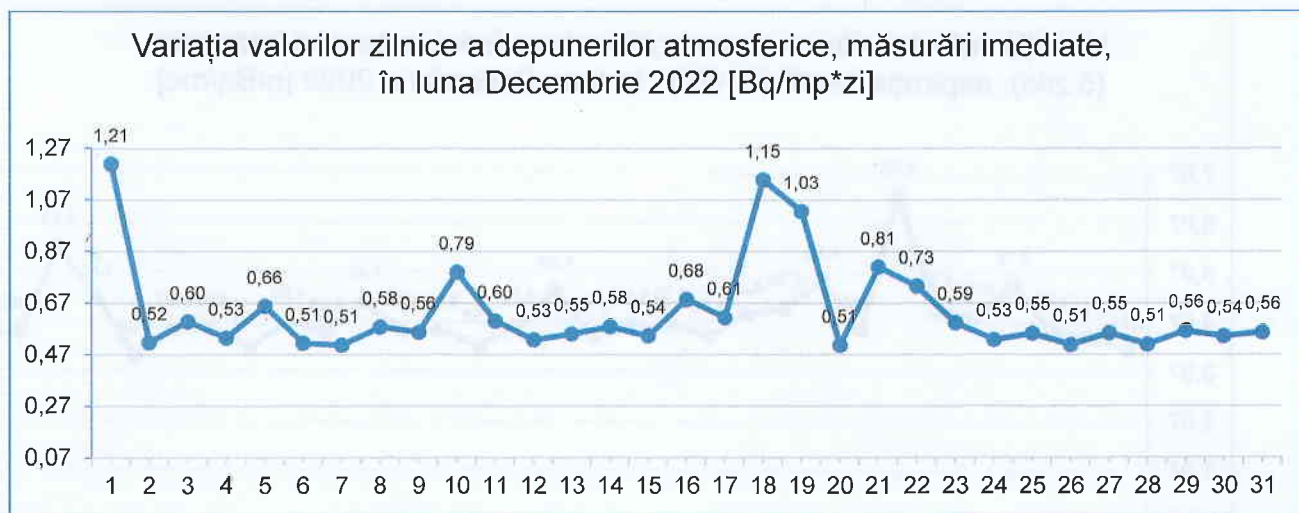
Figura nr. 3.3.1.1 Variația valorilor zilnice a depunerilor atmosferice, măsurări imediate, luna decembrie 2022 [Bq/mp*zi]
