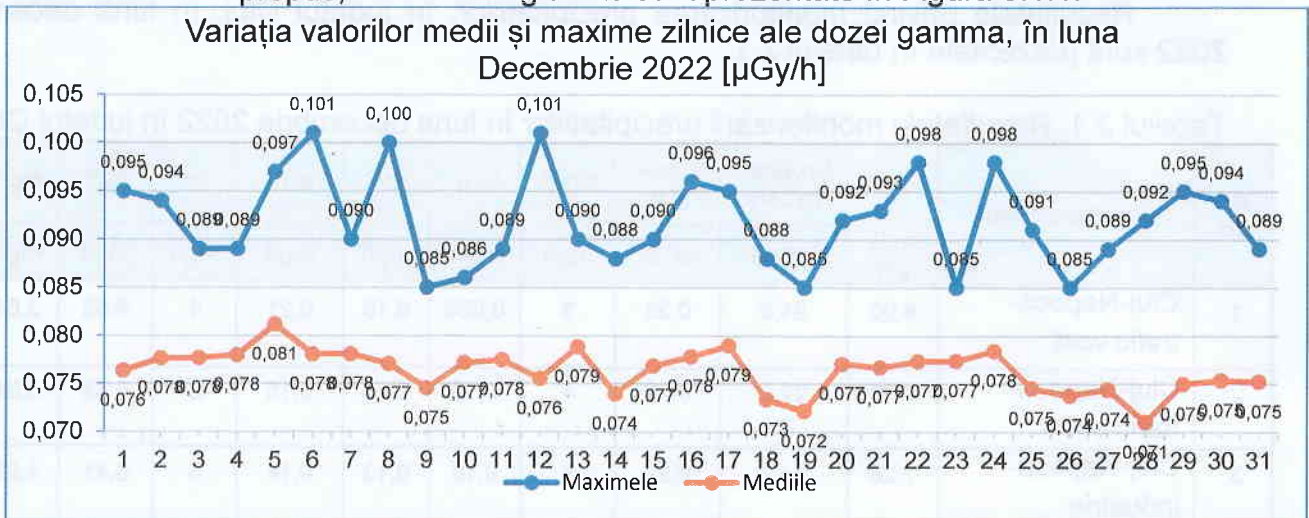
Figura nr. 3.1.1 Variația valorilor medii și maxime zilnice ale debitului dozei gamma în luna Decembrie 2022
