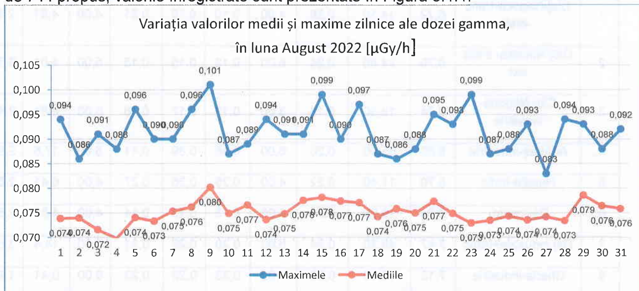
Figura nr. 3.1.1 Variația valorilor medii și maxime zilnice ale debitului dozei gamma în luna August 2022
