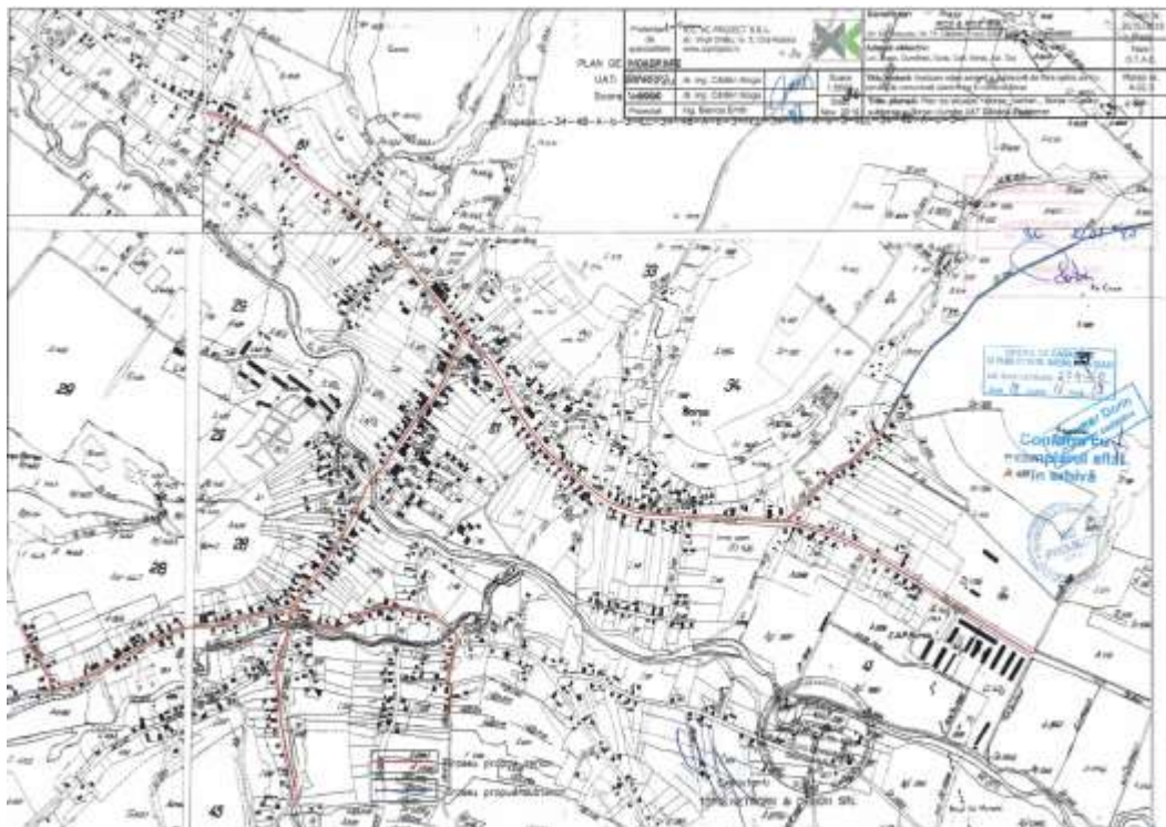
Desfășurarea rețelilor la nivelul localității Borșa (linie roșie)
