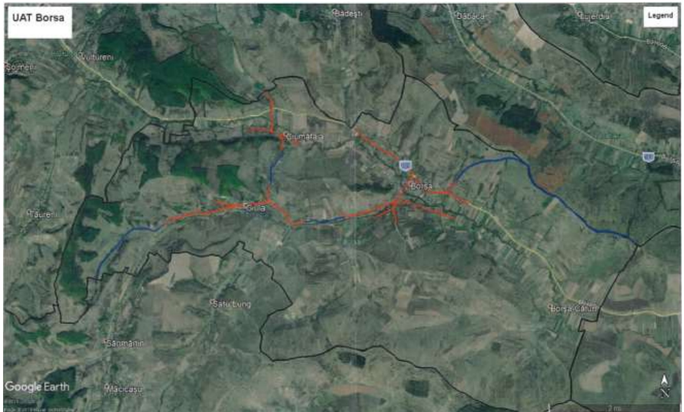
Desfășurarea rețelilor la nivelul comunei Borșa: linie roșie – trasee aeriene; linie albastră – trasee îngropate
