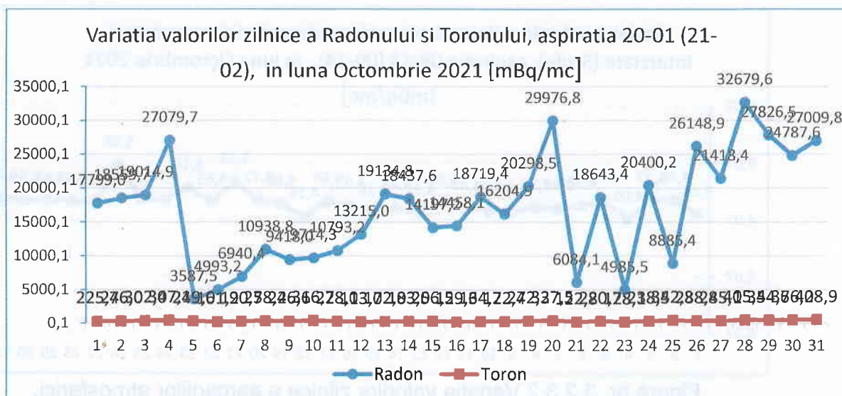
Figura nr. 3.2.2.4 aspirația 20-01
