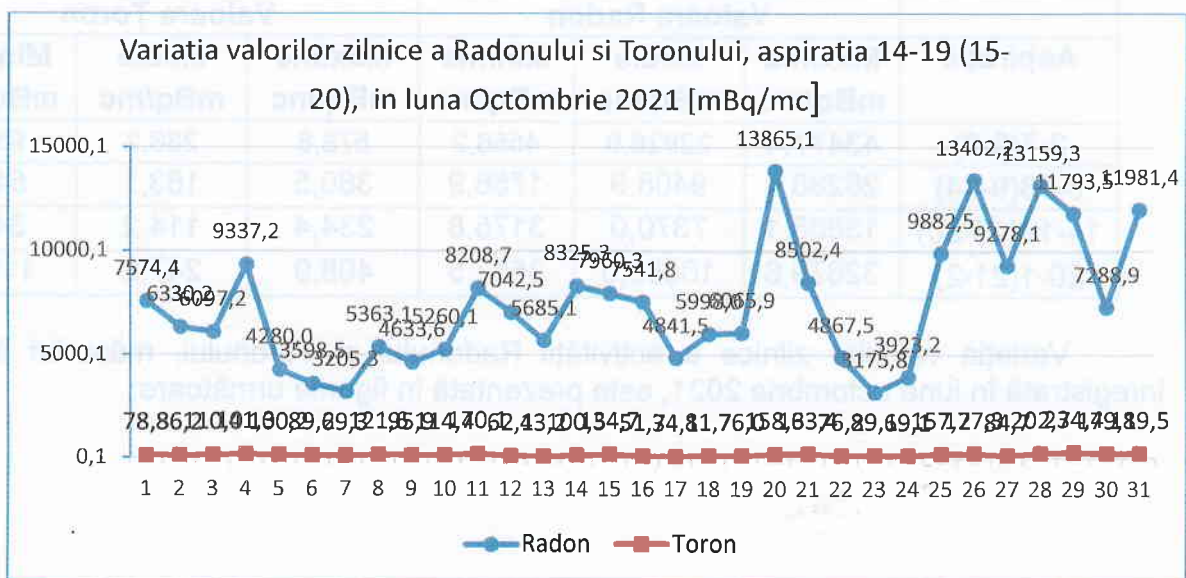
Figura nr. 3.2.2.3 aspiratia 14-19
