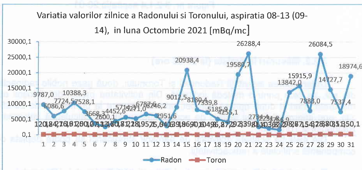
Figura nr. 3.2.2.2 aspiratia 8-13
