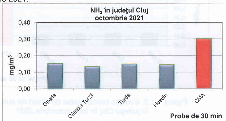
Figura 1.1.1. Evoluția concentrației de amoniac în județul Cluj în luna octombrie 2021
