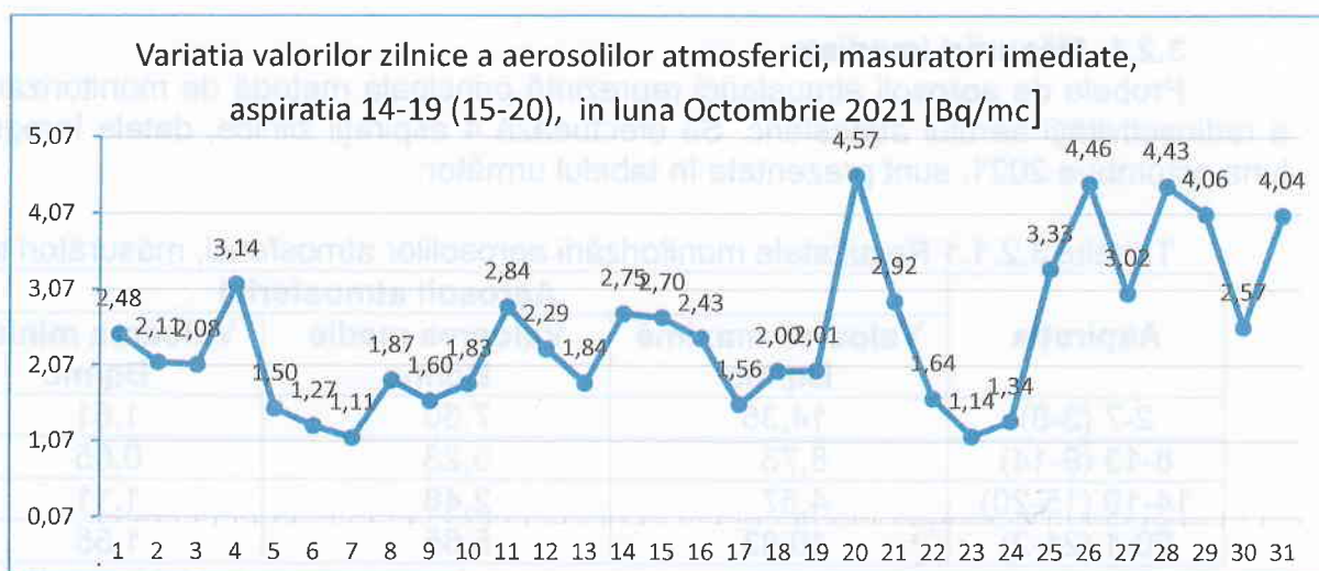
Figura nr. 3.2.1.3 aspirația 14-19
