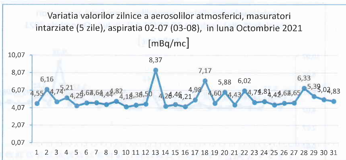
Figura nr. 3.2.3.1 Variația valorilor zilnice a aerosolilor atmosferici, măsurări la 5 zile, aspirația 03-08, în luna Octombrie 2021
