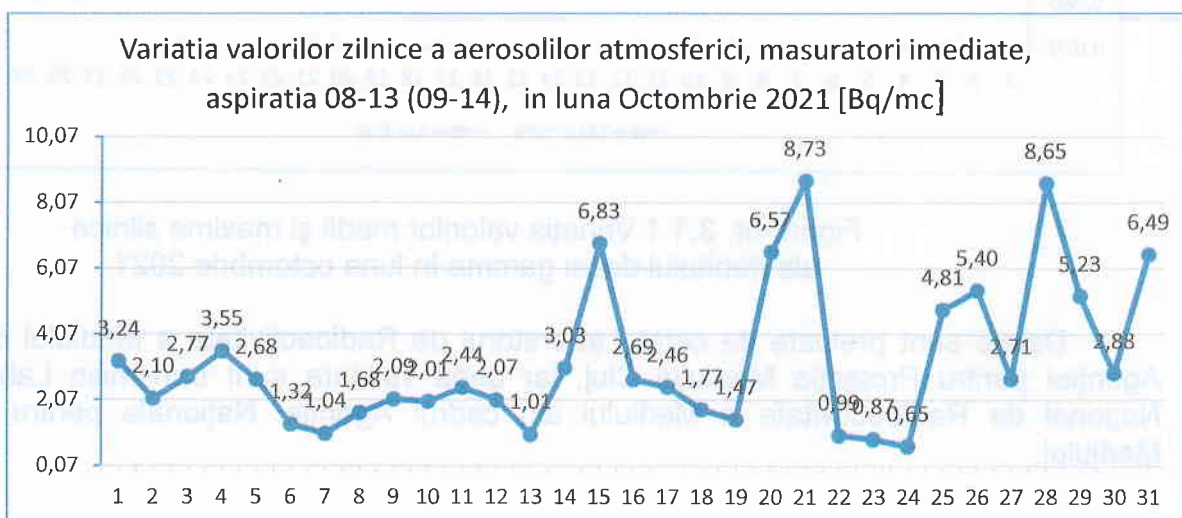
Figura nr. 3.2.1.2 aspirația 8-13
