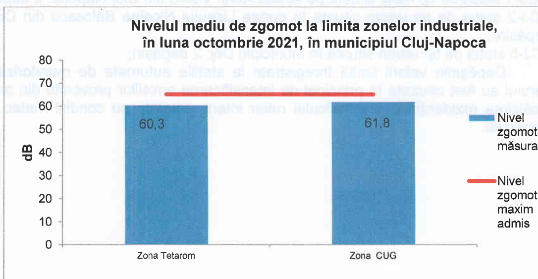
Figura 4.6. Nivelul de zgomot la limita zonelor industriale, în luna octombrie 2021
