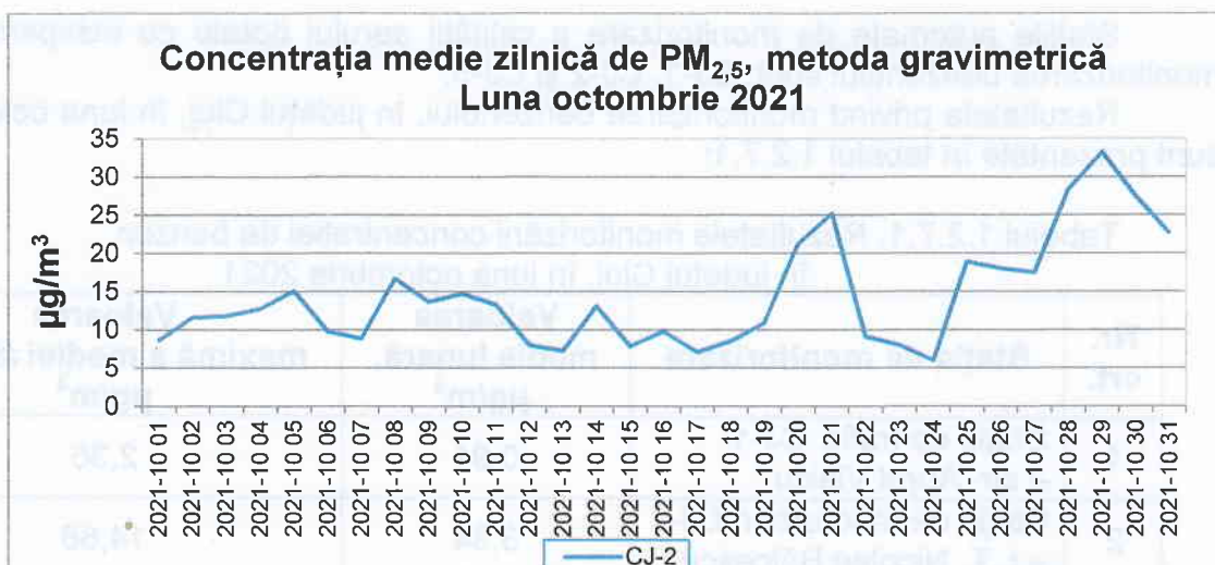
Figura 1.2.5.2. Evoluția concentrației medii zilnice de PM 2,5 , în județul Cluj, în luna octombrie 2021
