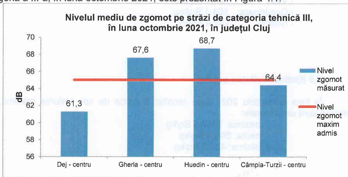
Figura 4.1. Nivelul de zgomot urban pe strazi de categoria III, în județul Cluj, în luna octombrie 2021
