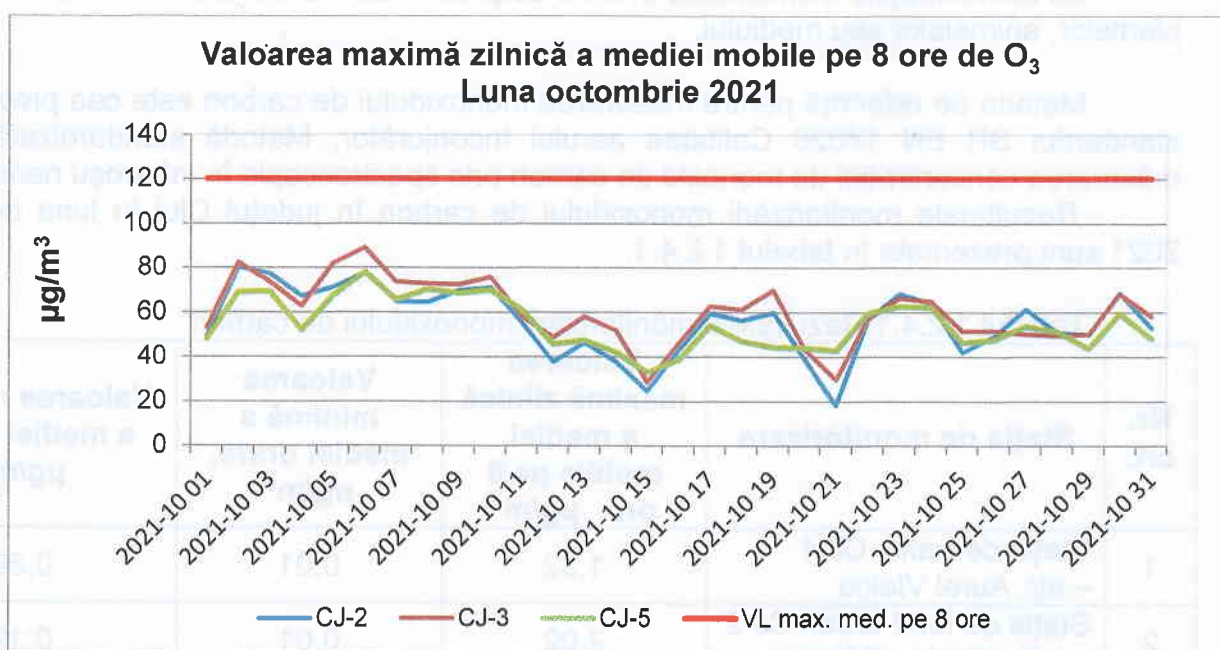
Figura 1.2.3.1. Evoluția maximelor zilnice ale mediilor mobile pe 8 ore de \text{O}_3 , în județul Cluj, în luna octombrie 2021
