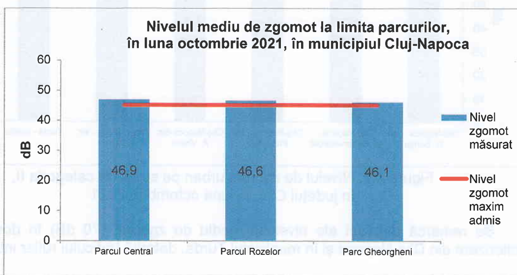
Figura 4.4. Nivelul de zgomot la limita parcurilor, în luna octombrie 2021
