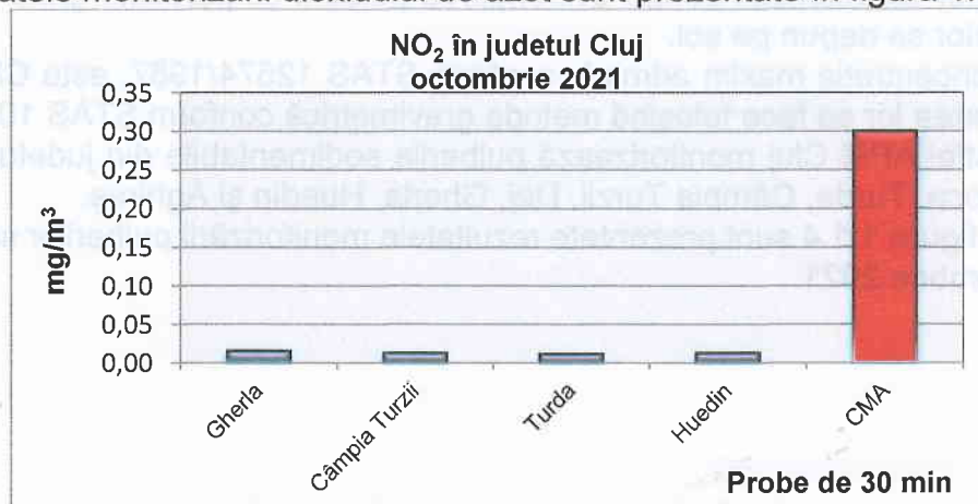
Figura 1.1.2. Evoluția concentrației de dioxid de azot în județul Cluj în luna octombrie 2021
