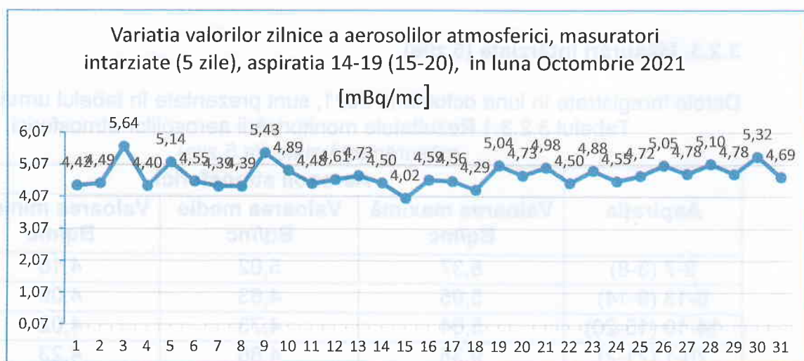
Figura nr. 3.2.3.3 Variația valorilor zilnice a aerosolilor atmosferici, măsurări la 5 zile, aspirația 14-19, în luna Octombrie 2021
