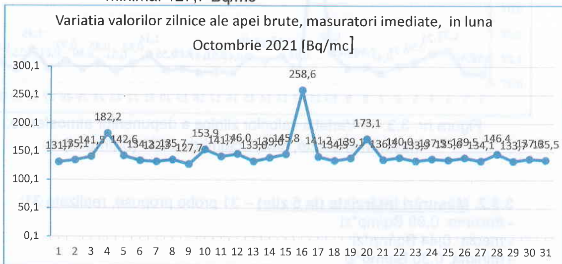
Figura nr. 3.4.1.1.1 Variația valorilor zilnice ale apei brute, măsurări imediate, luna octombrie 2021
