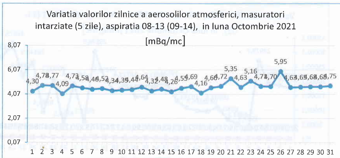
Figura nr. 3.2.3.2 Variația valorilor zilnice a aerosolilor atmosferici, măsurări la 5 zile, aspirația 08-13, în luna Octombrie 2021
