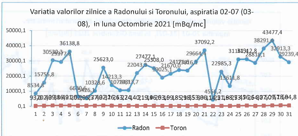
Figura nr. 3.2.2.1 aspiratia 2-7
