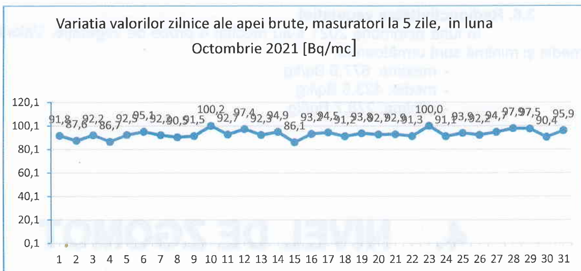
Figura nr. 3.4.1.2.1 Variația valorilor zilnice ale apei brute, măsurări la 5 zile, luna octombrie 2021
