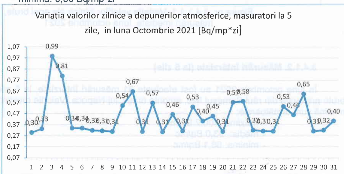
Figura nr. 3.3.2.1 Variația valorilor zilnice a depunerilor atmosferice, măsurări la 5 zile, luna Octombrie 2021 [Bq/mp*zi]
