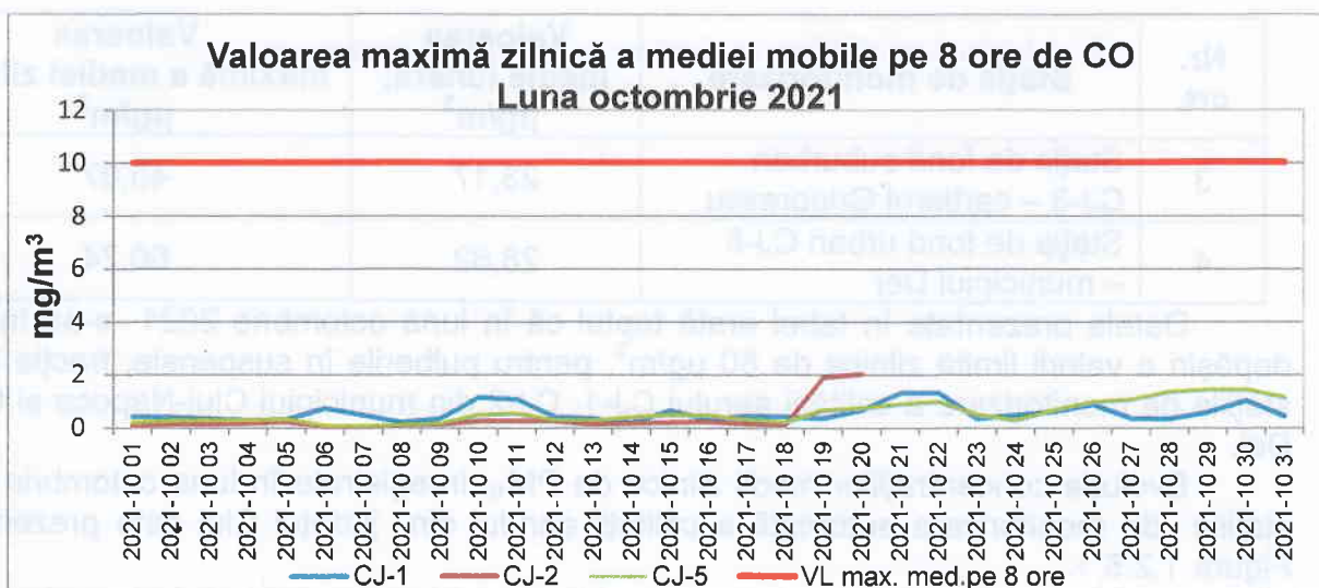
Figura 1.2.4.1. Evoluția concentrațiilor maxime zilnice a mediilor mobile pe 8 ore de CO, în județul Cluj, în luna octombrie 2021
