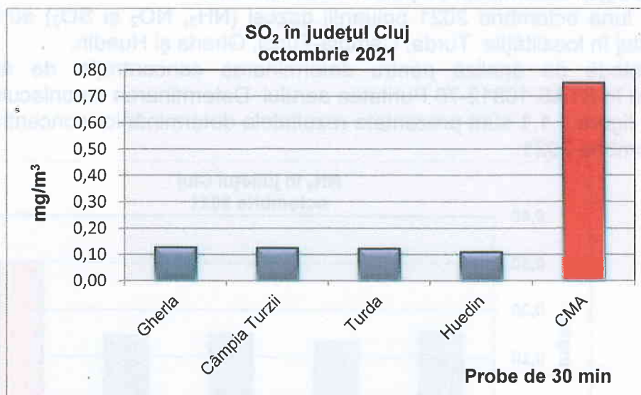
Figura 1.1.3. Evoluția concentrației de dioxid de sulf în județul Cluj în luna octombrie 2021
