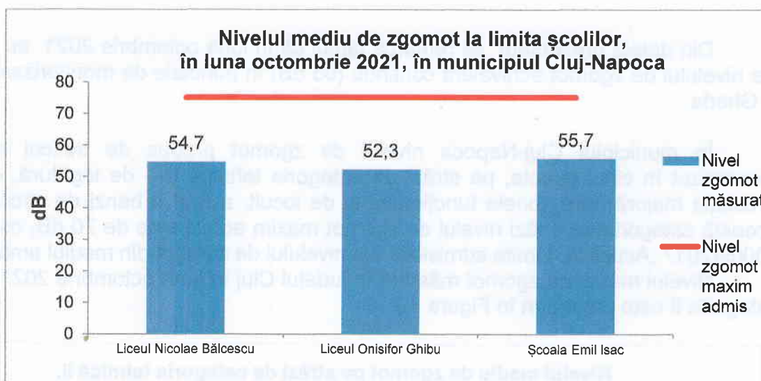
Figura 4.3. Nivelul de zgomot la limita școlilor, în luna octombrie 2021
