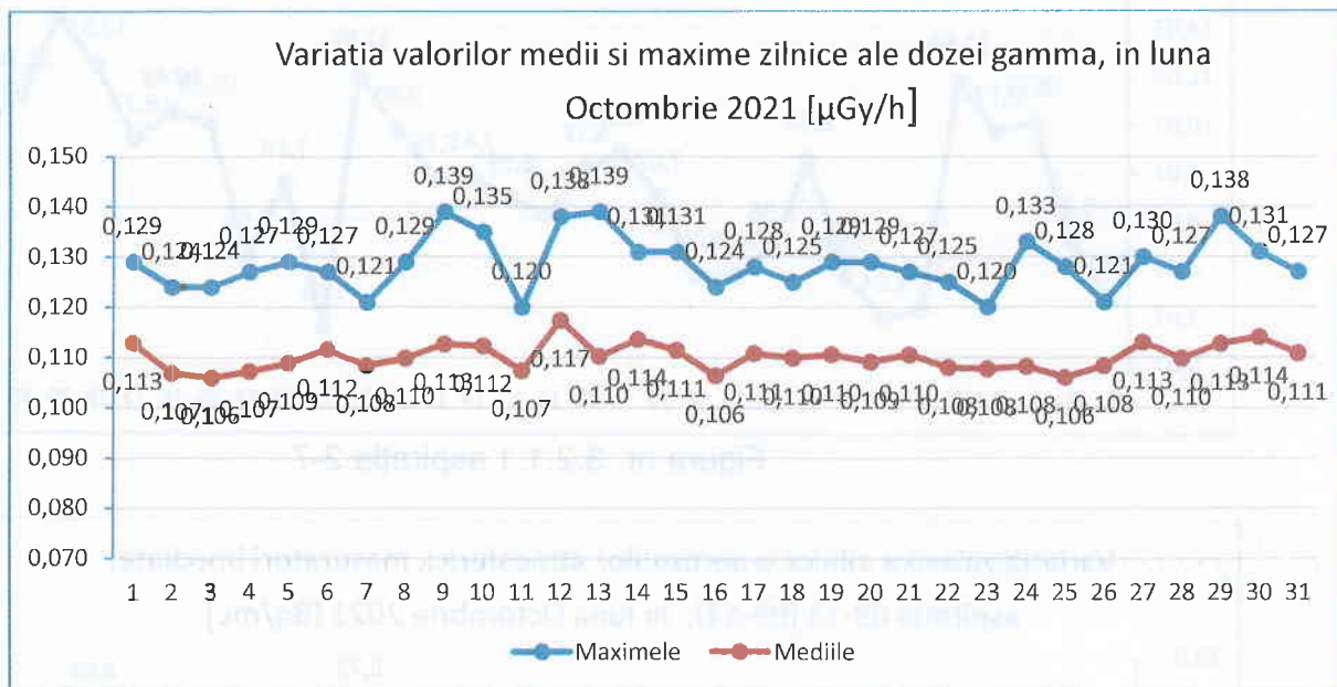
Figura nr. 3.1.1 Variația valorilor medii și maxime zilnice ale debitului dozei gamma în luna octombrie 2021
