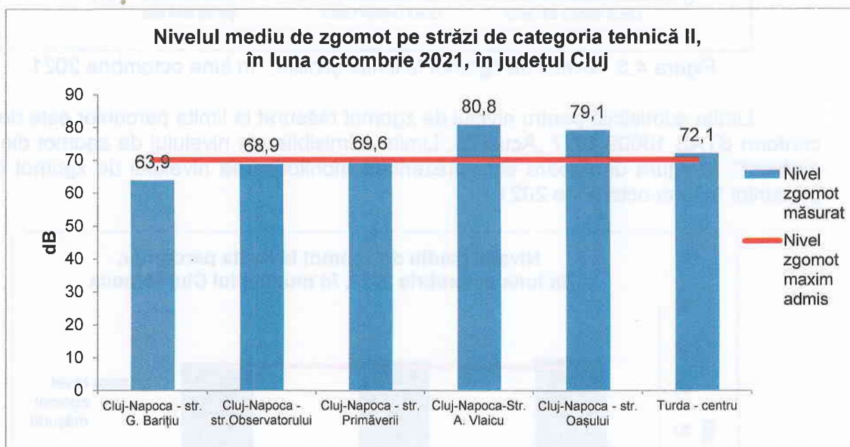
Figura 4.2. Nivelul de zgomot urban pe străzi de categoria II, în județul Cluj, în luna octombrie 2021
