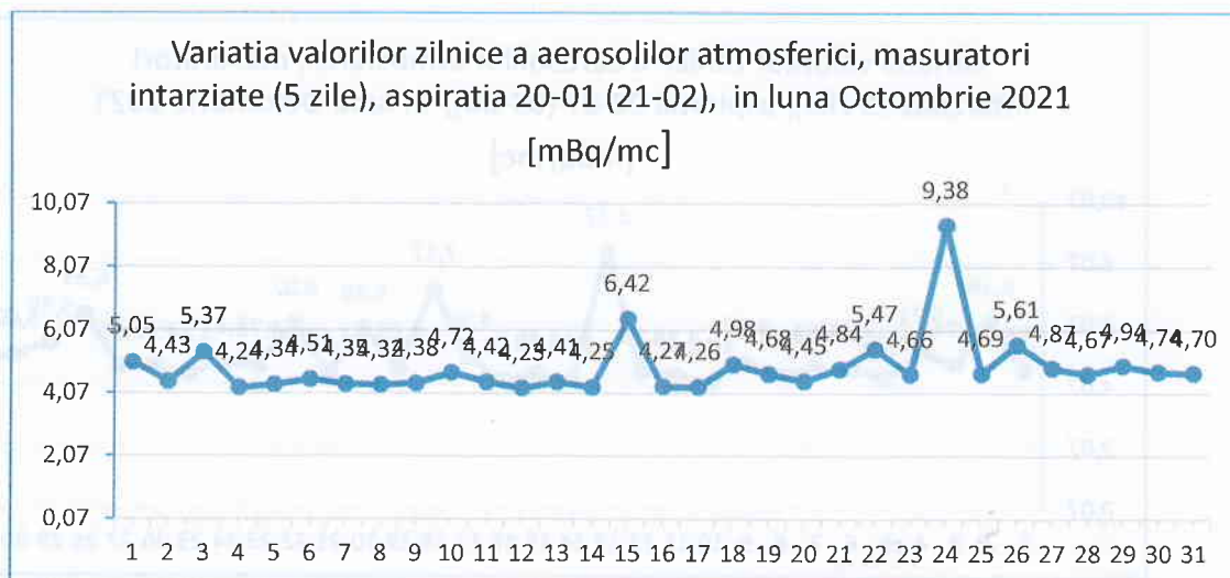
Figura nr. 3.2.3.4 Variația valorilor zilnice a aerosolilor atmosferici, măsurări la 5 zile, aspirația 20-01, în luna Octombrie 2021
