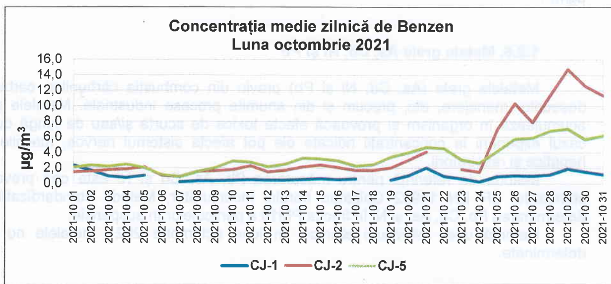
Figura 1.2.7.1. Evoluția concentrației medii zilnice de benzen în județul Cluj, în luna octombrie 2021
