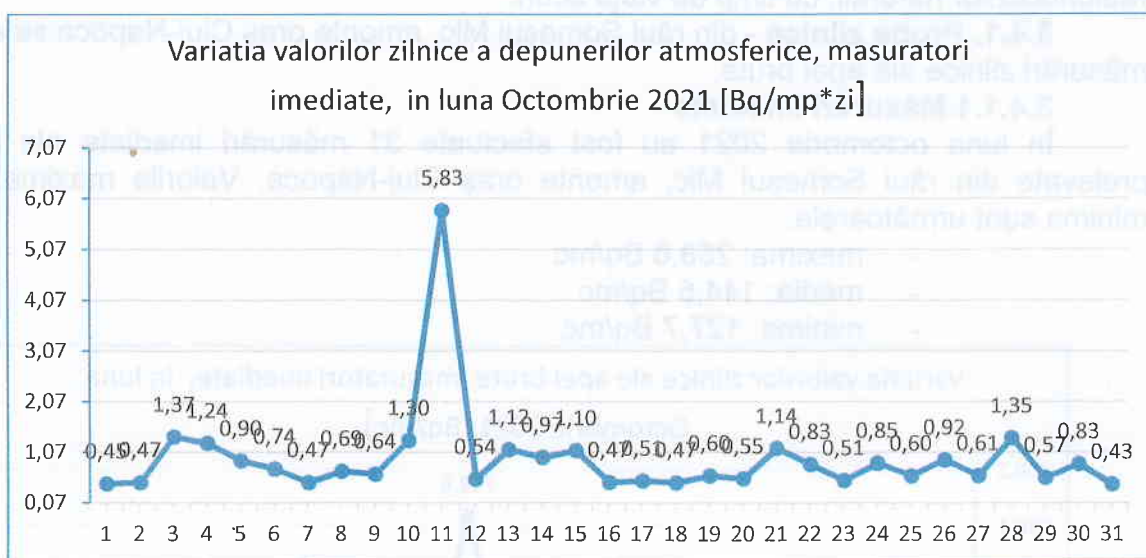
Figura nr. 3.3.1.1 Variația valorilor zilnice a depunerilor atmosferice, măsurări imediate, luna Octombrie 2021 [Bq/mp*zi]
