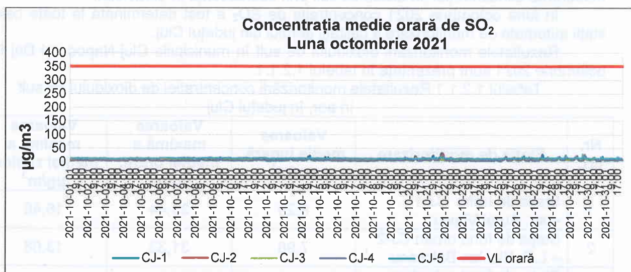
Figura 1.2.1.2. Evoluția concentrației medii orare de \text{SO}_2 în județul Cluj în luna octombrie 2021
