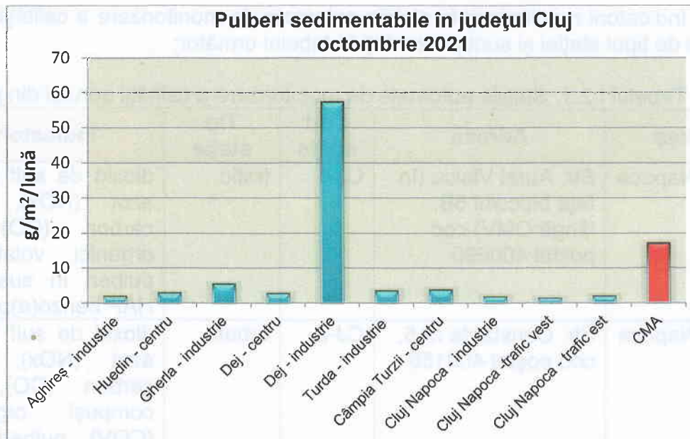
Figura 1.1.4. Evoluția concentrației de pulberi sedimentabile în județul Cluj în luna octombrie 2021
