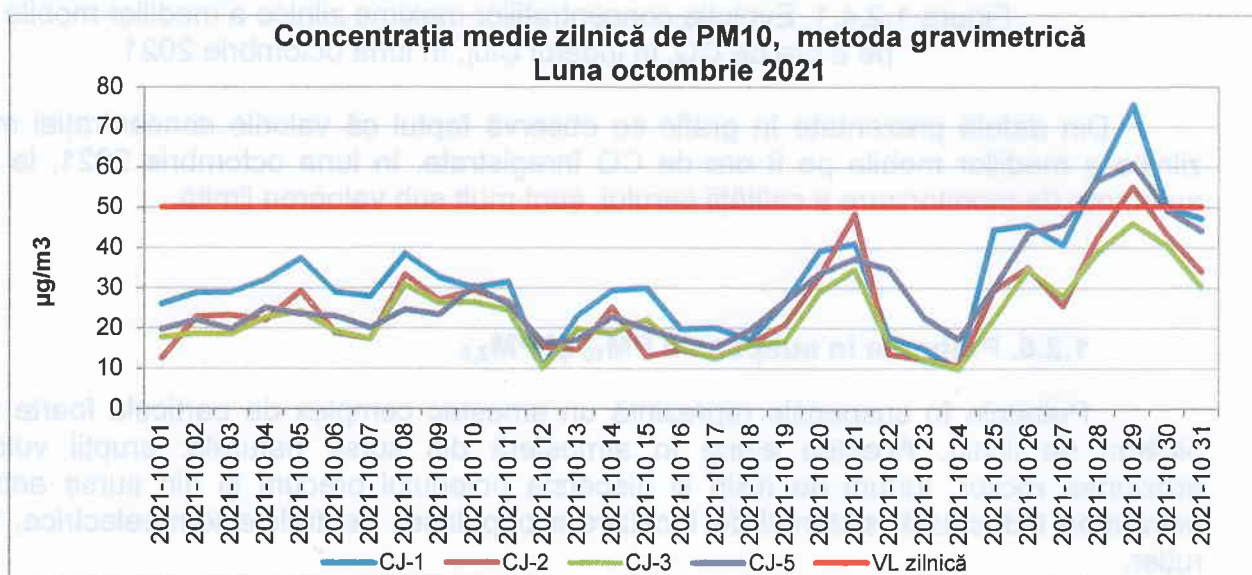
Figura 1.2.5.1. Evoluția concentrației medii zilnice de \text{PM}_{10} , în județul Cluj, în luna octombrie 2021
