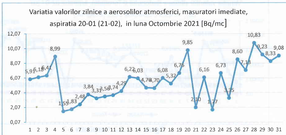
Figura nr. 3.2.1.4 aspirația 20-01
