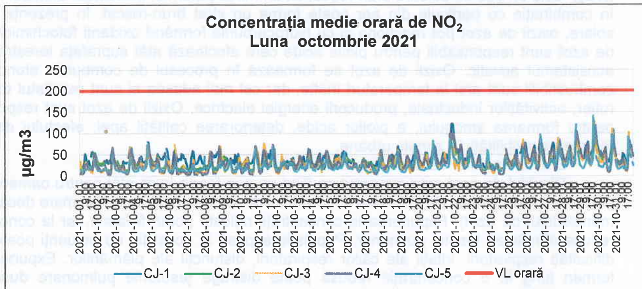
Figura 1.2.2.1. Evoluția concentrațiilor medii orare de \text{NO}_2 în județul Cluj în luna octombrie 2021
