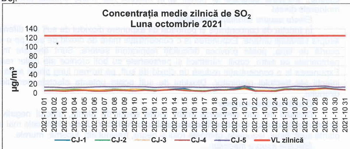
Figura 1.2.1.1. Evoluția concentrației medii zilnice de \text{SO}_2 în județul Cluj în luna octombrie 2021
