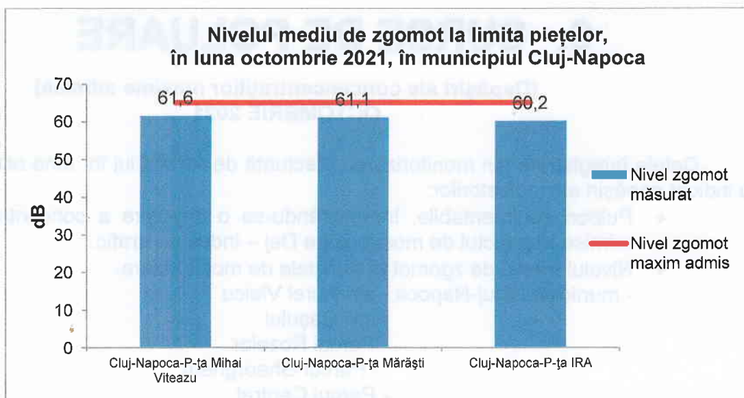
Figura 4.5. Nivelul de zgomot la limita piețelor, în luna octombrie 2021
