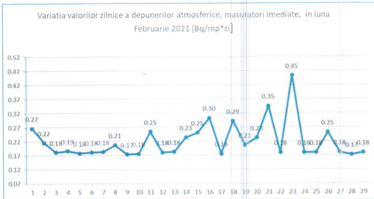
Figura nr. 3.3.1.1 Variația valorilor zilnice a depunerilor atmosferice, măsurări imediate, luna Februarie 2021 [Bq/mp*zi]
