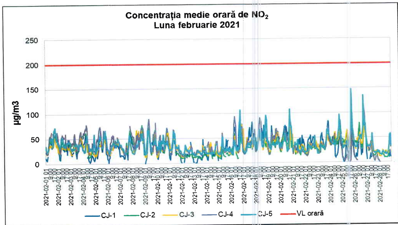
Figura 1.2.2.1. Evoluția concentrațiilor medii orare de \text{NO}_2 în județul Cluj în luna februarie 2021
