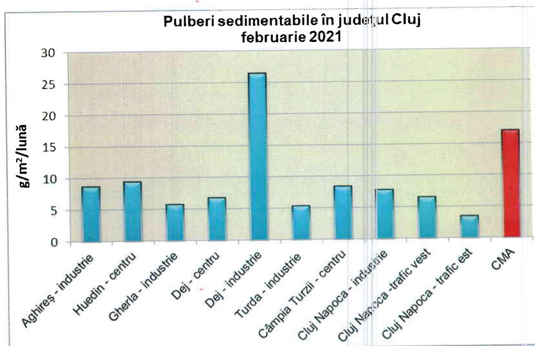
Figura 1.1.4. Evoluția concentrației de pulberi sedimentabile în județul Cluj în luna februarie 2021
