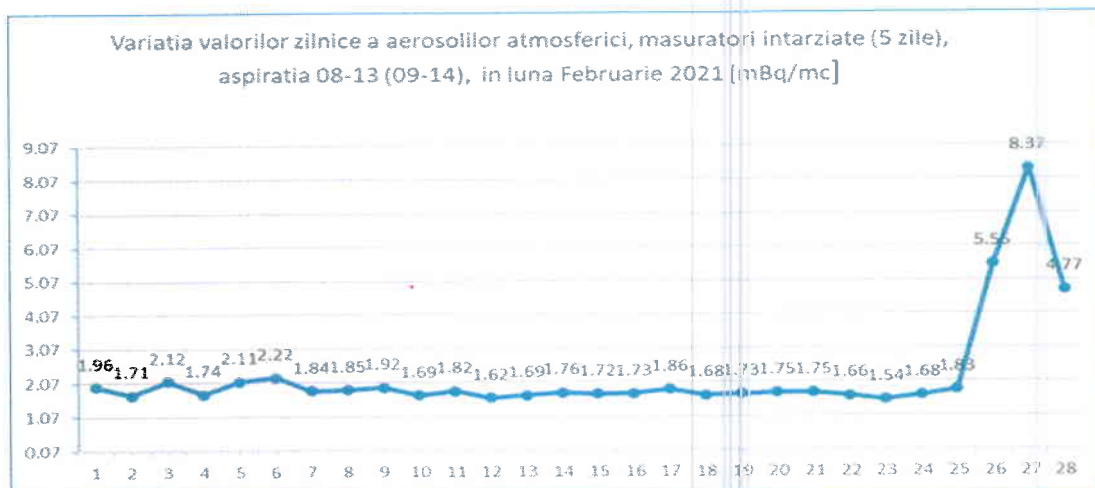
Figura nr. 3.2.3.2 Variația valorilor zilnice a aerosolilor atmosferici, măsurări la 5 zile, aspirația 08-13, în luna Februarie 2021
