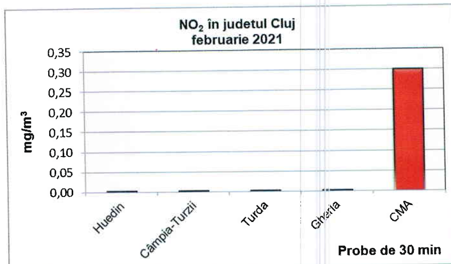
Figura 1.1.2. Evoluția concentrației de dioxid de azot în județul Cluj în luna februarie 2021
