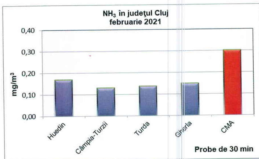
Figura 1.1.1. Evoluția concentrației de amoniac în județul Cluj în luna februarie 2021
