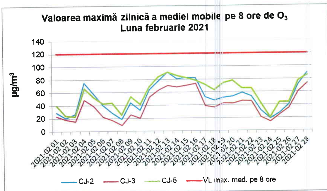
Figura 1.2.3.1. Evoluția maximelor zilnice ale mediilor mobile pe 8 ore de \text{O}_3 , în județul Cluj, în luna februarie 2021
