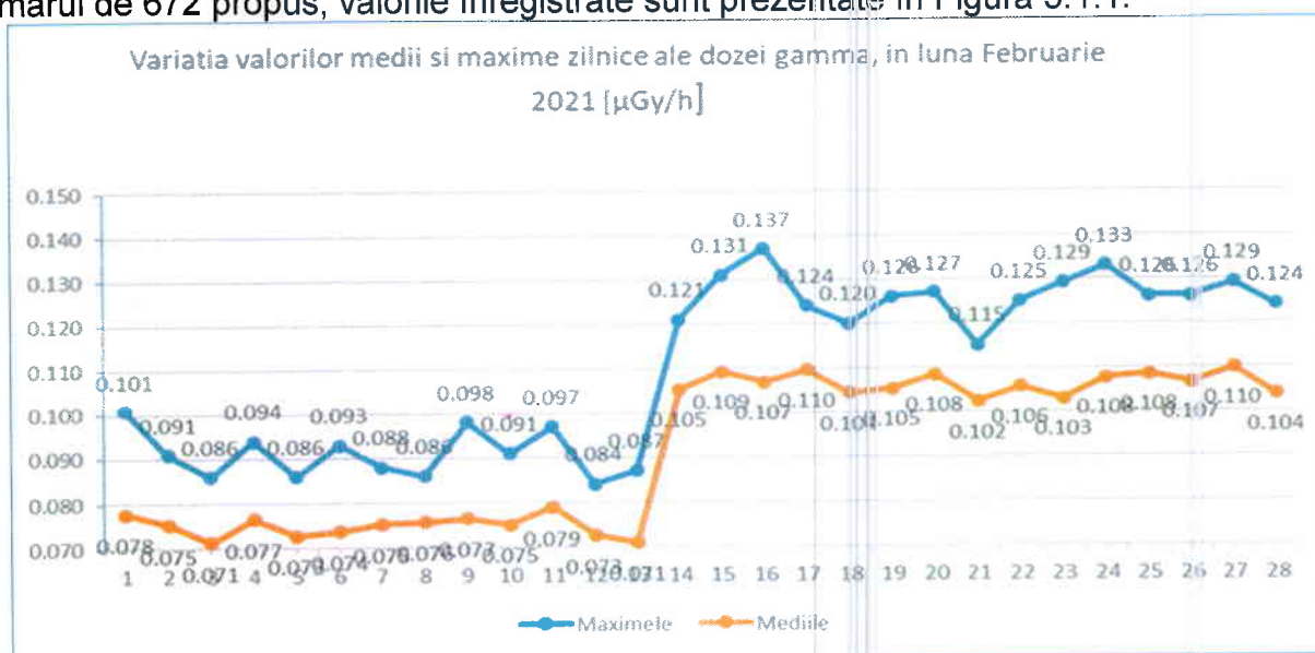
Figura nr. 3.1.1 Variația valorilor medii și maxime zilnice ale debitului dozei gamma în luna februarie 2021
