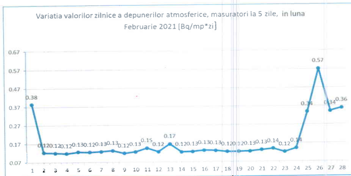
Figura nr. 3.3.2.1 Variația valorilor zilnice a depunerilor atmosferice, măsurări la 5 zile, luna Februarie 2021 [Bq/mp*zi]
