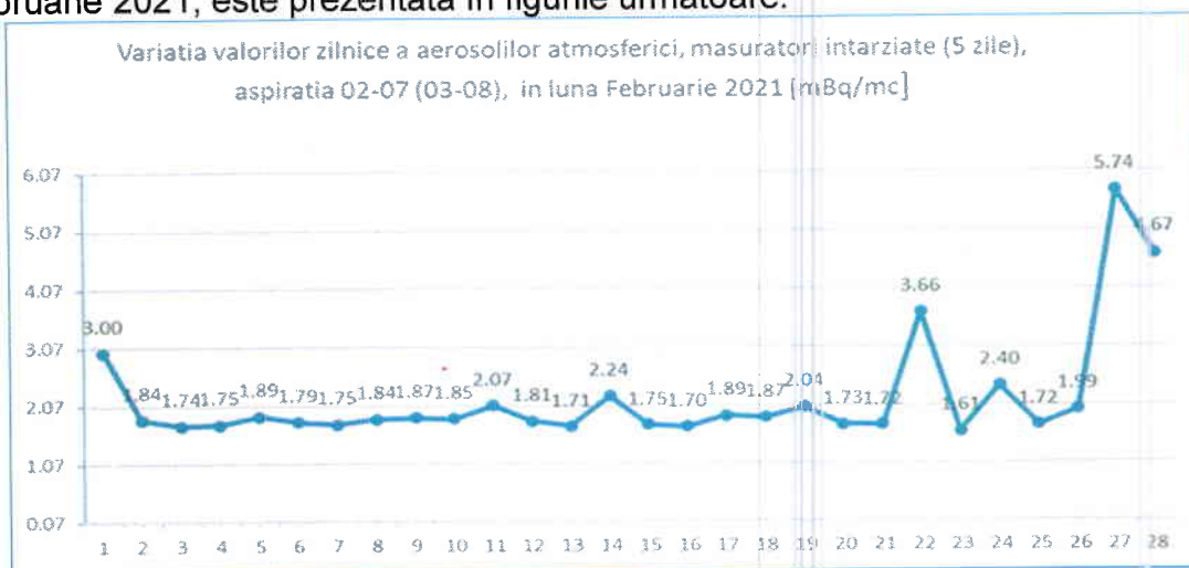
Figura nr. 3.2.3.1 Variația valorilor zilnice a aerosolilor atmosferici, măsurări la 5 zile, aspirația 03-08, în luna Februarie 2021
