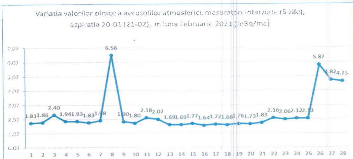
Figura nr. 3.2.3.4 Variația valorilor zilnice a aerosolilor atmosferici, măsurări la 5 zile, aspirația 20-01, în luna Februarie 2021
