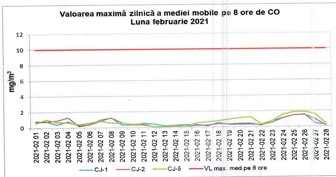
Figura 1.2.4.1. Evoluția concentrațiilor maxime zilnice a mediilor mobile pe 8 ore de CO, în județul Cluj, în luna februarie 2021
