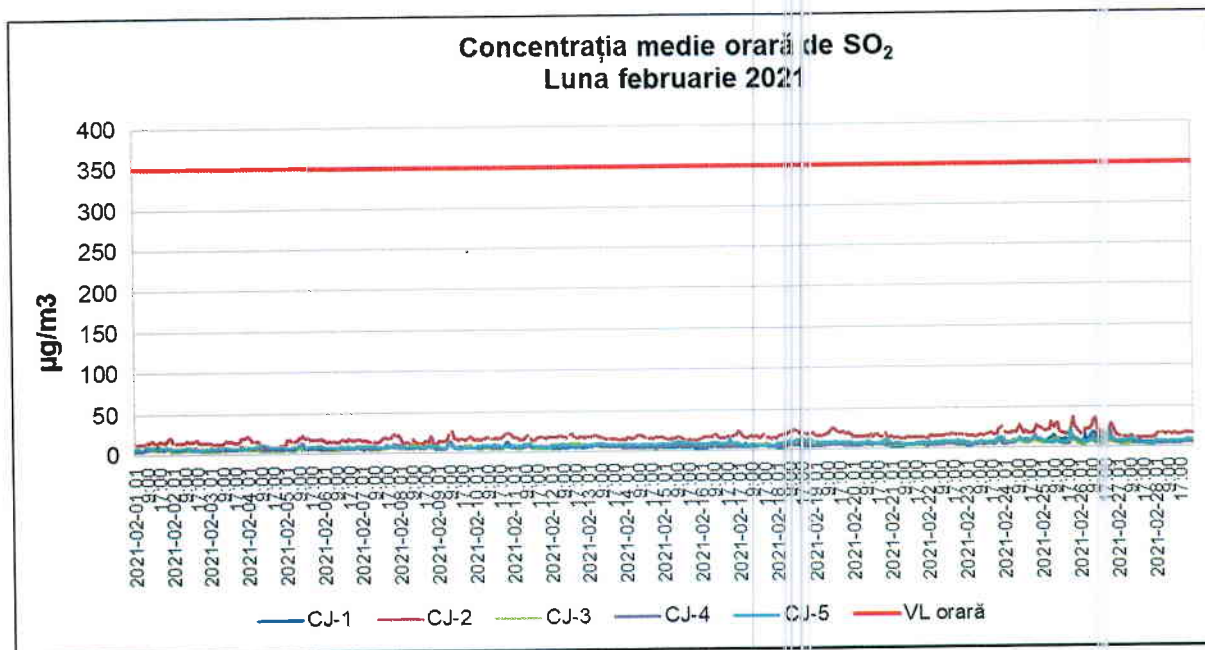
Figura 1.2.1.2. Evoluția concentrației medii orare de SO 2 în județul Cluj în luna februarie 2021
