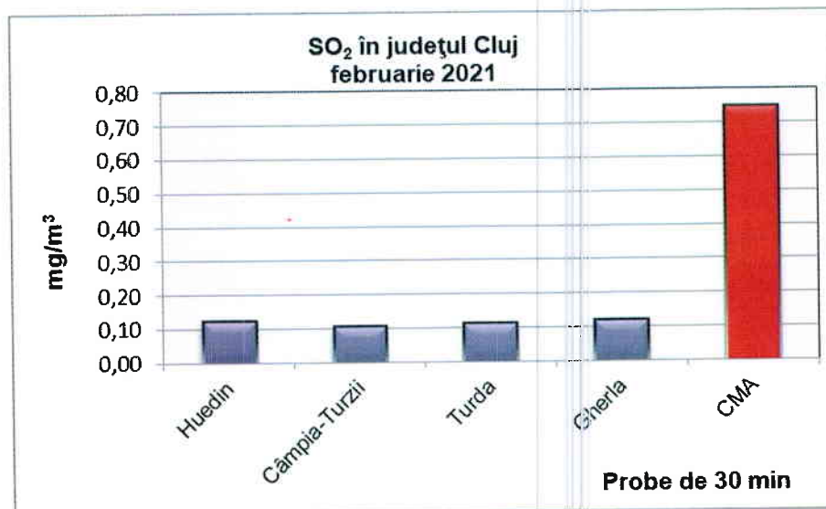
Figura 1.1.3. Evoluția concentrației de dioxid de sulf în județul Cluj în luna februarie 2021
