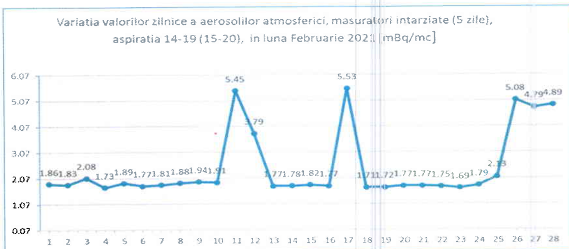
Figura nr. 3.2.3.3 Variația valorilor zilnice a aerosolilor atmosferici, măsurări la 5 zile, aspirația 14-19, în luna Februarie 2021
