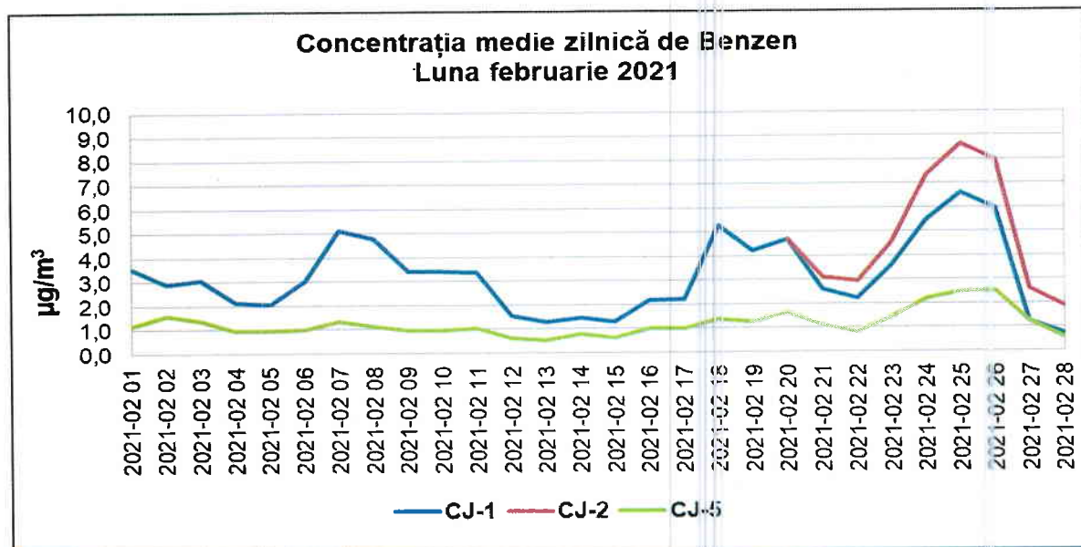
Figura 1.2.7.1. Evoluția concentrației medii de zilnice de benzen în județul Cluj, în luna februarie 2021
