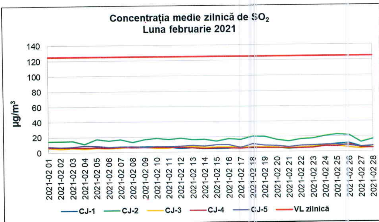
Figura 1.2.1.1. Evoluția concentrației medii zilnice de SO 2 În județul Cluj în luna februarie 2021
