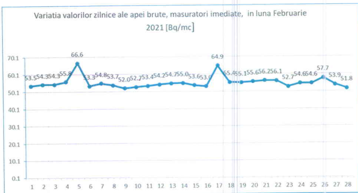
Figura nr. 3.4.1.1.1 Variația valorilor zilnice ale apei brute, măsurări imediate, luna februarie 2021
