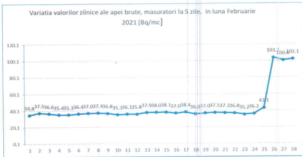
Figura nr. 3.4.1.2.1 Variația valorilor zilnice ale apei brute, măsurări la 5 zile, luna februarie 2021
