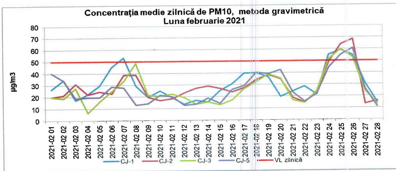
Figura 1.2.5.1. Evoluția concentrației medii zilnice de PM 10 , în județul Cluj, în luna februarie 2021
