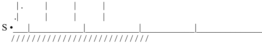
Figura 2.5.h: Unda de sunet reflectată la ordinul de 4 pe o linie aflată într-un șanț: secțiunea transversală actuală (partea superioară), secțiunea transversală nedesfășurată (partea inferioară)
