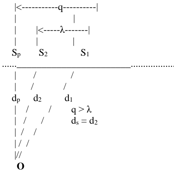
Figura 2.7.l: Geometria segmentului traiectului de zbor pentru poziția observatorului înaintea segmentului
