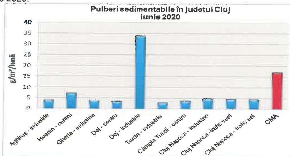
Figura 1.1.4. Rezultatele monitorizării pulberilor sedimentabile
