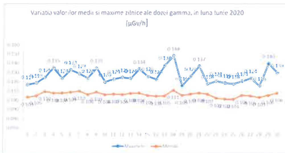
Fig. nr. 3.1.1 Variația valorilor medii și maxime zilnice ale debitului dozei gamma în luna iunie 2020
