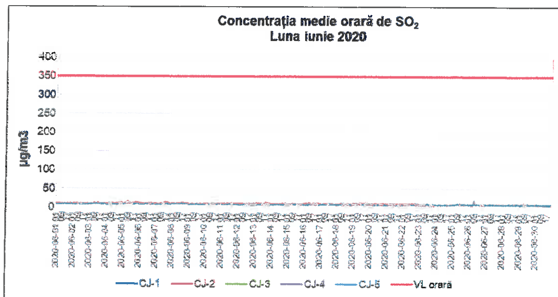
Figura 1.2.1.2. Evoluția mediilor orare de SO 2 în luna iunie 2020
