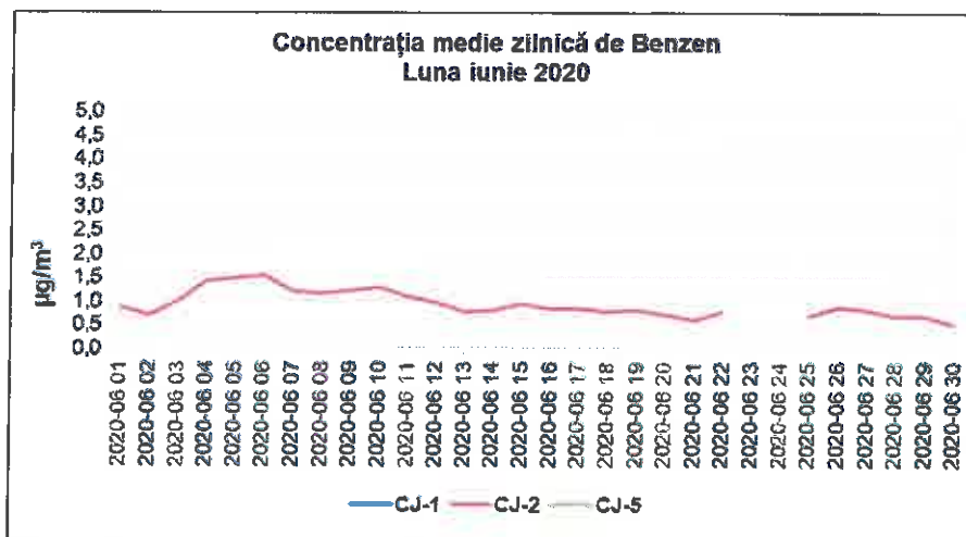
Figura 1.2.7.1. Evoluția mediilor zilnice de benzen, în luna iunie 2020
