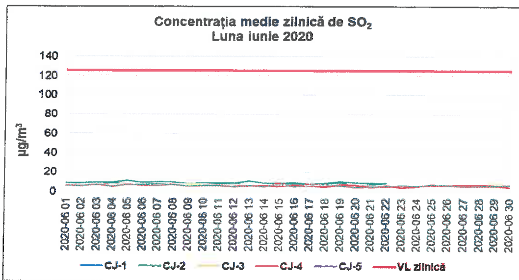
Figura 1.2.1.1. Evoluția mediilor zilnice de SO 2 în luna iunie 2020
