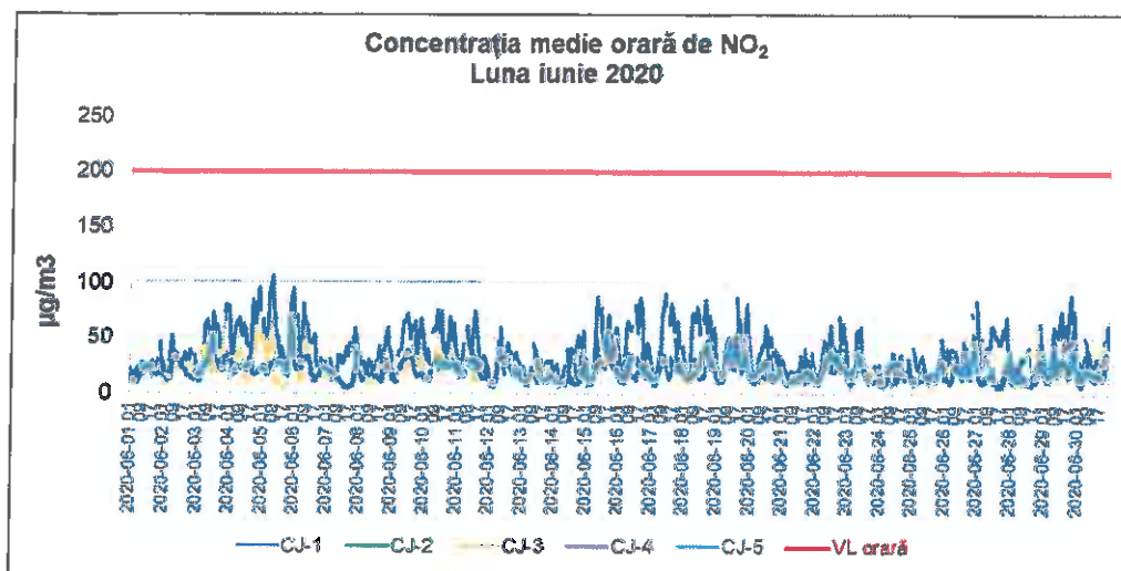
Figura 1.2.2.1. Evoluția mediilor orare de NO 2 în luna iunie 2020
