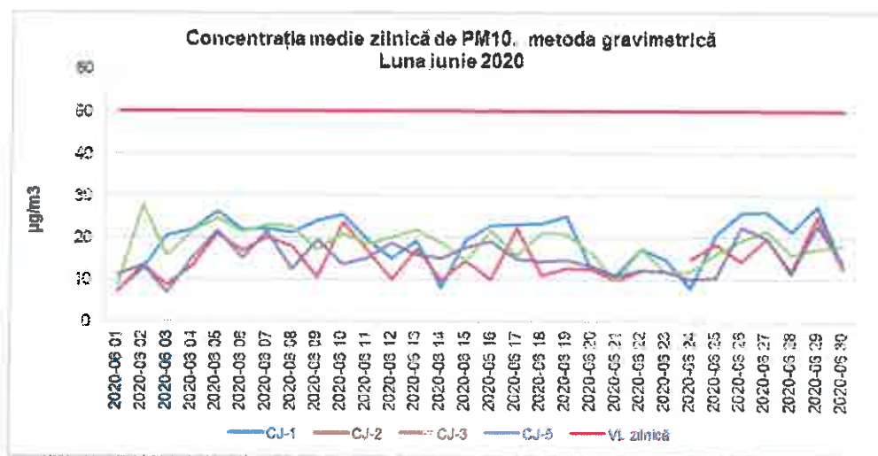
Figura 1.2.5.1. Evoluția mediilor zilnice de PM 10 , în luna iunie 2020
