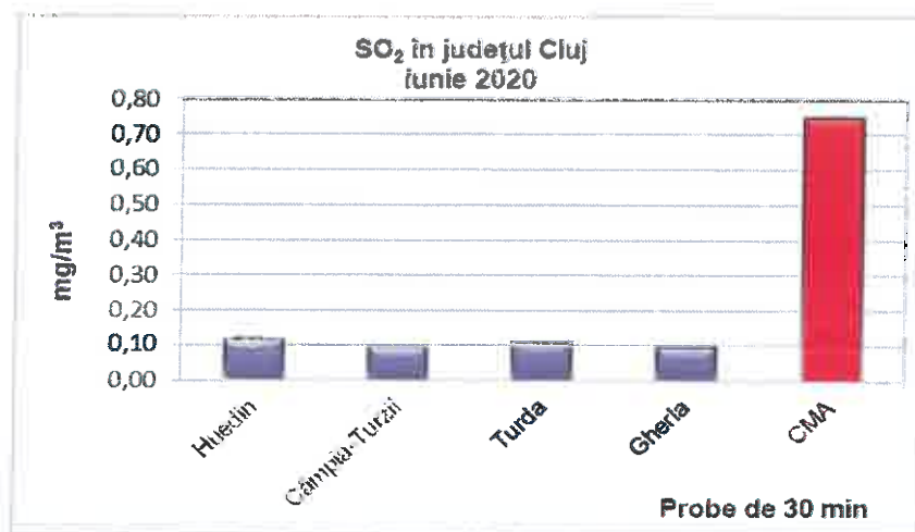
Figura 1.1.3. Rezultatele monitorizării dioxidului de sulf
