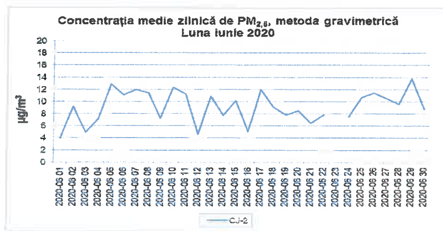
Figura 1.2.5.2. Evoluția mediilor zilnice de PM_{10} , în luna iunie 2020
