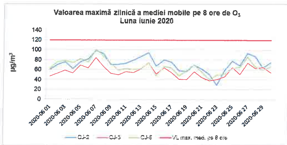
Figura 1.2.3.1. Evoluția maximelor zilnice ale mediilor mobile pe 8 ore de \text{O}_3 , în luna iunie 2020
