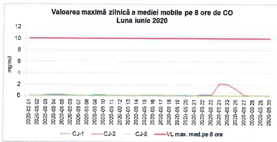
Figura 1.2.4.1. Evoluția maximelor zilnice ale mediilor mobile pe 8 ore de CO, în luna iunie 2020
