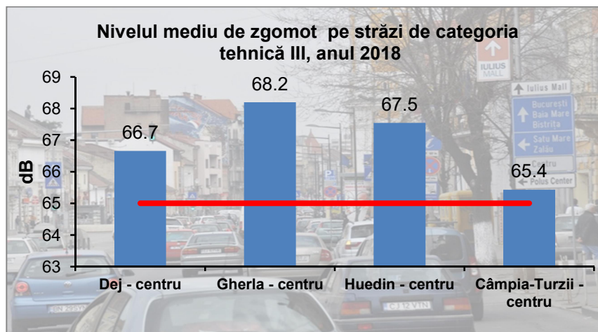
Figura VIII.1.2.1.8. Nivelul de zgomot urban în județul Cluj, în anul 2018 ) 20
