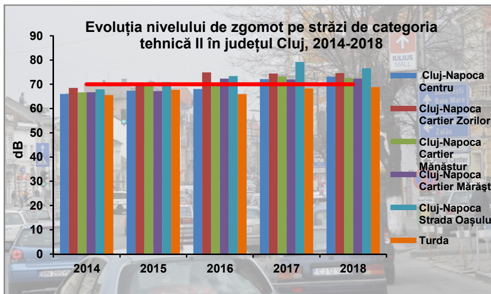
Figura VIII.1.2.1.10. Evoluția nivelului de zgomot în județul Cluj, străzi de categorie tehnică II ) 22
