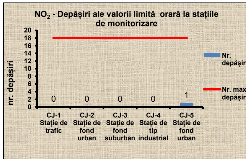
Figura VIII.1.1.1.4 Numărul de depășiri ale concentrației medii orare pentru dioxidul de azot, raportat la numărul maxim de depășiri permise ) 4
