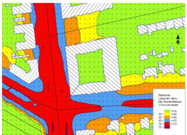
Figura VIII.1.2.1.1. Harta strategică de zgomot ) 9
