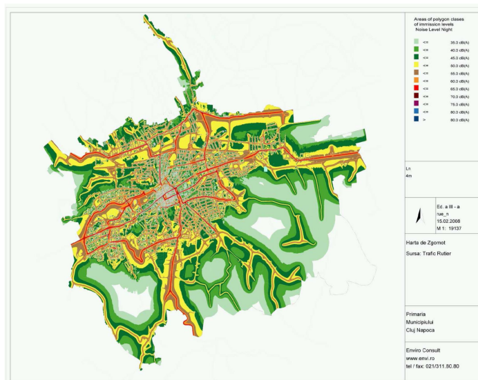
Figura VIII.1.2.1.3. Harta de zgomot pentru traficul rutier, indicatorul L_{noapte} ;) 11
