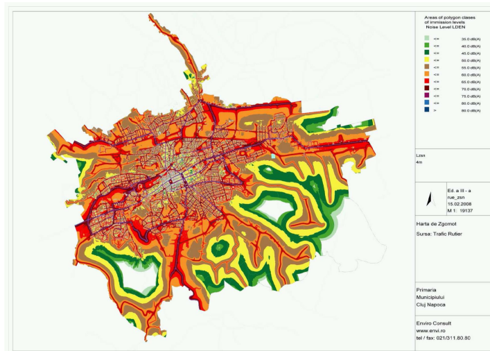
Figura VIII.1.2.1.2. Harta de zgomot pentru traficul rutier, indicatorul L_{zsn} ) 10
