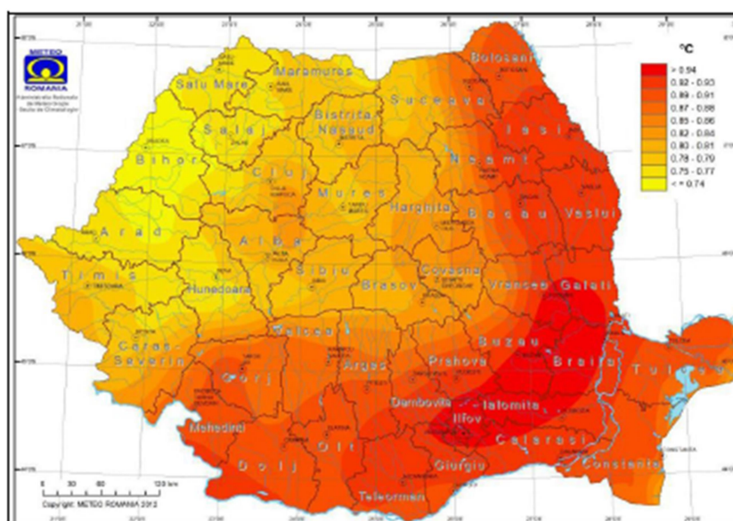
Figura VIII.1.5.1.2. Creșterea temperaturii medii multianuale (°C) în intervalul 2001-2030 comparativ cu intervalul de referință 1961-1990 ) 28
