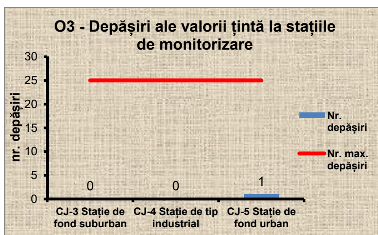
Figura VIII.1.1.1.2 Numărul de depășiri ale maximei mediilor pe 8 ore pentru ozon, raportat la numărul maxim de depășiri permise ) 2
