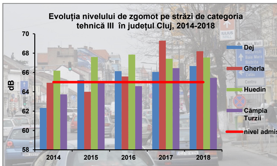
Figura VIII.1.2.1.9. Evoluția nivelului de zgomot în județul Cluj, străzi de categoria tehnică III ) 21
