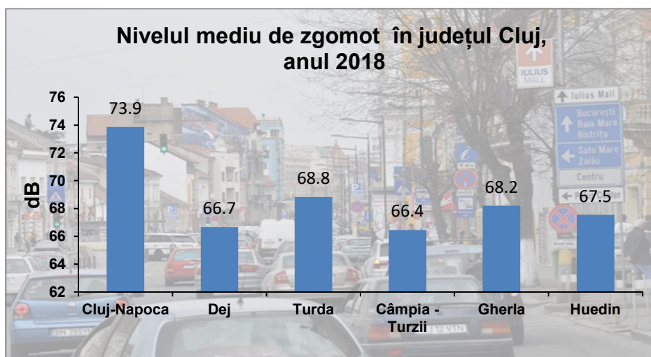
Figura VIII.1.2.1.6 Nivelul de zgomot urban în județul Cluj, în anul 2018 ) 18
