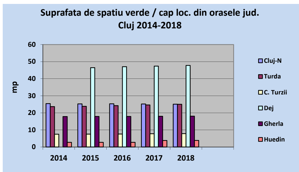
Figura VIII.1.4.1.2. Suprafața de spațiu verde/cap de locuitor din orașele județului Cluj în perioada 2014-2018 (mp/cap de locuitor)
