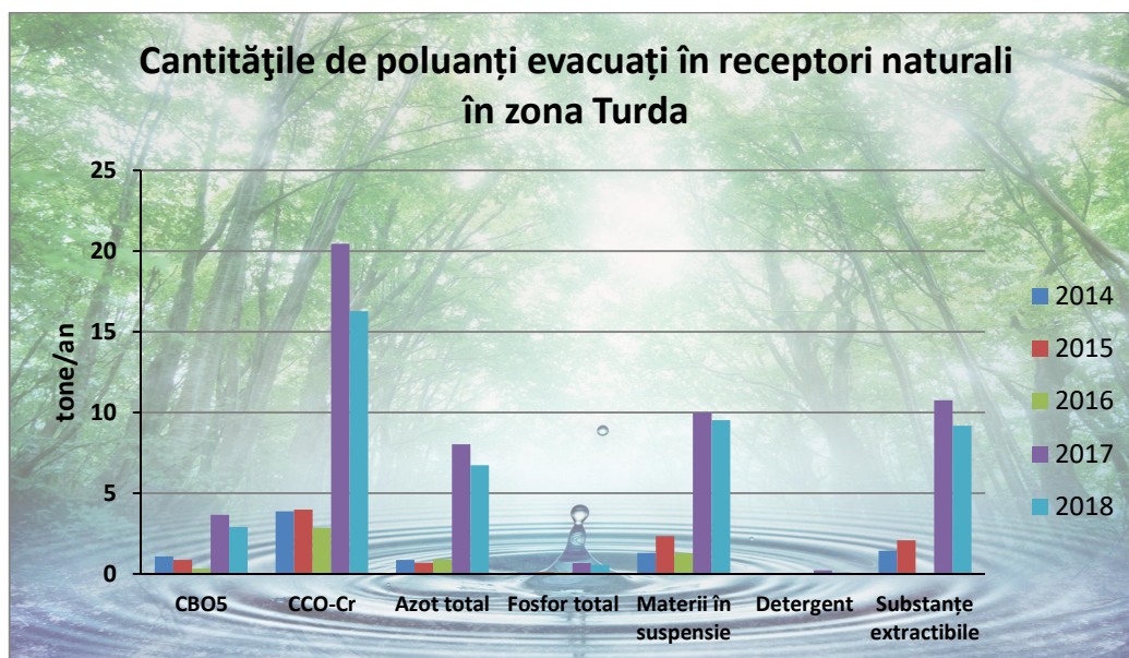
Figura II.2.2.2.10. Cantitățile de poluanți evacuați în receptori naturali în zona Turda, în perioada 2014-2018
