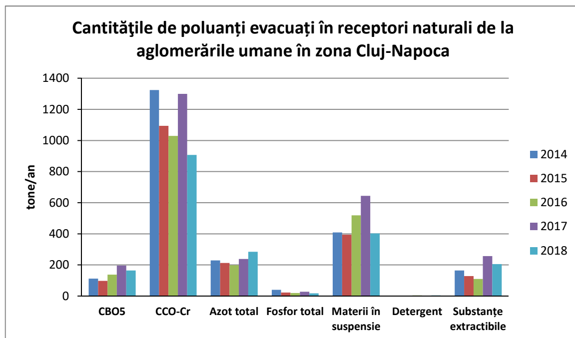
Figura II.2.2.2.2. Cantitățile de poluanți evacuați în receptori naturali de la aglomerările umane în zona Cluj-Napoca, în perioada 2014-2018
