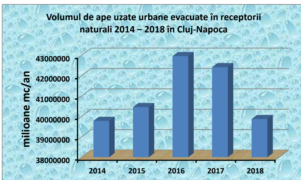
Figura II.2.2.13. Volumul de ape uzate urbane evacuate în receptorii naturali în perioada 2014 – 2018 de la stația de epurare din Cluj-Napoca
