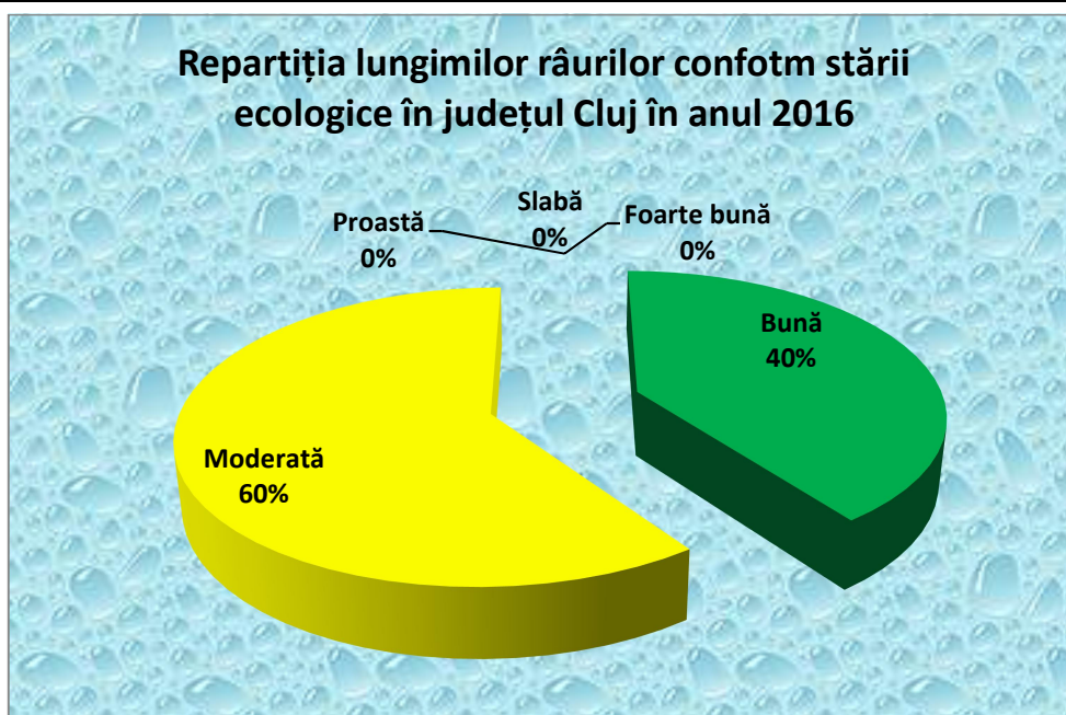
Figura II.2.1.1.1. Starea ecologică a râurilor din Bazinul Hidrografic Someș-Tisa la nivelul județului Cluj în anul 2016 ) 2
