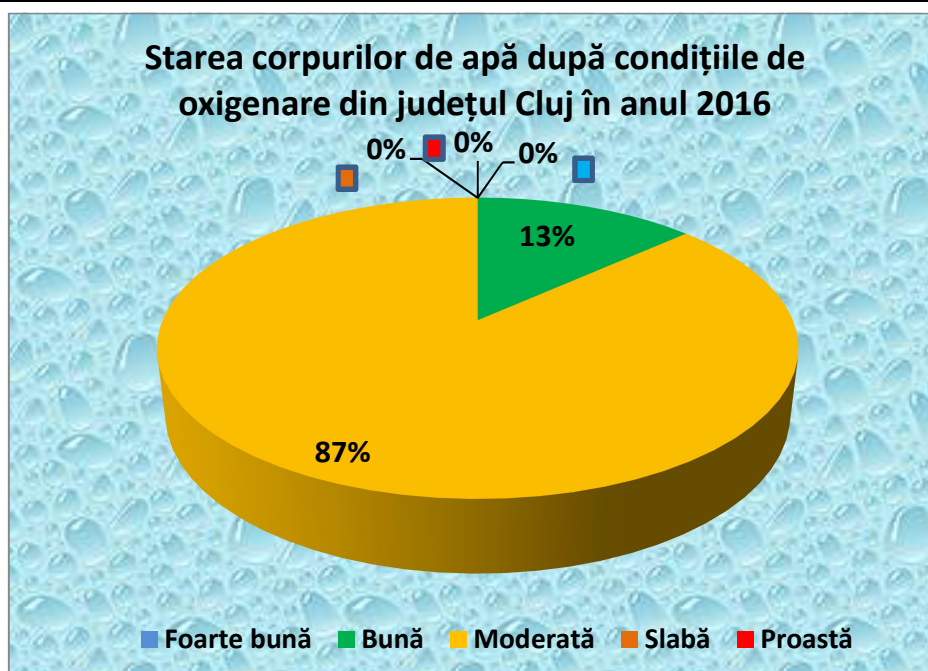
Figura II.2.1.1.6. Starea corpurilor de apă naturală – râuri după condițiile de oxigenare în județul Cluj în anul 2016
