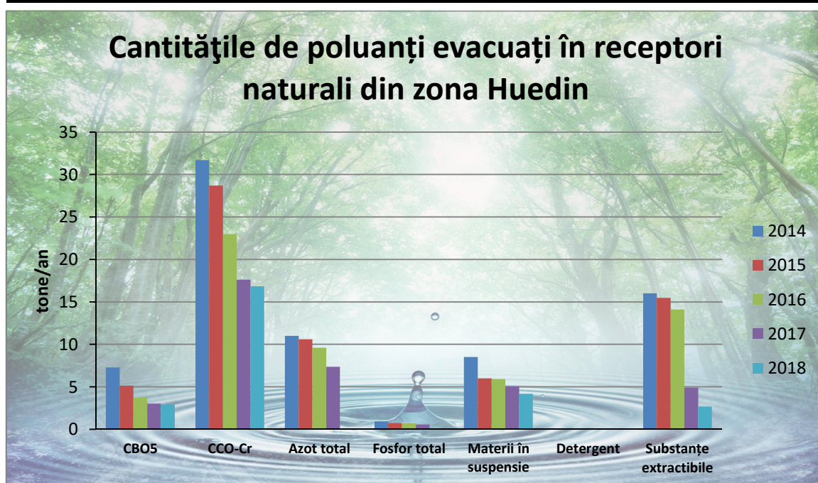
Figura II.2.2.2.6. Cantitățile de poluanți evacuați în receptori naturali din zona Huedin, în perioada 2014-2018
