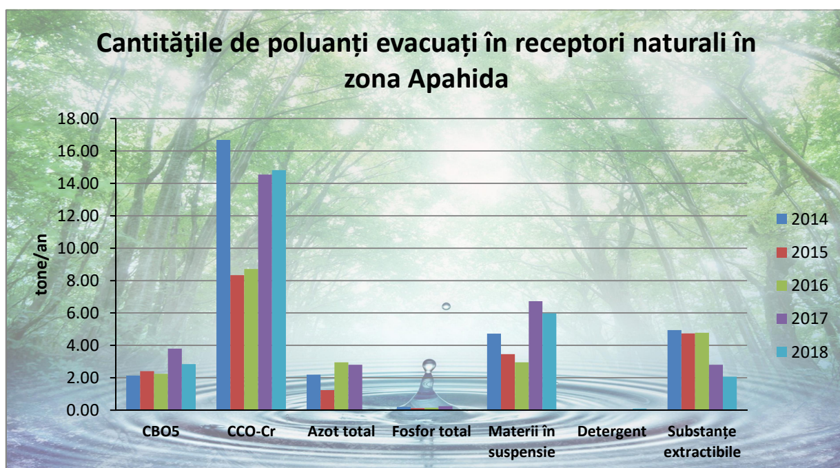
Figura II.2.2.2.3. Cantitățile de poluanți evacuați în receptori naturali în zona Apahida, în perioada 2014-2018
