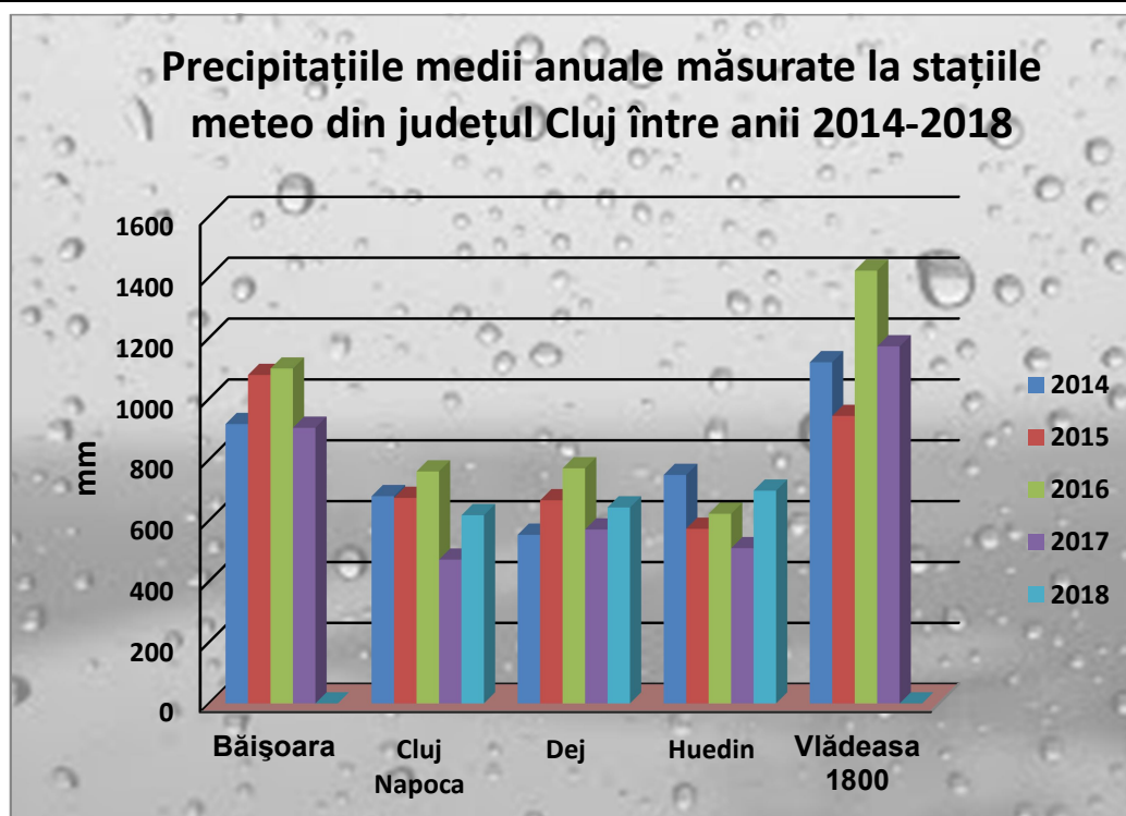
Figura II.1.2.2.3. Evoluția cantităților medii de precipitații măsurate la stațiile meteo din județul Cluj în perioada 2014 – 2018.
