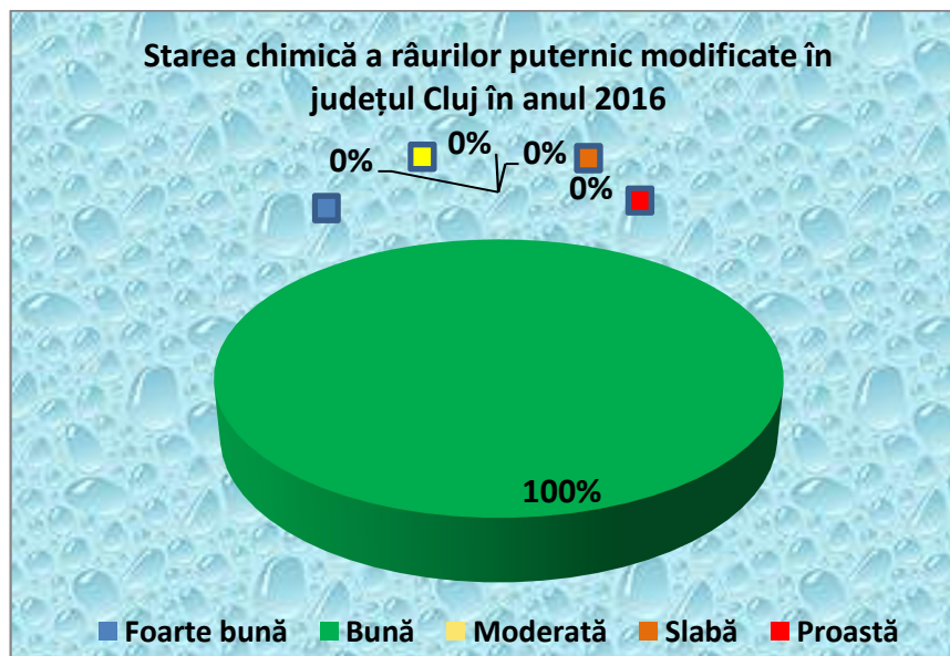
Figura II.2.1.1.4. Starea chimică a râurilor puternic modificate din Bazinul Hidrografic Someș-Tisa la nivelul județului Cluj în anul 2016 ) 5
