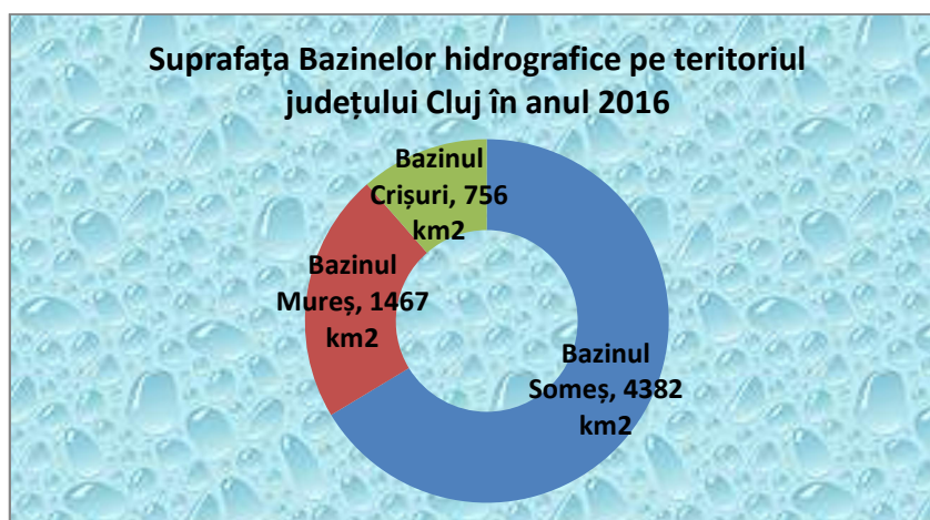
Figura II.1.1.1. Suprafața Bazinelor hidrografice pe teritoriul județului Cluj în anul 2016.
