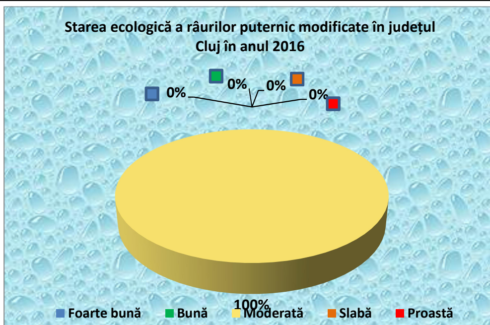
Figura II.2.1.1.3. – Starea ecologică a râurilor puternic modificate din Bazinul Hidrografic Someș-Tisa la nivelul județului Cluj în anul 2016 ) 4
