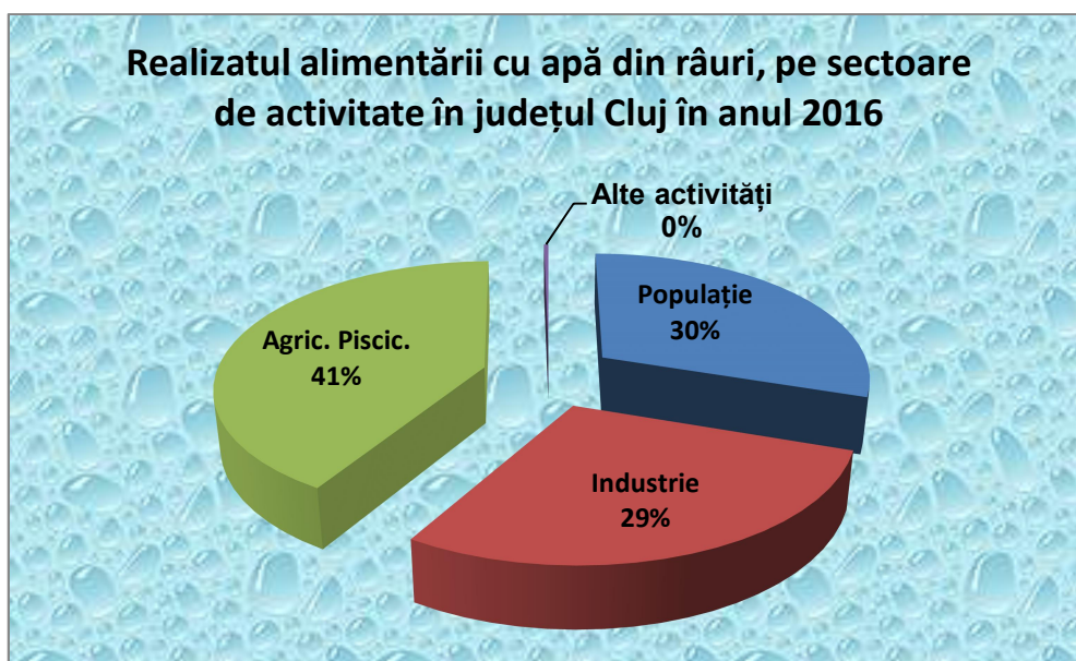
Figura II.1.1.2.7. Realizatul alimentării cu apă din râuri în județul Cluj în anul 2016
