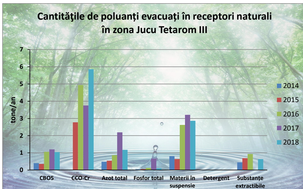
Figura II.2.2.2.8. Cantitățile de poluanți evacuați în receptori naturali în zona Jucu Tetarom III, în perioada 2014-2018
