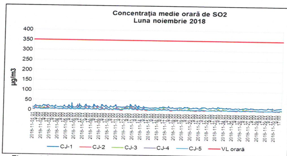
Figura 1.2.1.2. Evoluția mediilor orare de SO 2 în luna noiembrie 2018
