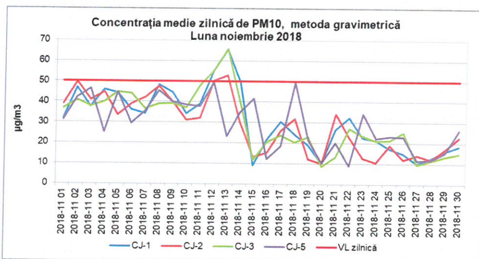
Figura 1.2.5.1. Evoluția mediilor zilnice de PM 10 , în luna noiembrie 2018
