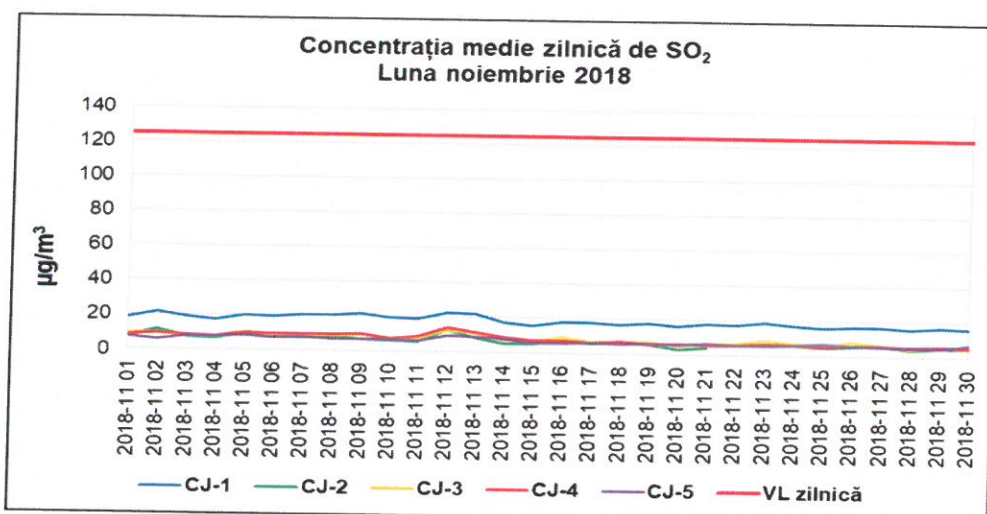
Figura 1.2.1.1. Evoluția mediilor zilnice de SO 2 în luna noiembrie 2018
