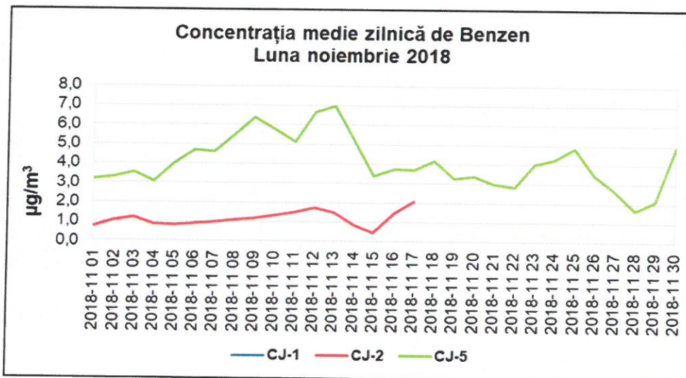
Figura 1.2.7.1. Evoluția mediilor zilnice de benzen, în luna noiembrie 2018
