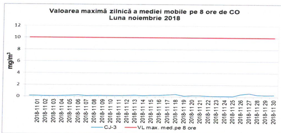
Figura 1.2.4.1. Evoluția maximelor zilnice ale mediilor mobile pe 8 ore de CO, în luna noiembrie 2018
