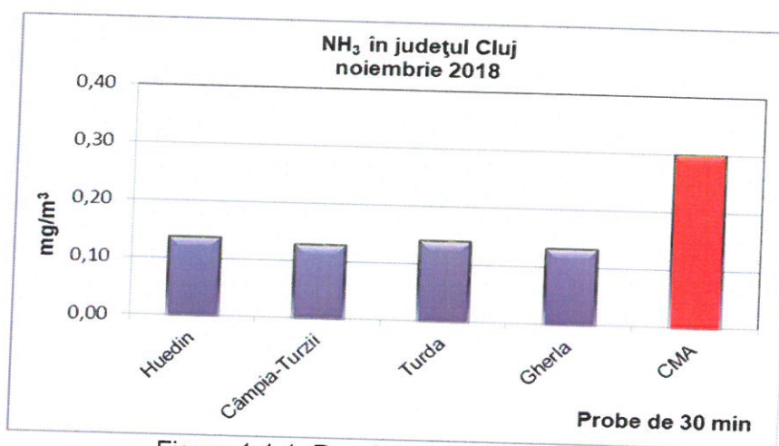
Figura 1.1.1. Rezultatele monitorizării amoniacului
