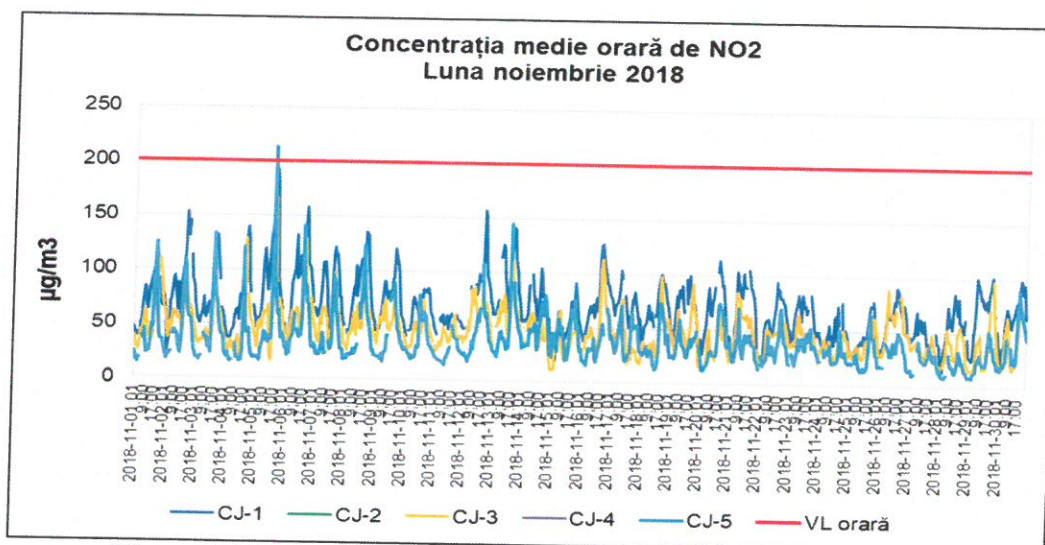
Figura 1.2.2.1. Evoluția mediilor orare de NO 2 în luna noiembrie 2018
