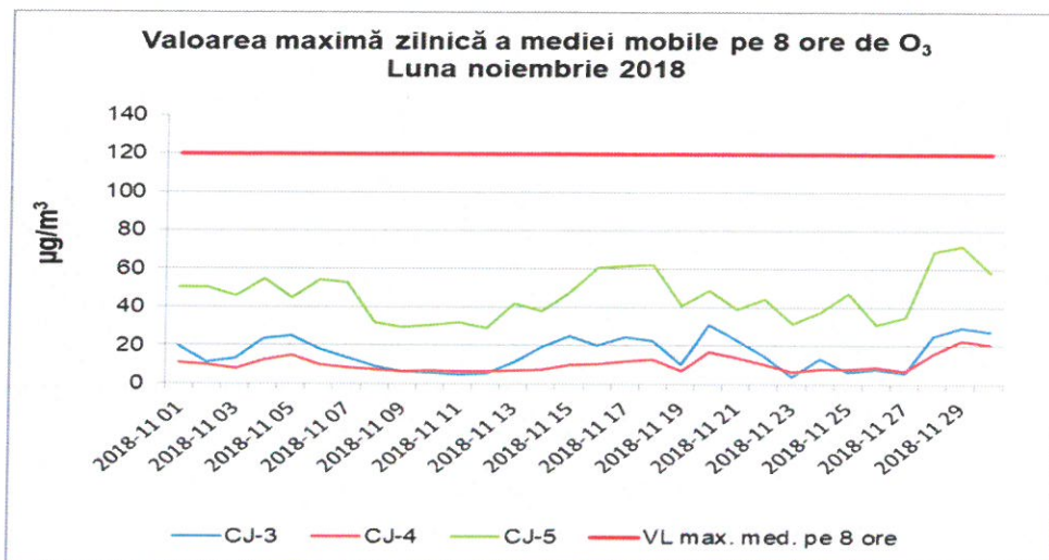
Figura 1.2.3.1. Evoluția maximelor zilnice ale mediilor mobile pe 8 ore de \text{O}_3 , în luna noiembrie 2018
