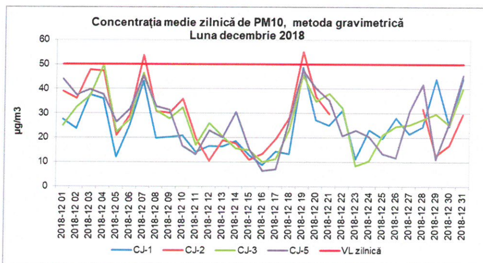
Figura 1.2.5.1. Evoluția mediilor zilnice de PM 10 , în luna decembrie 2018
