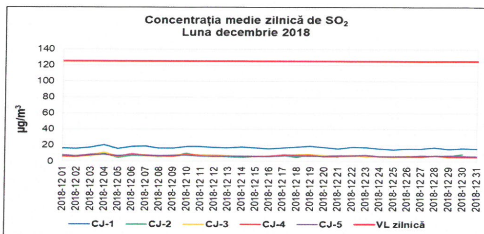
Figura 1.2.1.1. Evoluția mediilor zilnice de SO 2 în luna decembrie 2018
