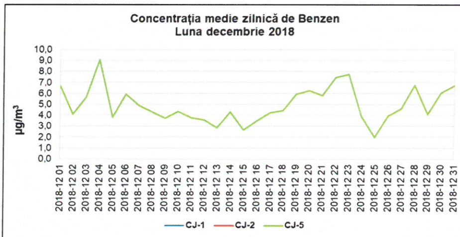
Figura 1.2.7.1. Evoluția mediilor zilnice de benzen, în luna decembrie 2018
