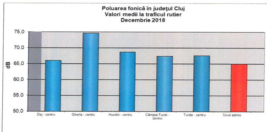
Figura 4.2. Rezultatele monitorizării nivelului de zgomot în județul Cluj
