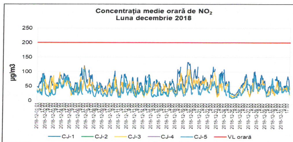
Figura 1.2.2.1. Evoluția mediilor orare de NO 2 în luna decembrie 2018
