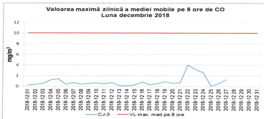
Figura 1.2.4.1. Evoluția maximelor zilnice ale mediilor mobile pe 8 ore de CO, în luna decembrie 2018
