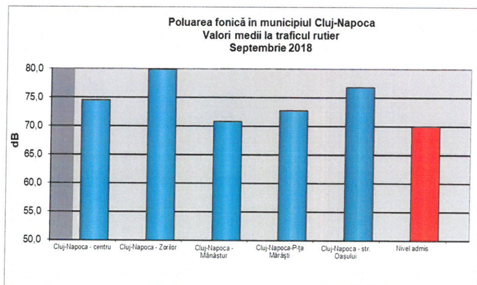
Figura 4.1. Rezultatele monitorizării nivelului de zgomot în Cluj-Napoca
