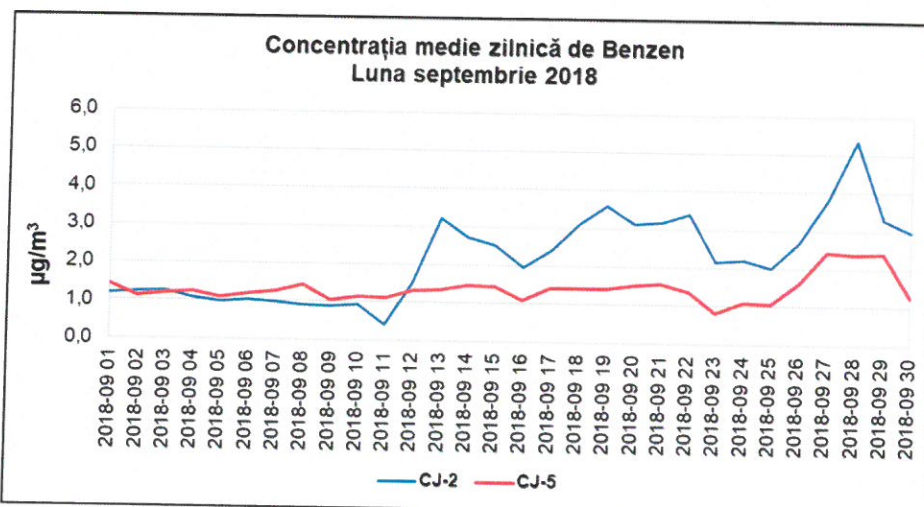
Figura 1.2.7.1. Evoluția mediilor zilnice de benzen, în luna septembrie 2018
