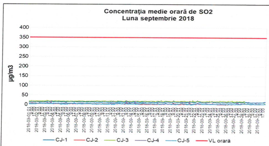
Figura 1.2.1.2. Evoluția mediilor orare de SO 2 în luna septembrie 2018
