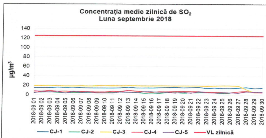
Figura 1.2.1.1. Evoluția mediilor zilnice de SO 2 în luna septembrie 2018
