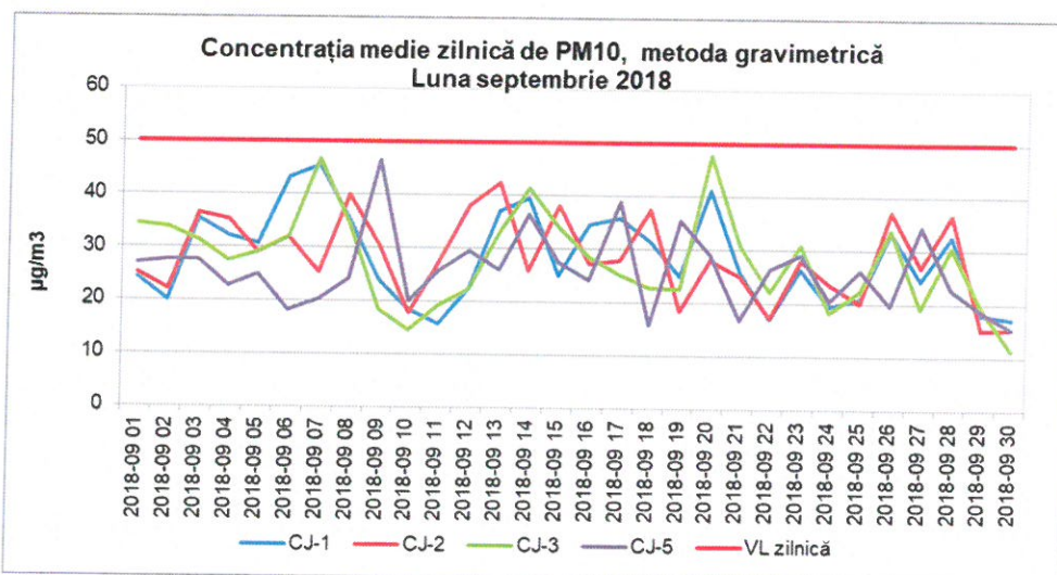
Figura 1.2.5.1. Evoluția mediilor zilnice de PM 10 , în luna septembrie 2018
