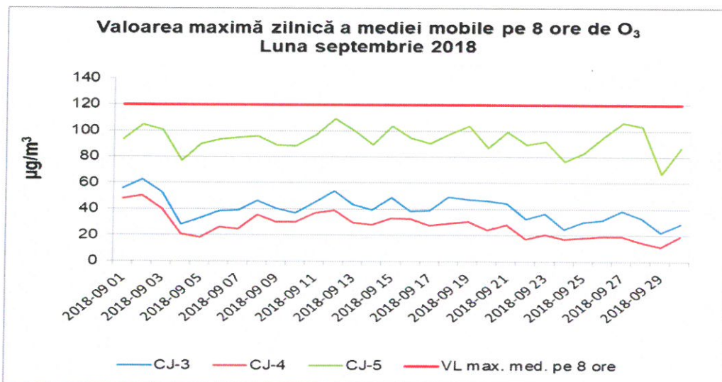
Figura 1.2.3.1. Evoluția maximelor zilnice ale mediilor mobile pe 8 ore de \text{O}_3 , în luna septembrie 2018
