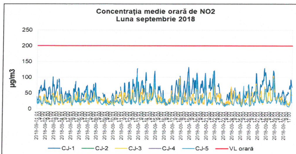
Figura 1.2.2.1. Evoluția mediilor orare de NO 2 în luna septembrie 2018
