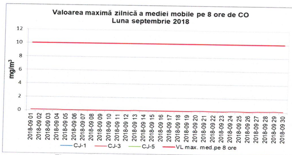
Figura 1.2.4.1. Evoluția maximelor zilnice ale mediilor mobile pe 8 ore de CO, în luna septembrie 2018
