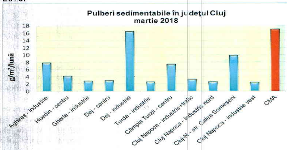
Figura 1.1.4. Rezultatele monitorizării pulberilor sedimentabile
