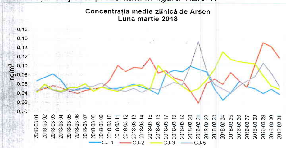
Figura 1.2.6.1. Evoluția mediilor zilnice de As, în luna martie 2018
