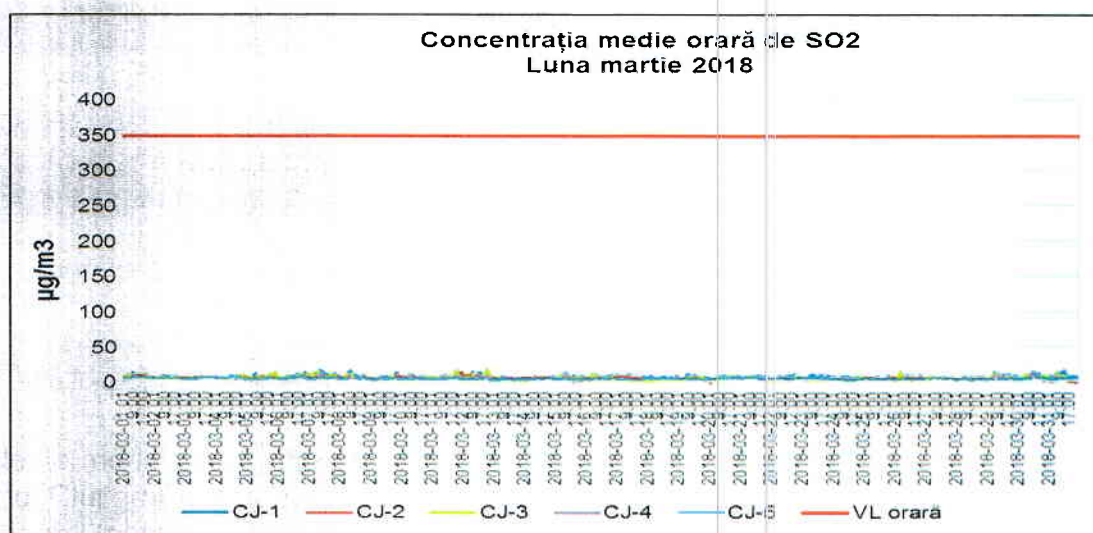
Figura 1.2.1.1. Evoluția mediilor orare de SO 2 în luna martie 2018
