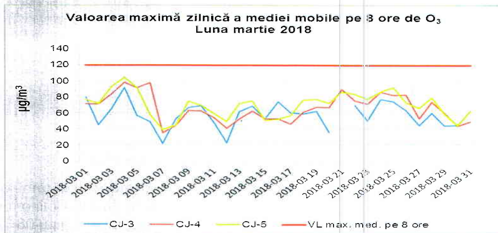
Figura 1.2.3.1. Evoluția maximelor zilnice ale mediilor mobile pe 8 ore de \text{O}_3 , în luna martie 2018
