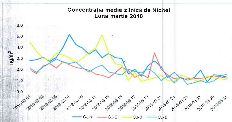
Figura 1.2.6.3. Evoluția mediilor zilnice de Ni, în luna martie 2018
