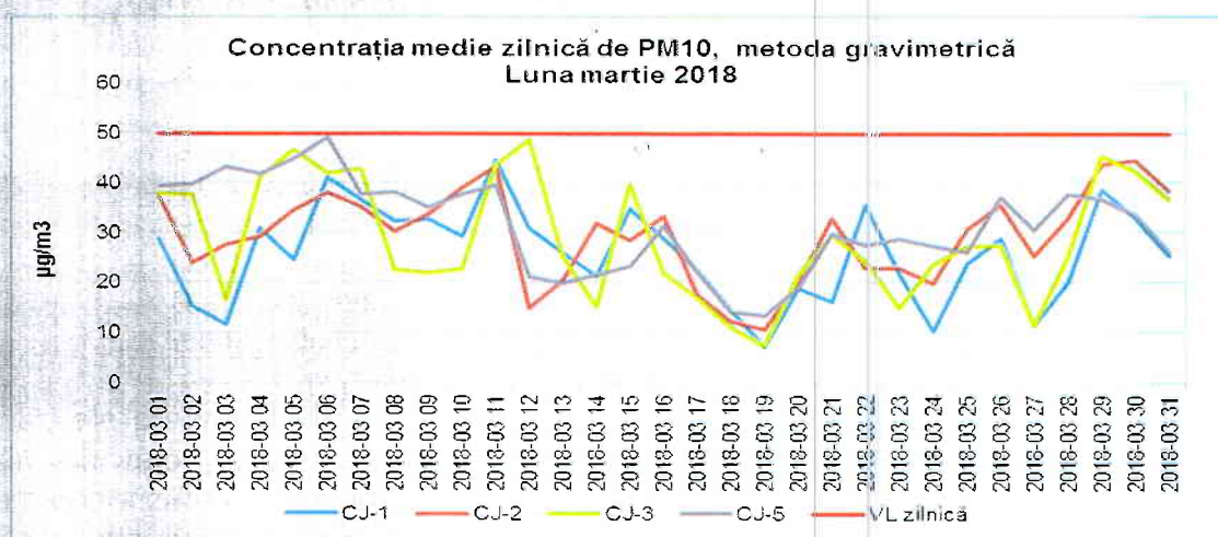
Figura 1.2.5.1. Evoluția mediilor zilnice de PM 10 , în luna martie 2018
