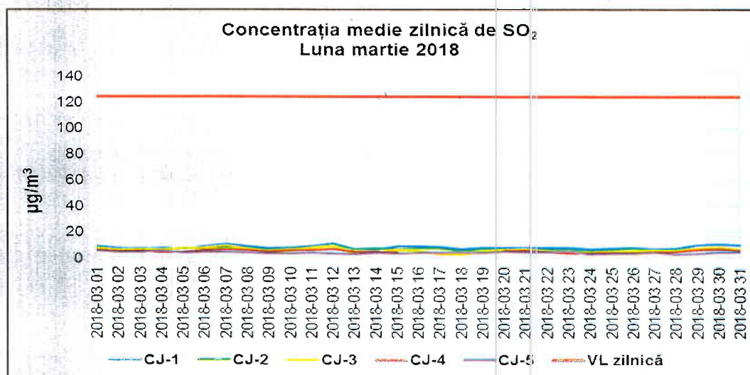
Figura 1.2.1.1. Evoluția mediilor zilnice de SO 2 în luna martie 2018
