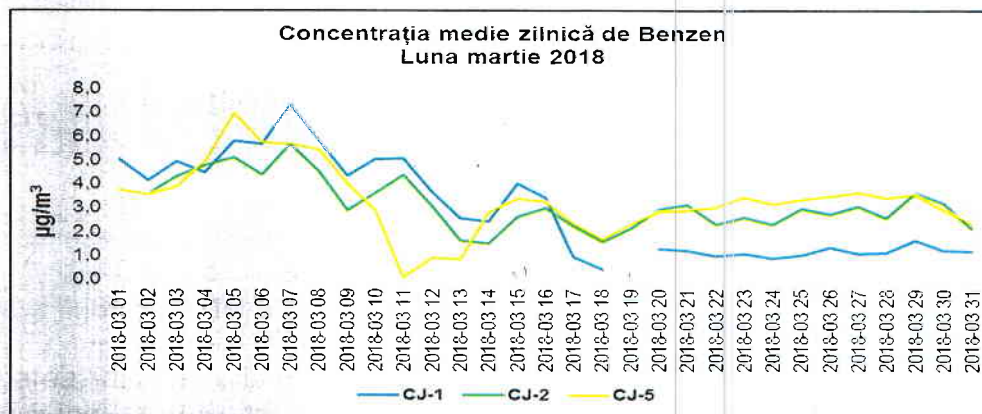
Figura 1.2.7.1. Evoluția mediilor zilnice de benzen, în luna martie 2018
