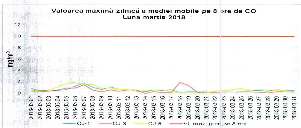
Figura 1.2.4.1. Evoluția maximelor zilnice ale mediilor mobile pe 8 ore de CO, în luna martie 2018
