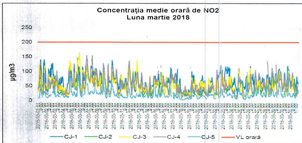
Figura 1.2.2.1. Evoluția mediilor orare de NO 2 în luna martie 2018
