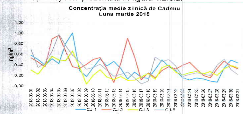
Figura 1.2.6.2. Evoluția mediilor zilnice de Cd, în luna martie 2018
