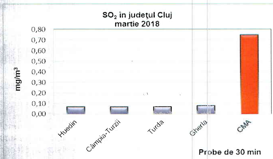
Figura 1.1.3. Rezultatele monitorizării dioxidului de sulf
