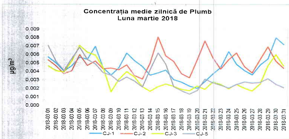
Figura 1.2.6.4. Evoluția mediilor zilnice de Pb, în luna martie 2018
