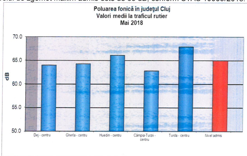
Figura 4.1. Rezultatele monitorizării nivelului de zgomot în județul Cluj
