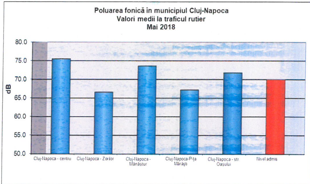
Figura 4.1. Rezultatele monitorizării nivelului de zgomot în Cluj-Napoca
