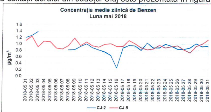
Figura 1.2.7.1. Evoluția mediilor zilnice de benzen, în luna mai 2018
