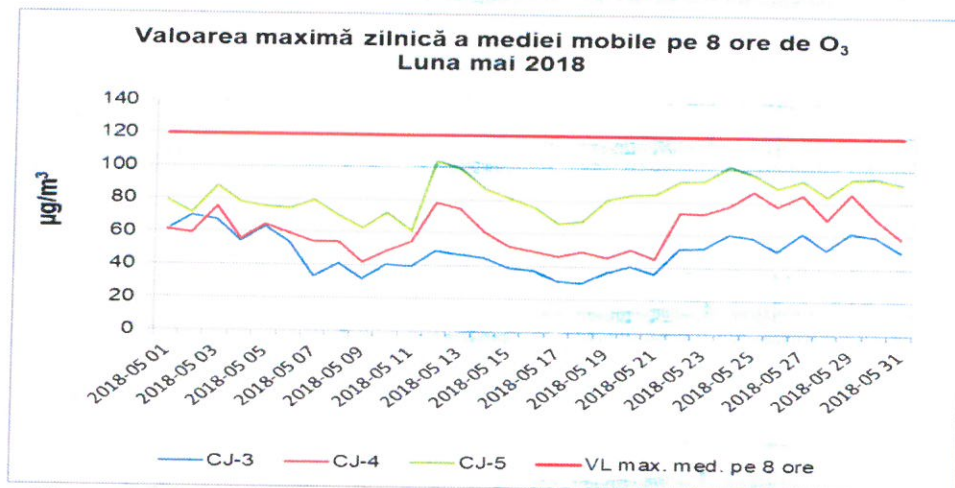
Figura 1.2.3.1. Evoluția maximelor zilnice ale mediilor mobile pe 8 ore de \text{O}_3 , în luna mai 2018
