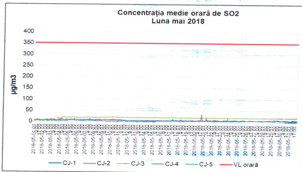
Figura 1.2.1.1. Evoluția mediilor orare de SO 2 în luna mai 2018
