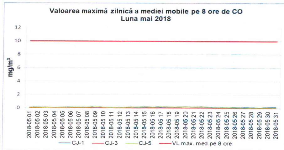
Figura 1.2.4.1. Evoluția maximelor zilnice ale mediilor mobile pe 8 ore de CO, în luna mai 2018
