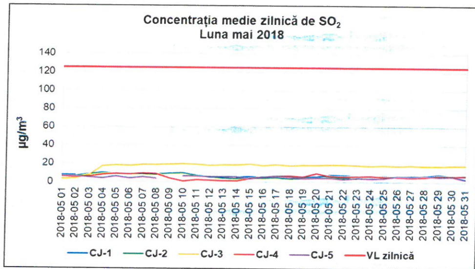
Figura 1.2.1.1. Evoluția mediilor zilnice de SO 2 în luna mai 2018
