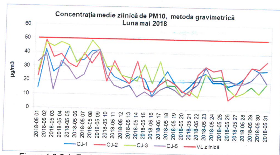
Figura 1.2.5.1. Evoluția mediilor zilnice de PM 10 , în luna mai 2018
