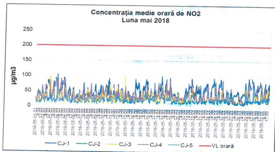
Figura 1.2.2.1. Evoluția mediilor orare de NO 2 în luna mai 2018
