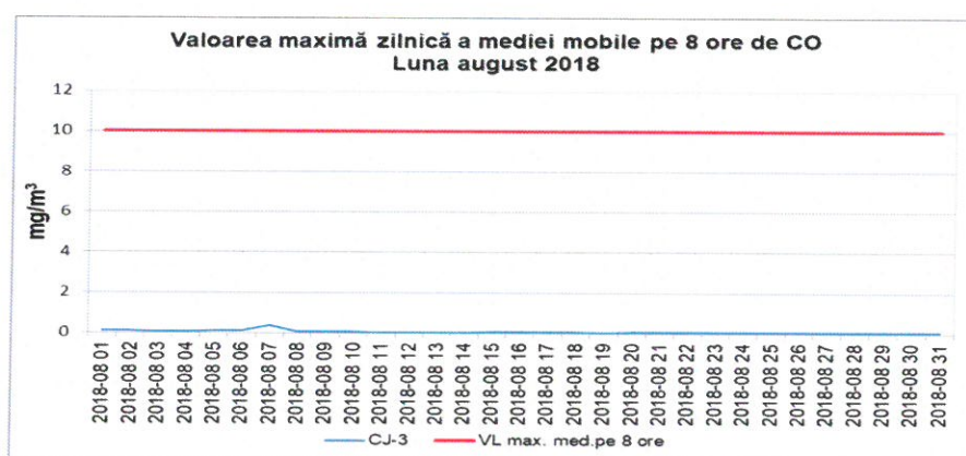
Figura 1.2.4.1. Evoluția maximelor zilnice ale mediilor mobile pe 8 ore de CO, în luna august 2018
