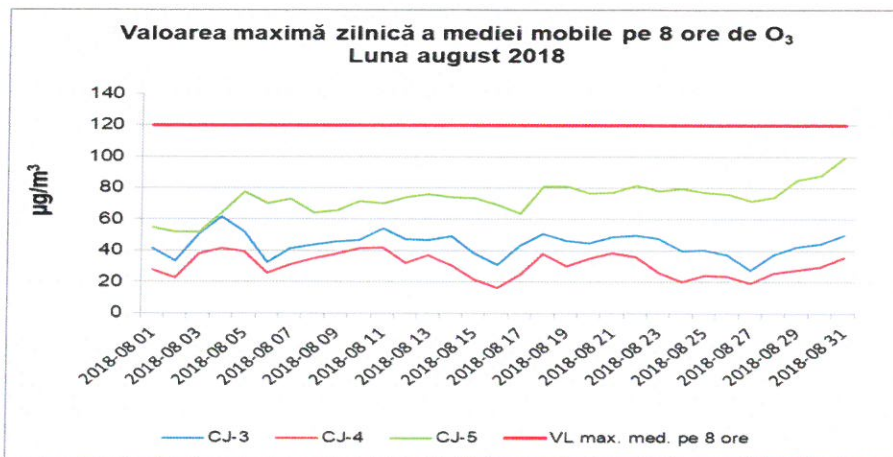
Figura 1.2.3.1. Evoluția maximelor zilnice ale mediilor mobile pe 8 ore de \text{O}_3 , în luna august 2018
