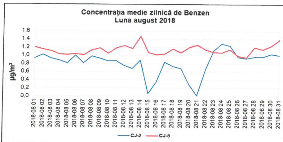
Figura 1.2.7.1. Evoluția mediilor zilnice de benzen, în luna august 2018
