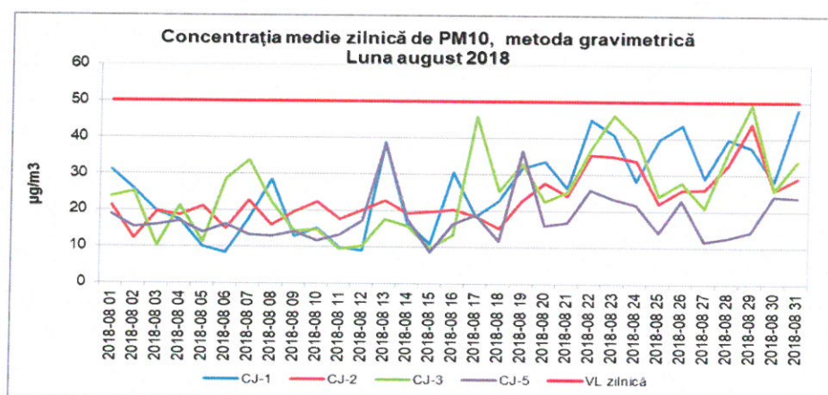
Figura 1.2.5.1. Evoluția mediilor zilnice de PM 10 , în luna august 2018
