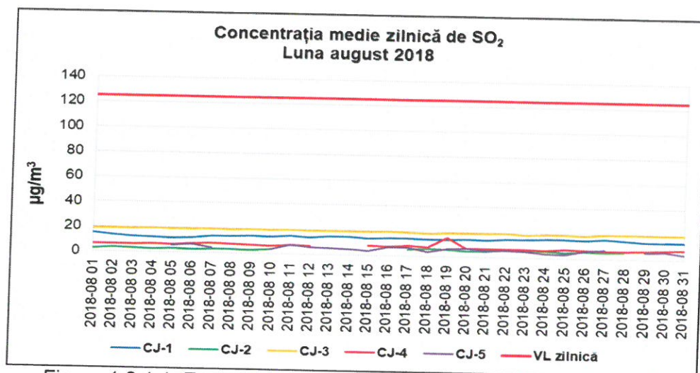
Figura 1.2.1.1. Evoluția mediilor zilnice de SO 2 în luna august 2018
