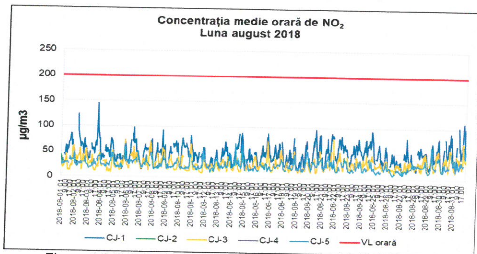
Figura 1.2.2.1. Evoluția mediilor orare de NO 2 în luna august 2018
