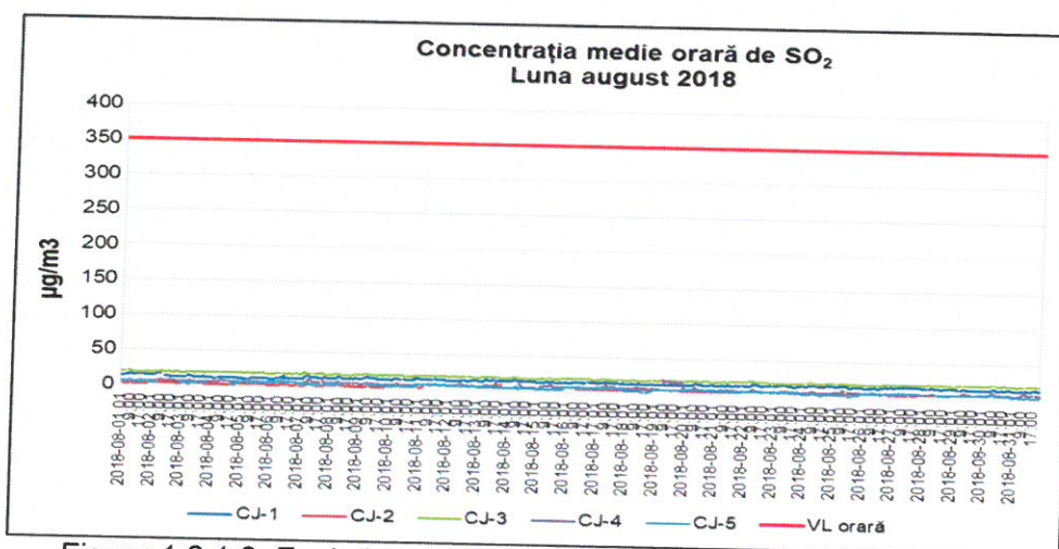
Figura 1.2.1.2. Evoluția mediilor orare de SO 2 în luna august 2018
