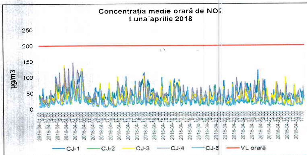
Figura 1.2.2.1. Evoluția mediilor orare de NO 2 în luna aprilie 2018
