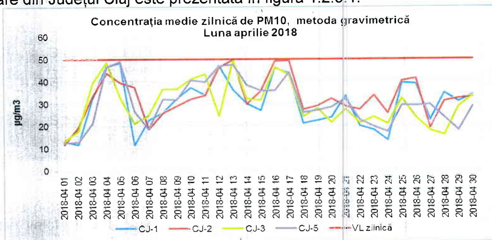
Figura 1.2.5.1. Evoluția mediilor zilnice de PM 10 , în luna aprilie 2018
