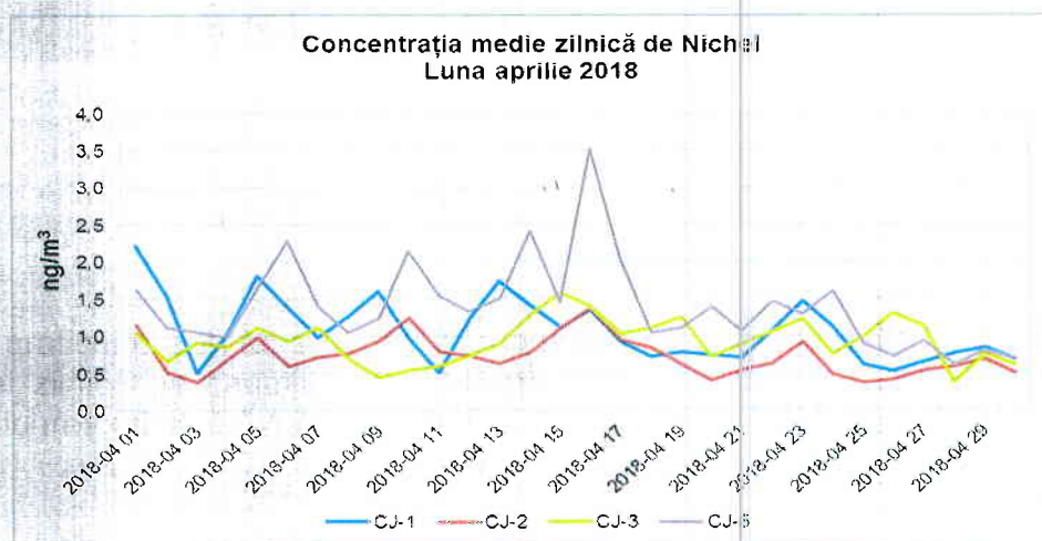
Figura 1.2.6.3. Evoluția mediilor zilnice de Ni, în luna aprilie 2018
