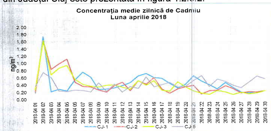
Figura 1.2.6.2. Evoluția mediilor zilnice de Cd, în luna aprilie 2018
