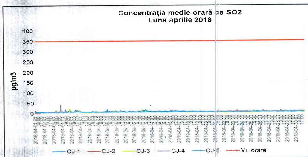
Figura 1.2.1.1. Evoluția mediilor orare de SO 2 în luna aprilie 2018
