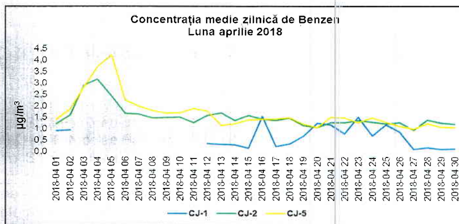
Figura 1.2.7.1. Evoluția mediilor zilnice de benzen în luna aprilie 2018
