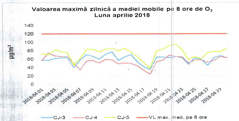
Figura 1.2.3.1. Evoluția maximelor zilnice ale mediilor mobile pe 8 ore de \text{O}_3 , în luna aprilie 2018
