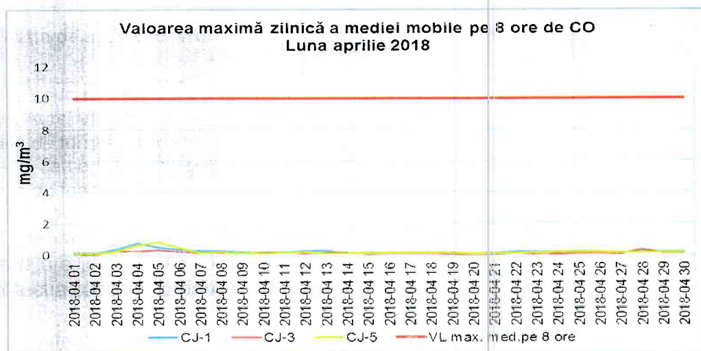
Figura 1.2.4.1. Evoluția maximelor zilnice ale mediilor mobile pe 8 ore de CO, în luna aprilie 2018
