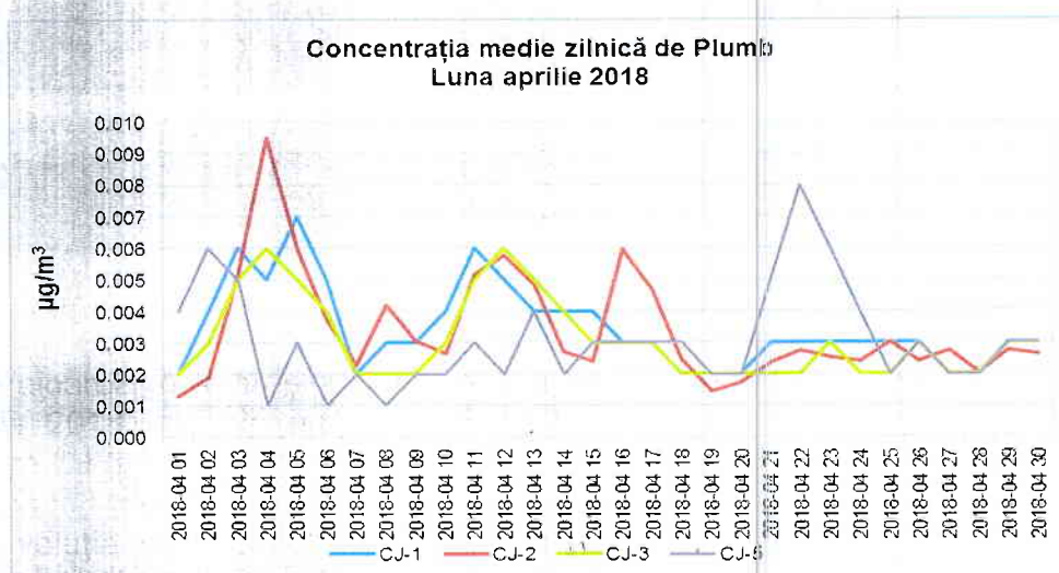
Figura 1.2.6.4. Evoluția mediilor zilnice de Pb, în luna aprilie 2018
