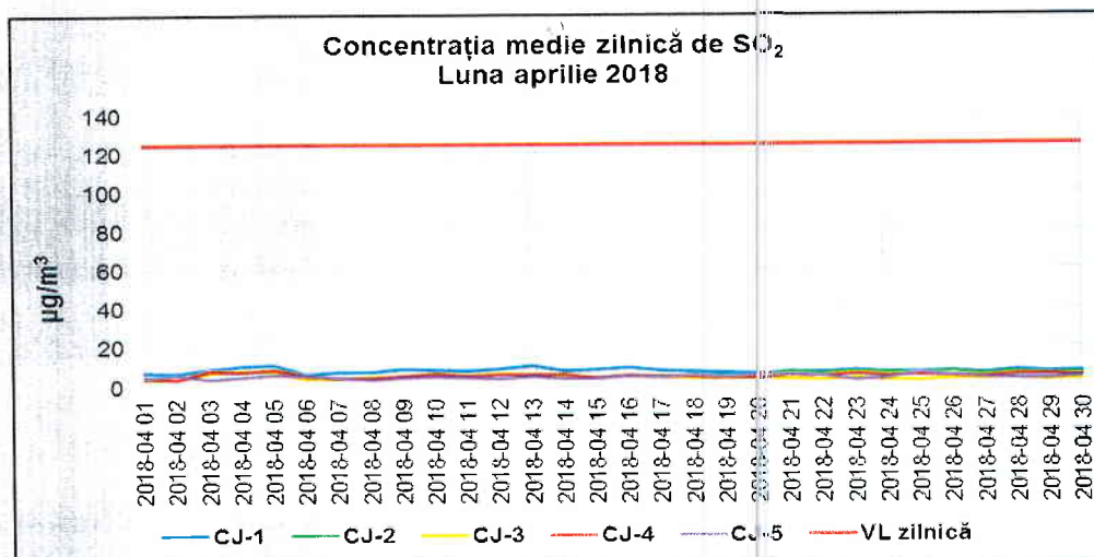
Figura 1.2.1.1. Evoluția mediilor zilnice de SO 2 în luna aprilie 2018
