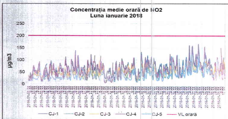
Figura 1.2.2.1. Evoluția mediilor orare de NO 2 în luna ianuarie 2018
