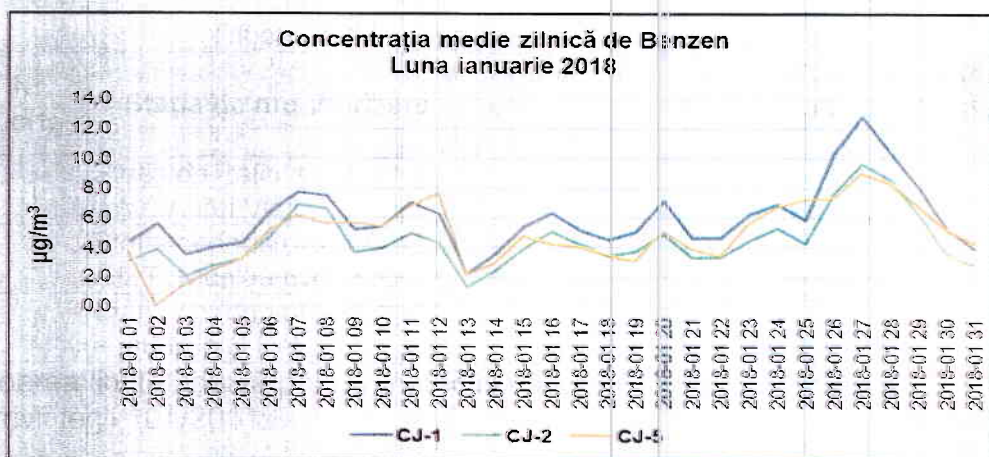
Figura 1.2.7.1. Evoluția mediilor zilnice de benzen, în luna ianuarie 2018
