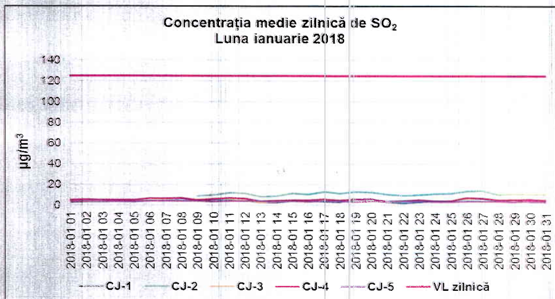
Figura 1.2.1.1. Evoluția mediilor zilnice de SO 2 în luna ianuarie 2018
