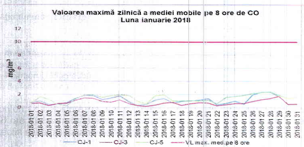
Figura 1.2.4.1. Evoluția maximelor zilnice ale mediilor mobile pe 8 ore de CO, în luna ianuarie 2018
