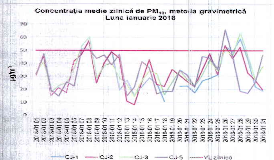
Figura 1.2.5.1. Evoluția mediilor zilnice de PM 10 , în luna ianuarie 2018
