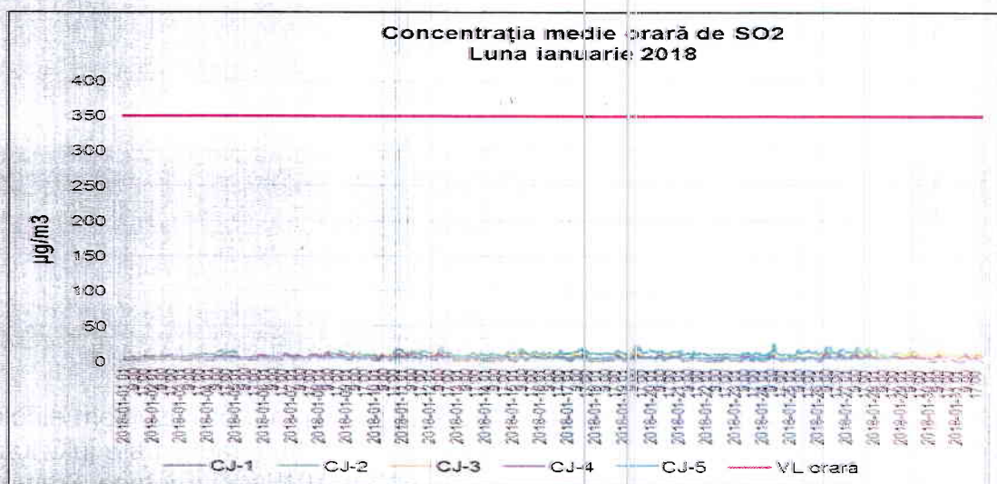
Figura 1.2.1.1. Evoluția mediilor orare de SO 2 în luna ianuarie 2018
