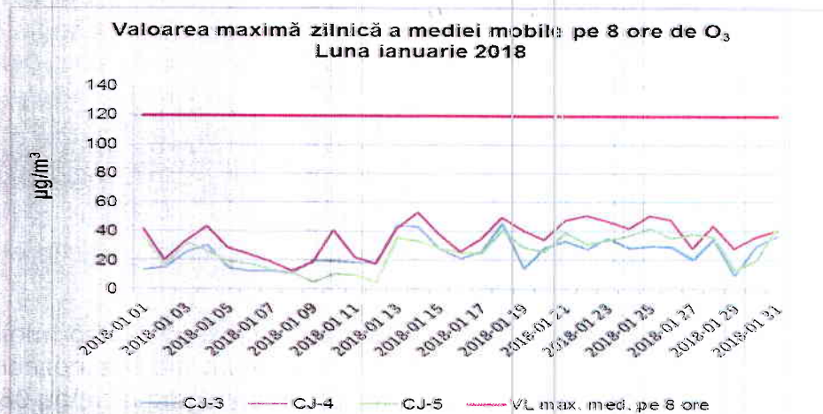
Figura 1.2.3.1. Evoluția maximelor zilnice ale mediilor mobile pe 8 ore de \text{O}_3 , în luna ianuarie 2018
