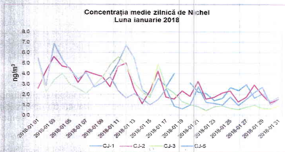
Figura 1.2.6.3. Evoluția mediilor zilnice de Ni, în luna ianuarie 2018
