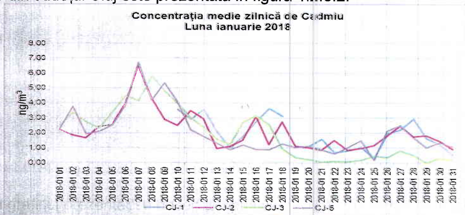
Figura 1.2.6.2. Evoluția mediilor zilnice de Cd în luna ianuarie 2018
