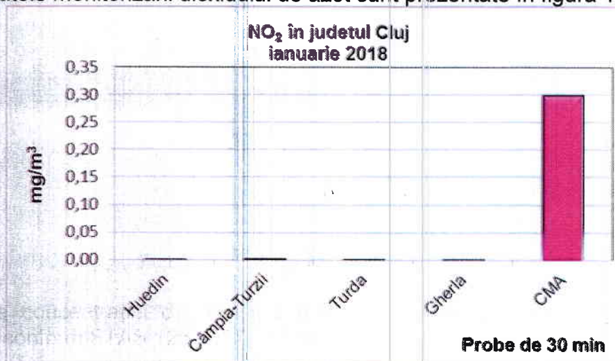
Figura 1.1.2. Rezultatele monitorizării dioxidului de azot
