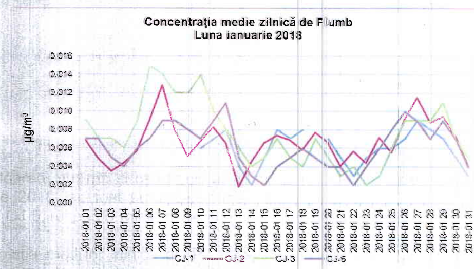
Figura 1.2.6.4. Evoluția mediilor zilnice de Pb, în luna ianuarie 2018
