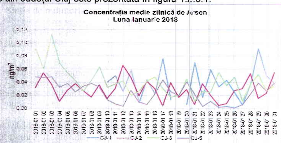
Figura 1.2.6.1. Evoluția mediilor zilnice de As, în luna ianuarie 2018
