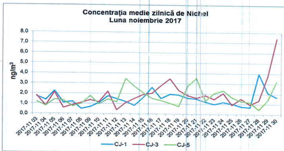
Figura 1.2.6.3. Evoluția mediilor zilnice de Ni, în luna noiembrie 2017
