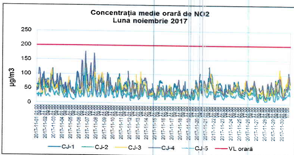
Figura 1.2.2.1. Evoluția mediilor orare de NO 2 în luna noiembrie 2017
