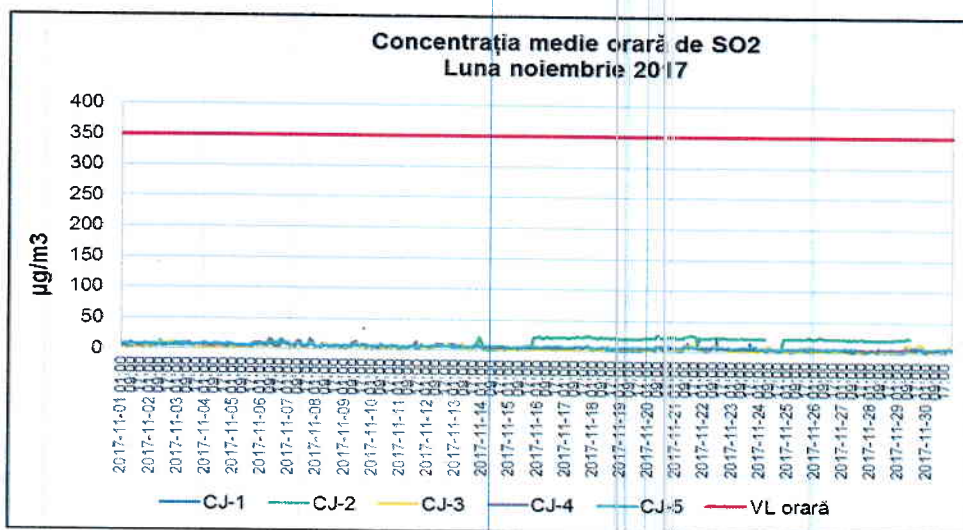
Figura 1.2.1.1. Evoluția mediilor orare de SO 2 în luna noiembrie 2017
