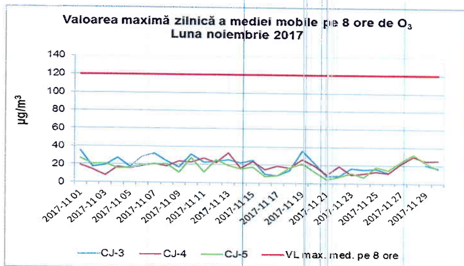
Figura 1.2.3.1. Evoluția maximelor zilnice ale mediilor mobile pe 8 ore de \text{O}_3 , în luna noiembrie 2017
