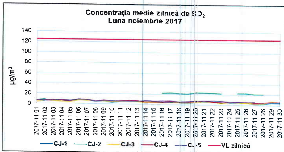
Figura 1.2.1.1. Evoluția mediilor zilnice de SO 2 în luna noiembrie 2017
