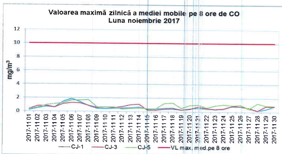
Figura 1.2.4.1. Evoluția maximelor zilnice ale mediilor mobile pe 8 ore de CO, în luna noiembrie 2017
