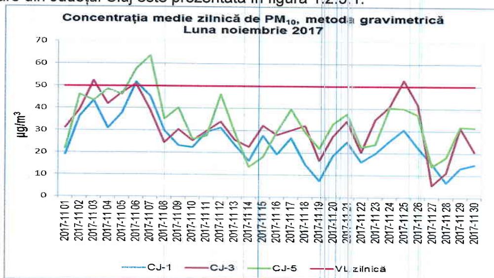
Figura 1.2.5.1. Evoluția mediilor zilnice de PM 10 în luna noiembrie 2017
