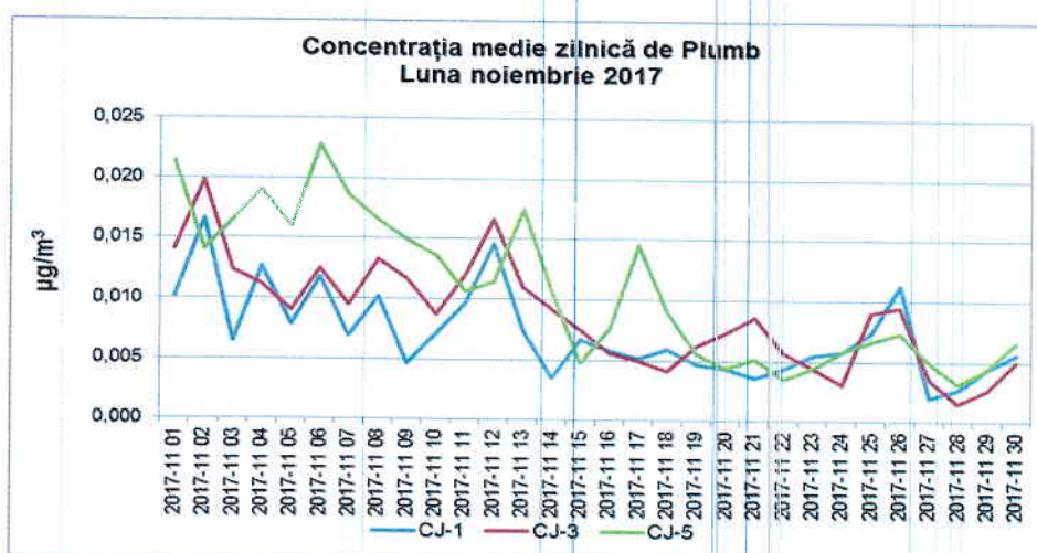
Figura 1.2.6.4. Evoluția mediilor zilnice de Pb, în luna noiembrie 2017
