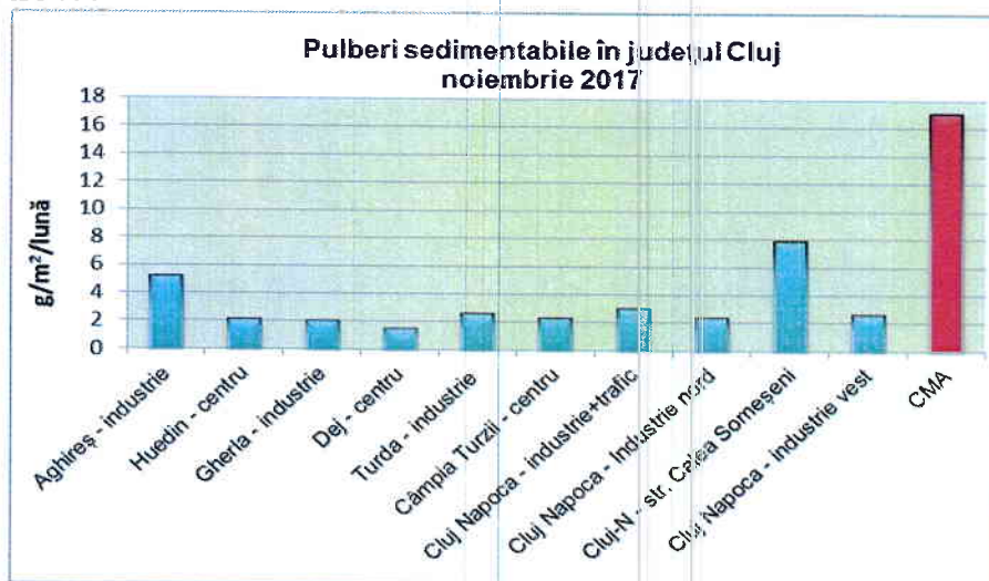
Figura 1.1.4. Rezultatele monitorizării pulberilor sedimentabile
