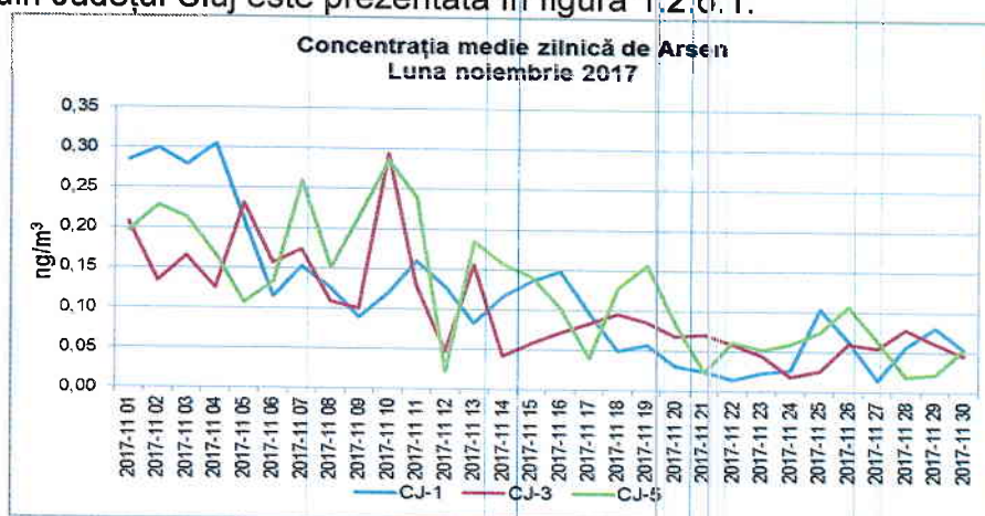
Figura 1.2.6.1. Evoluția mediilor zilnice de As, în luna noiembrie 2017
