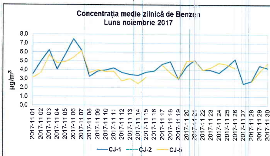
Figura 1.2.7.1. Evoluția mediilor zilnice de benzen, în luna noiembrie 2017
