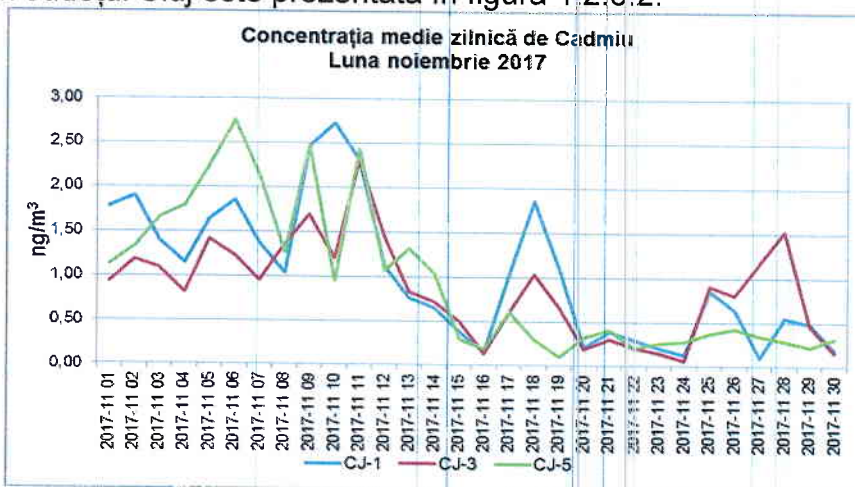
Figura 1.2.6.2. Evoluția mediilor zilnice de Cd, în luna noiembrie 2017
