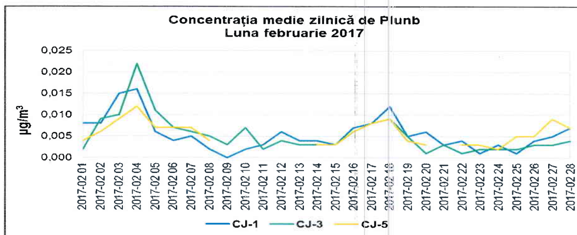
Figura 1.2.6.4. Evoluția mediilor zilnice de Pb, în luna februarie 2017
