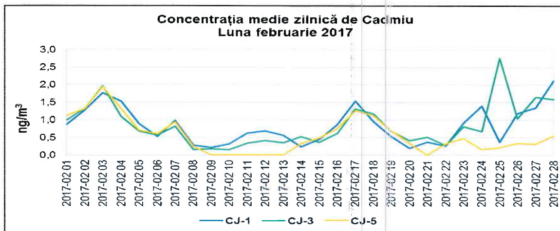
Figura 1.2.6.2. Evoluția mediilor zilnice de Cd, în luna februarie 2017
