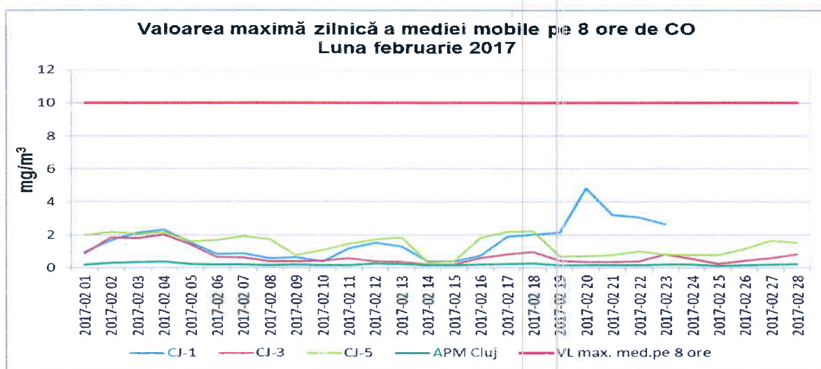
Figura 1.2.4.1. Evoluția maximelor zilnice ale mediilor mobile pe 8 ore de CO, în luna februarie 2017
