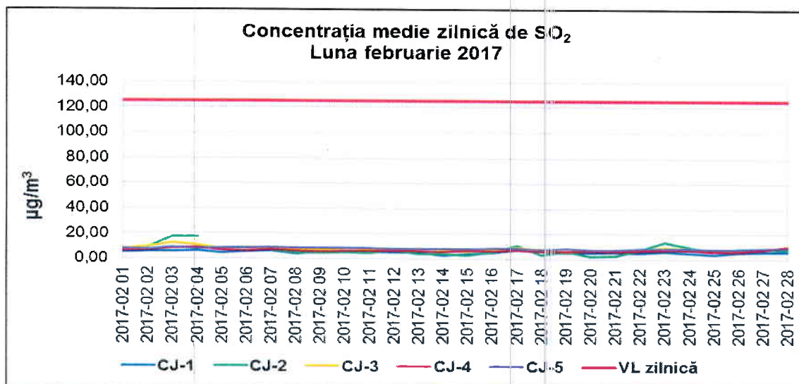
Figura 1.2.1.1. Evoluția mediilor zilnice de SO 2 în luna februarie 2017
