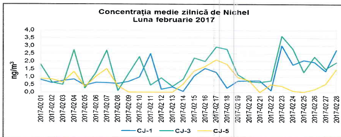
Figura 1.2.6.3. Evoluția mediilor zilnice de Ni, în luna februarie 2017
