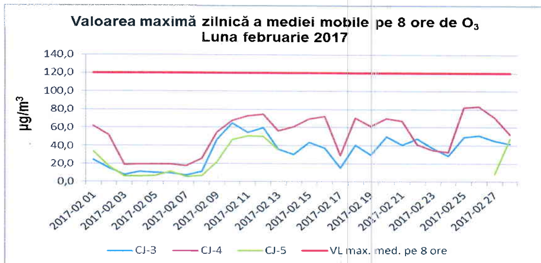
Figura 1.2.3.1. Evoluția maximelor zilnice ale mediilor mobile pe 8 ore de \text{O}_3 , în luna februarie 2017
