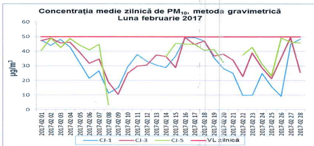
Figura 1.2.5.1. Evoluția mediilor zilnice de PM 10 , în luna februarie 2017
