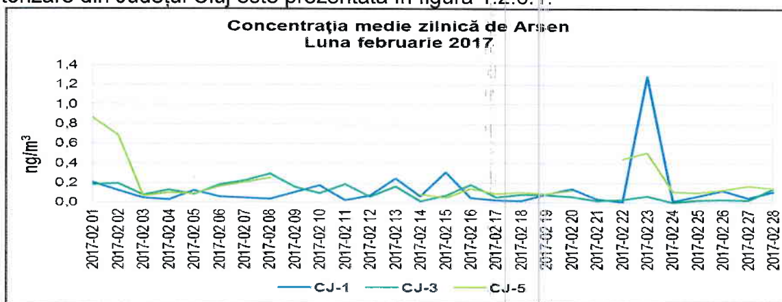
Figura 1.2.6.1. Evoluția mediilor zilnice de As, în luna februarie 2017
