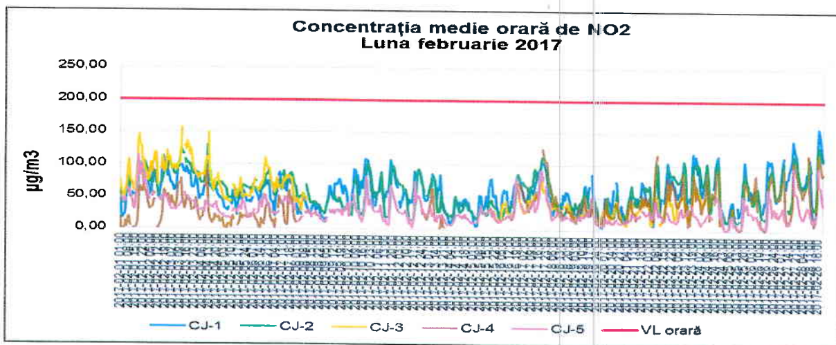
Figura 1.2.2.1. Evoluția mediilor orare de NO 2 în luna februarie 2017
