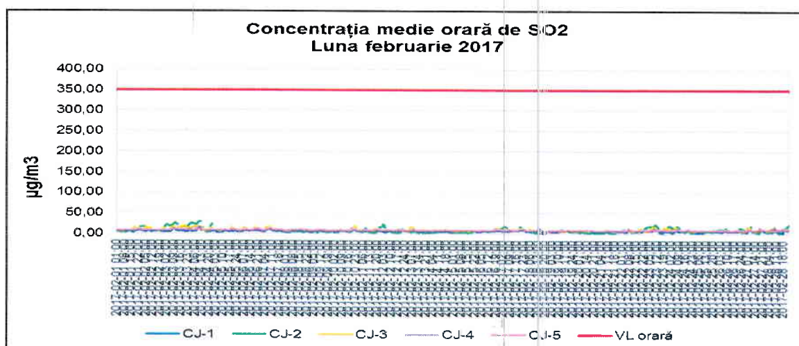
Figura 1.2.1.1. Evoluția mediilor orare de SO 2 în luna februarie 2017
