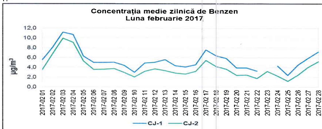
Figura 1.2.7.1. Evoluția mediilor zilnice de benzen, în luna februarie 2017
